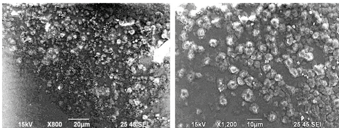
Рисунок 1. Дисперсная фаза воды под трансмиссионным электронным микроскопом JEOL JSM – 6390 LA через сутки после испарения свободной воды со стеклянной поверхности. Слева – множество мелких кристаллов соли (светлые точки) над слоем дисперсной фазы. Справа – кристаллизация хлорида натрия вокруг центральной части единиц дисперсной фазы («темной точки»)
