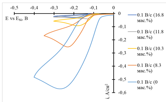
Катодные области вольтамперограмм, полученных на стеклоуглероде в расплавах LiCl-KCl-CsCl с разным содержанием LiCl при 630 °С
