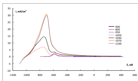
Рисунок 1. Анодные поляризационные кривые в 2М NaOH
