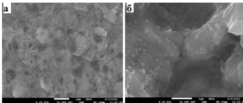
Электронно-микроскопические изображения гальванотермического покрытия: а – до выдержки в 1 М HCl; б – после выдержки в 1 М HCl
