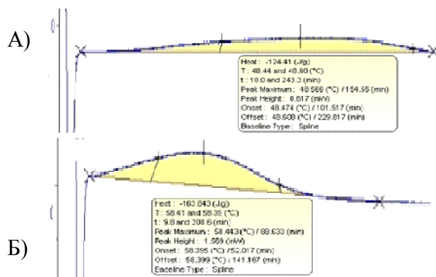
Термограмма отверждения эпоксидной смолы при термостатировании при 50 °С (А) и 60 °С (Б)
