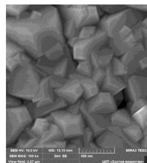
Электронно-микроскопические изображения пленок CdPbS
