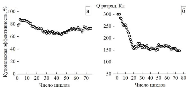
Зависимость кулоновской эффективности от числа циклов заряда/разряда (а); Зависимость электрического заряда разряда от числа циклов заряда/разряда (б)
