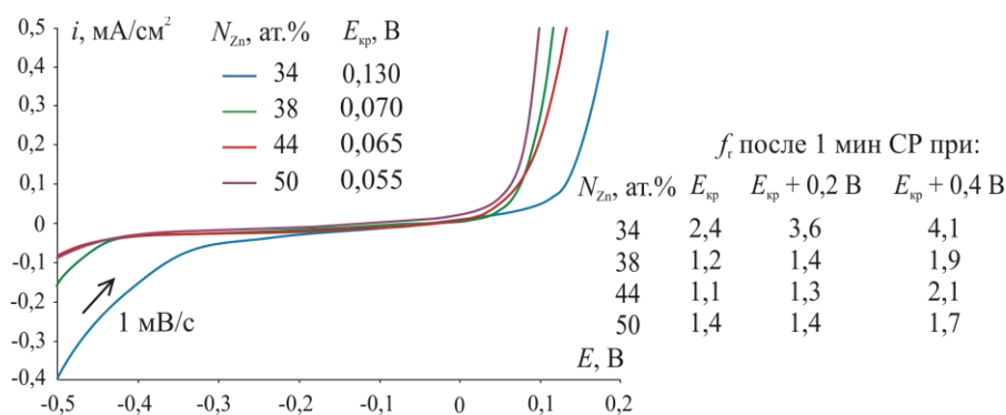
Вольтамперограммы Cu,Zn-сплавов в 0,09 М KCl + 0,01 М HCl
