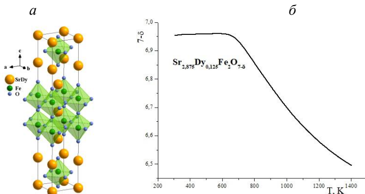
Данные для \text{Sr}_{2.875}\text{Dy}_{0.125}\text{Fe}_2\text{O}_7 : а – структурная модель с выделенным окружением для атома Fe (4e); б – зависимости изменения содержания кислорода от температуры на воздухе
