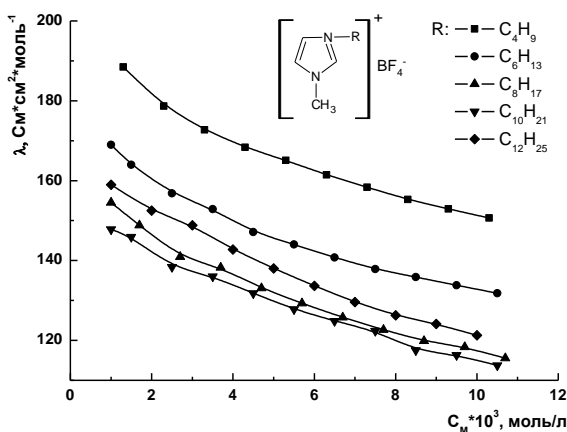
Зависимости эквивалентной ЭП растворов тетрафторборатов 1-алкил-3-метилимидазолия в ацетонитриле от концентрации при 25 °С
