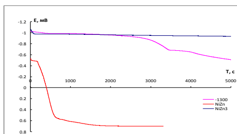
Рисунок 2. Хронопотенциограмма на покрытиях в растворе 2М NaOH
