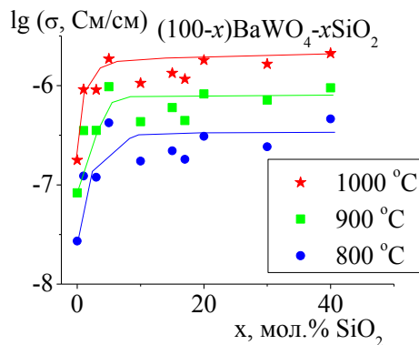
Концентрационная зависимость электропроводности композитов (100-x)\text{BaWO}_4-x\text{SiO}_2
