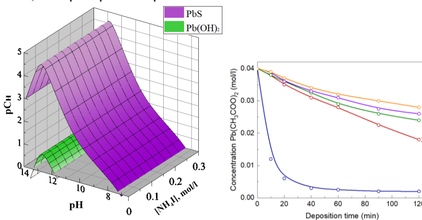
Граничные условия образования труднорастворимых фаз PbS, Pb(OH) 2 (слева) и кинетические кривые превращения соли свинца в PbS в присутствии NH 4 I, моль/л: 0 (1), 0.1 (2), 0.15 (3) 0.2 (4), 0.3 (5) (справа)
