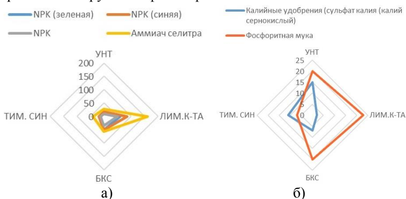
ВО РГФ над азотсодержащими (а) и неазотными (б) удобрениями
