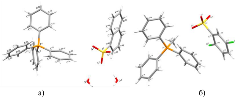
а) Строение 1-нафталинсульфоната тетрафенилфосфония ( 1 );
