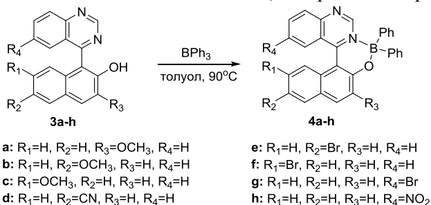
Схема 2 – Синтез N,B,O – комплексов, содержащих хиназолин
