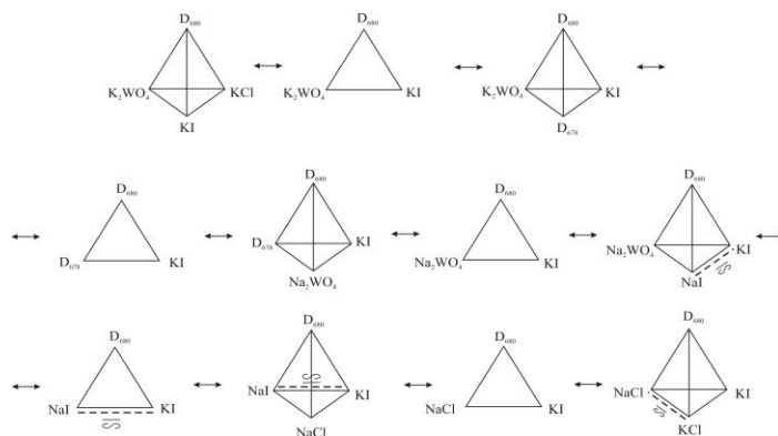
Рисунок 2 – Древо фаз четырехкомпонентной взаимной системы \text{Na,K}||\text{Cl,I,WO}_4
