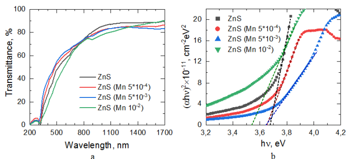
Светопропускание (а) и графическое определение оптической ширины запрещенной зоны (b) пленок ZnS:Mn
