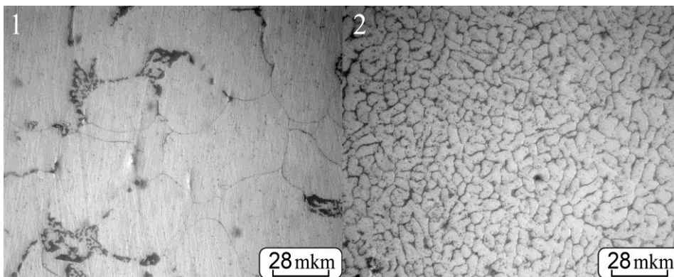
Микрофотография сплава АК6 охлаждённого при обычной скорости (1) и при 1000 К/с (2)
