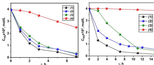
Фотоокисление ГХ на \text{La}_x\text{Sr}_{2-x}\text{Ti}_{1-x/2}\text{Cu}_{x/2}\text{O}_4 ( x=0.2 (1); x=0.3 (2) и x=0.5 (3), ГХ (4), при облучении УФ-светом (а); синий свет (б)
