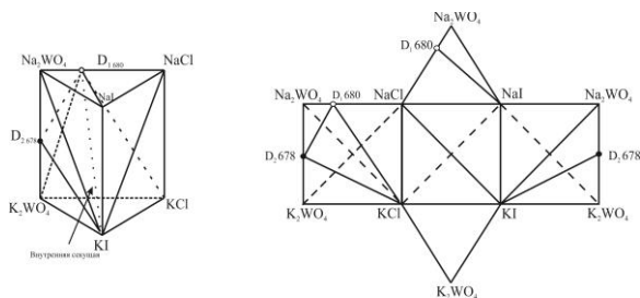
Рисунок 1 – Схема призмы составов и схема развертки четырехкомпонентной взаимной системы \text{Na,K}||\text{Cl,I,WO}_4
