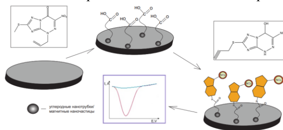
Схема иммобилизации производных триазолазинов на поверхности стеклоуглеродного рабочего электрода
