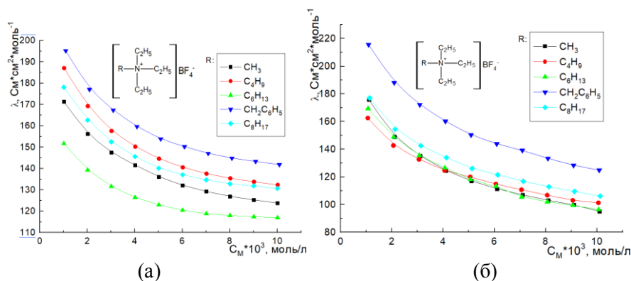
(а) (б) Зависимость эквивалентной ЭП разбавленных растворов тетрафторборатов N-алкилтриэтиламмония от концентрации в ацетонитриле (а) и ацетоне (б) при 25°С
