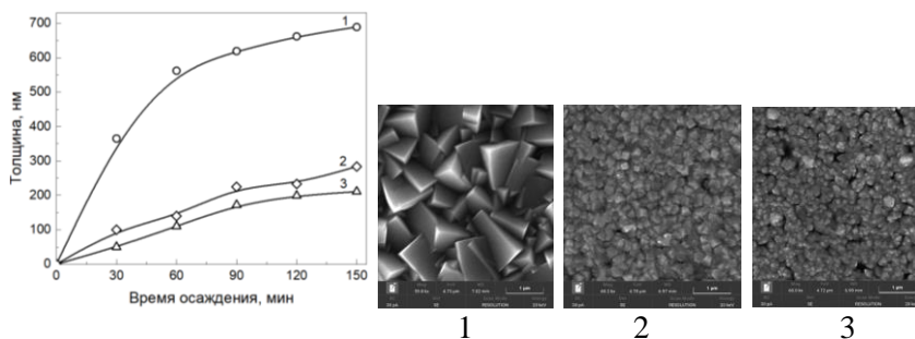
Изменение толщины от продолжительности химического осаждения на стеклянные подложки в присутствии тиомочевины (1), аллилтиомочевины (2) и тиаоацетамида (3)
