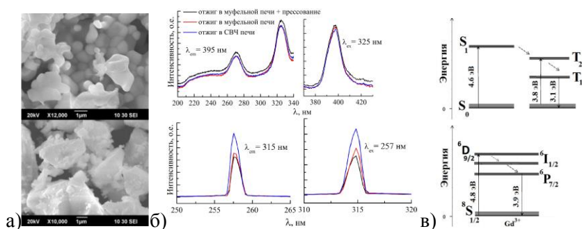
а) СЭМ-изображения образцов \text{NaGdGeO}_4 (а); б) Спектры возбуждения и люминесценции образцов \text{NaGdGeO}_4 (б)
