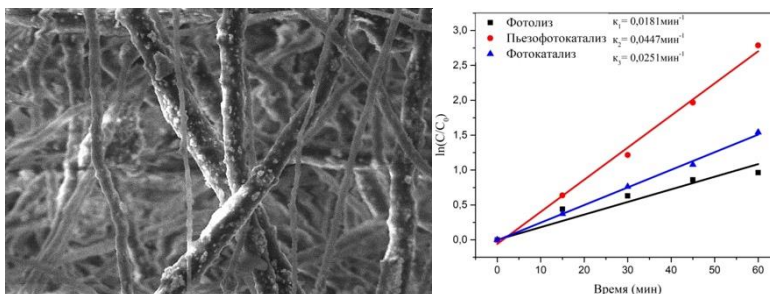
Микрофотография нановолокон ПВДФ, модифицированных ВТ (слева); Полулогарифмические анаморфозы разложения метиленового синего (МС, 1 \text{ мг л}^{-1} , 20 мл) (справа)
