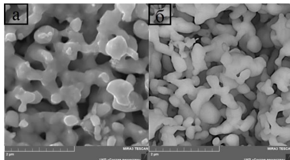
СЭМ изображение образца Ag-Zn после деаллоинга (Det: SE) (а); СЭМ изображение образца Cu-Zn после деаллоинга (Det: SE) (б)
