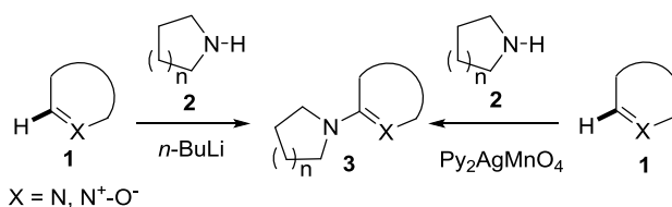
Синтез производных аминокринов
