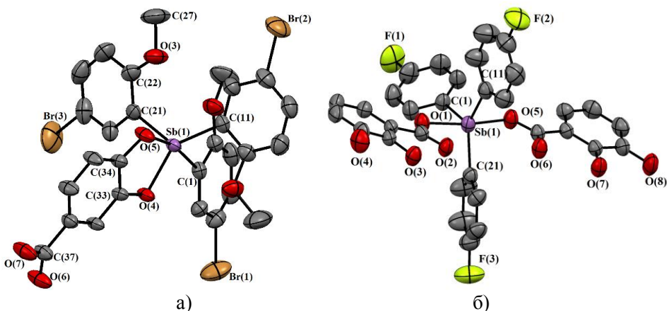
а) Строение 4-карбоксипирокатехolato-O,O'- трис (5-бром-2-метоксифенил)сурьмы;
