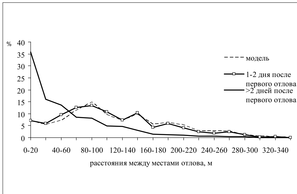
Рис. 10. Частотное распределение расстояний между точками повторных отловов зарянок осенью 1994–1996 гг. на Росситенском мысу Куршской косы. Показаны повторные отловы в первые 1–2 дня после первого отлова; повторные отловы более чем через 2 дня после первого отлова и нейтральная модель, предполагающая беспорядочные перемещения птиц по полевому стационару.
