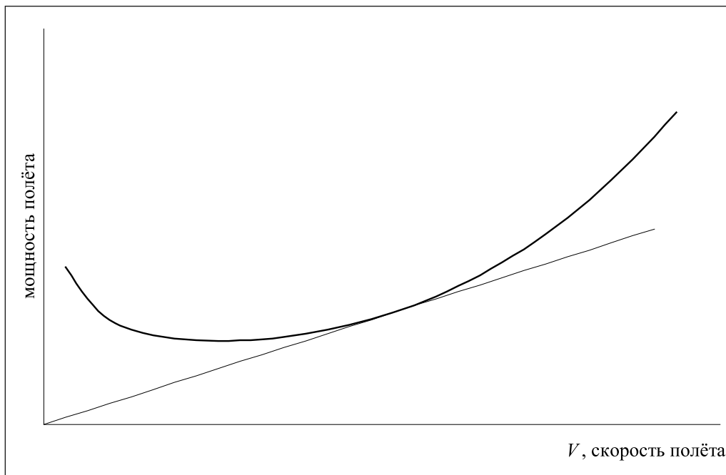
Рис. 4. Зависимость мощности полёта птиц (расхода энергии на полет) от его скорости, предсказываемая на основе аэродинамических моделей и лежащая в основе теории оптимальной миграции. V_{opt} — оптимальная скорость полёта, определяемая касательной к кривой мощности полёта из точки начала координат.
