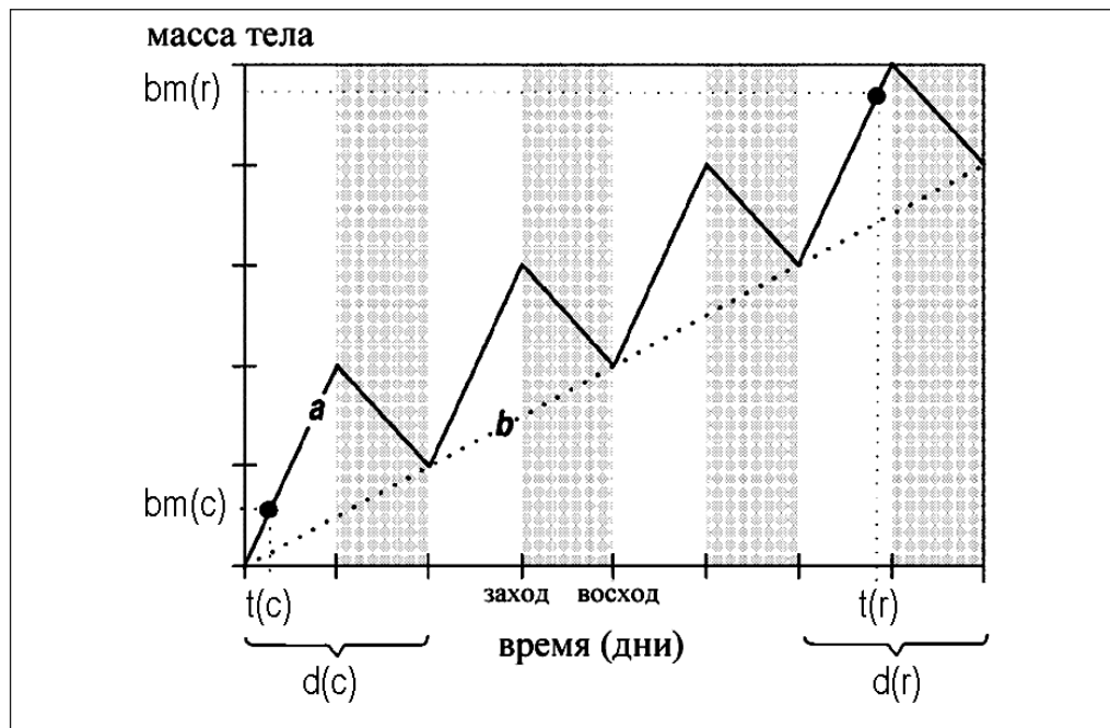
Рис. 2. Модель скорости жиронакопления на миграционных остановках (из Schaub, Jenni, 2000; с изменениями). Объяснения в тексте.
