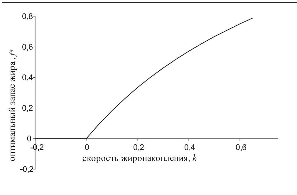
Рис. 6. График зависимости оптимального запаса жира f^* от скорости жиронакопления k .
