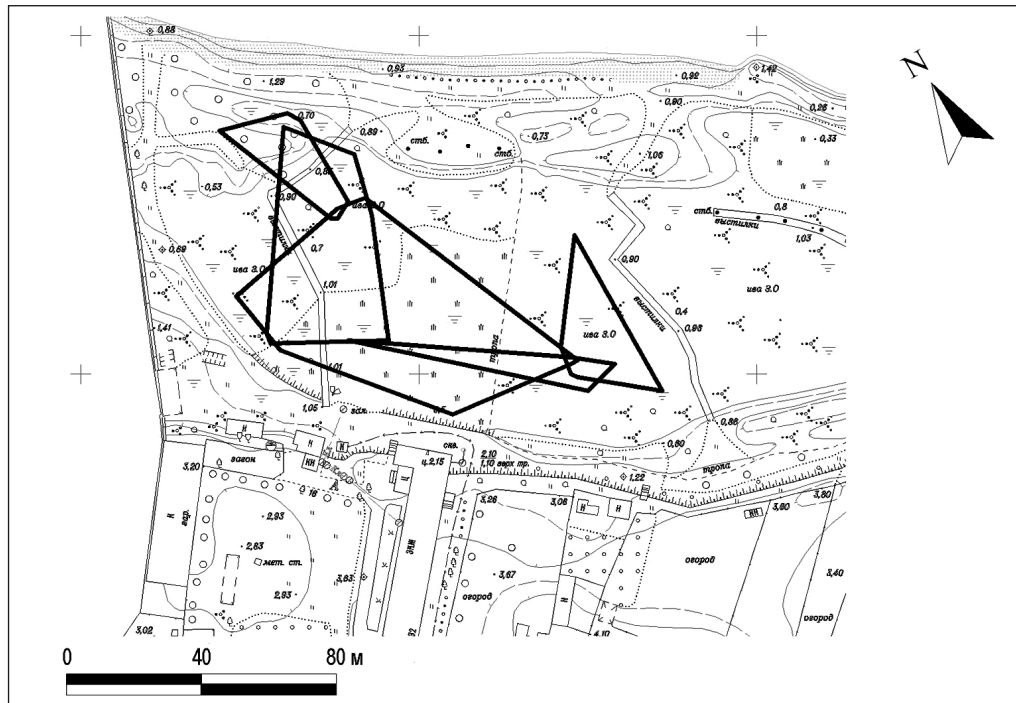
Рис. 20. Индивидуальные участки одновременно находившихся на Росситтенском мысу Куршской косы барсучков, определённые методом минимального выпуклого полигона.
