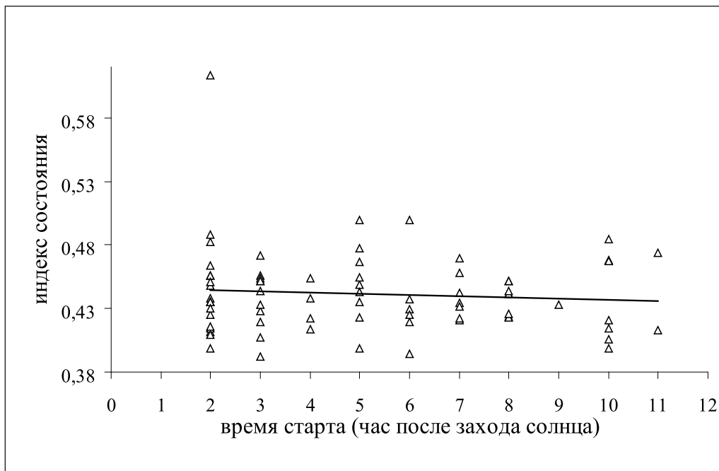
Рис. 29. Зависимость времени ночного старта у зарянок, пойманных в высокие сети осенью на Куршской косе, от индекса состояния в момент старта, пересчитанного на начало ночи (из Bulyuk, Tsvey, 2006).
