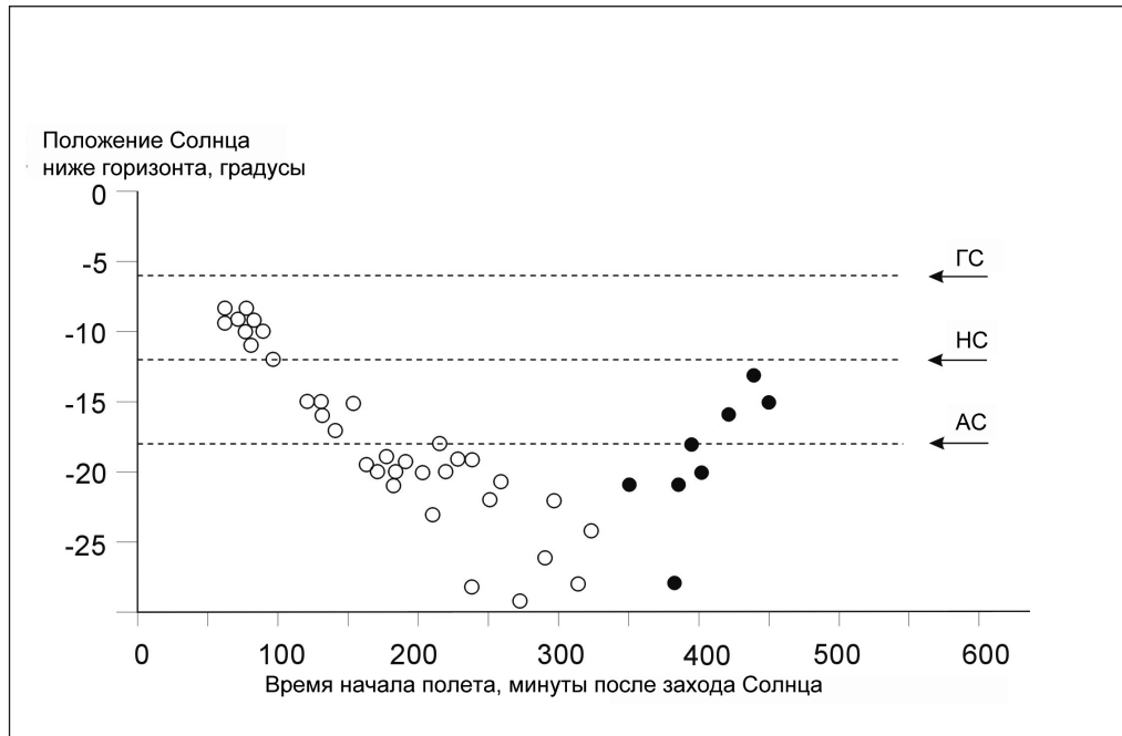
Рис. 27. Время начала ночного миграционного полёта помеченных передатчиками зарянок по отношению к положению Солнца ниже горизонта на Куршской косе осенью. Обозначения как на рис. 26.
