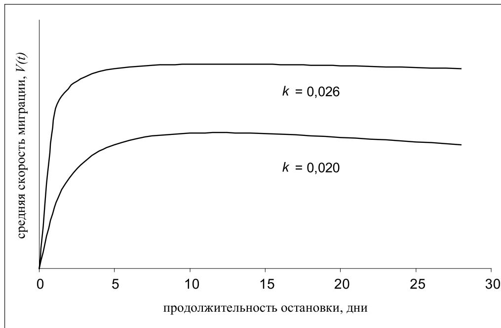
Рис. 5. График зависимости скорости миграции V(t) от продолжительности остановки t для двух различных k , c = 6000 , t_0 = 1 .
