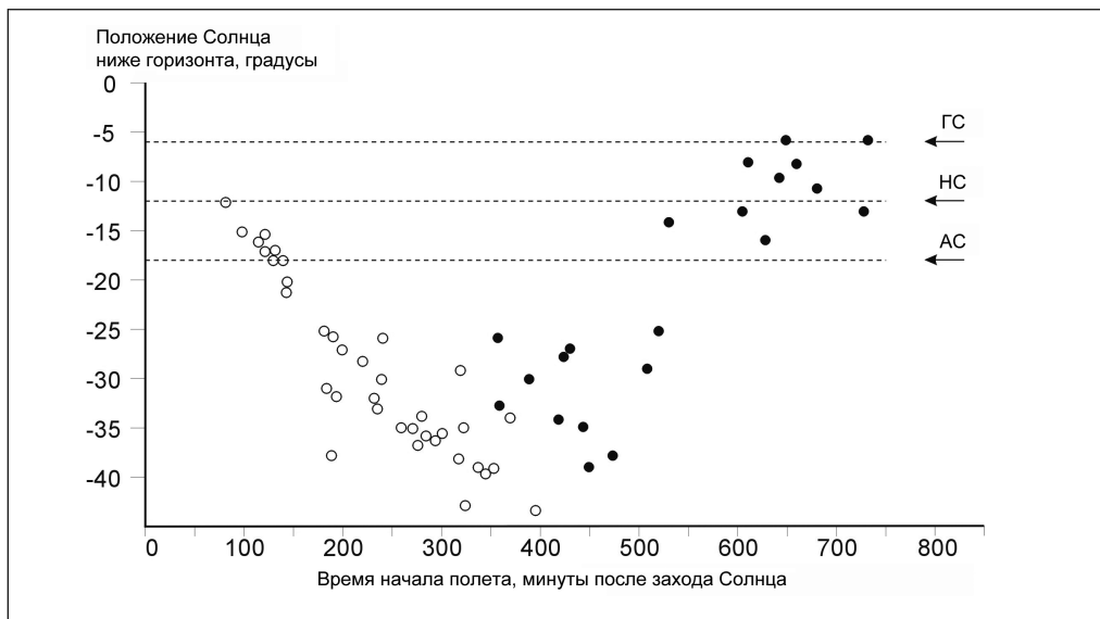
Рис. 26. Время начала ночного миграционного полёта помеченных передатчиками зарянок по отношению к положению Солнца ниже горизонта на Куршской косе весной. Стрелки указывают на время окончания гражданских (ГС), навигационных (НС) и астрономических (АС) сумерек. Белые кружки обозначают старты при снижающемся Солнце, чёрные кружки — старты при поднимающемся Солнце.
