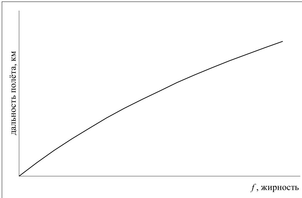
Рис. 3. Форма зависимости возможной дальности полёта птицы от её жирности ( f ), выраженной как масса жира, делённая на тощую массу тела мигранта. Согласно теории оптимальной миграции и формуле 3.1.
