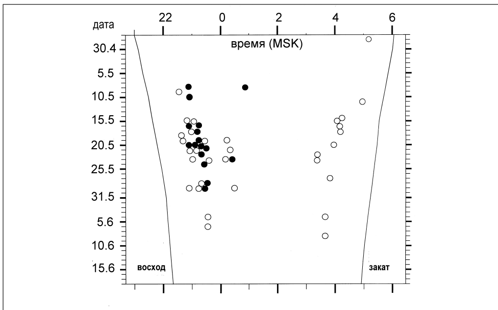
Рис. 22. Время начала ночного полёта барсучков весной на Куршской косе. Точки — птицы с кольцами (заведомо взлетающие), кружки — птицы без колец (взлетающие или садящиеся). Другие обозначения как на рис. 21.
