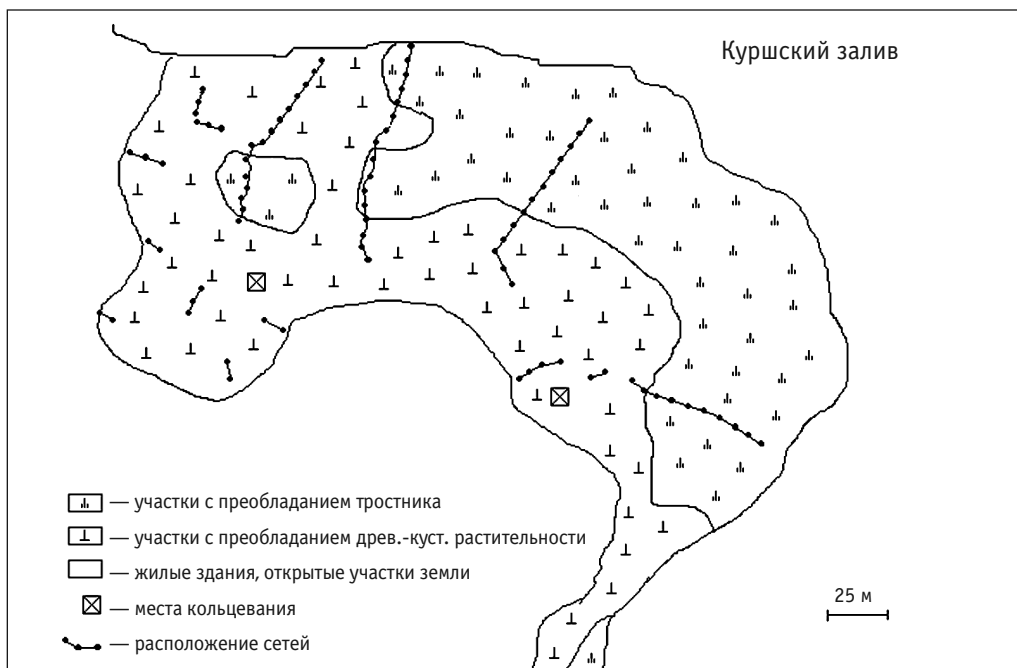
Рис. 9. Схема расположения паутинных сетей на полевом стационаре «Рыбачий» Биологической станции ЗИН РАН в 1994–2003 гг.
