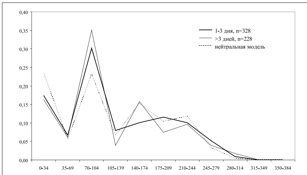
Рис. 15. Частотное распределение расстояний от места предыдущего отлёва при летне-осенних отловах тростниковых камышевок на Куршской косе Балтийского моря и сравнение его с нейтральной моделью. Отдельно рассмотрены птицы, остановившиеся на 1–3 дня и более чем на 3 дня. Различия незначимы (ANOVA по Фридману, \chi^2_{2,9} = 4,67 , P > 0,05 ).
