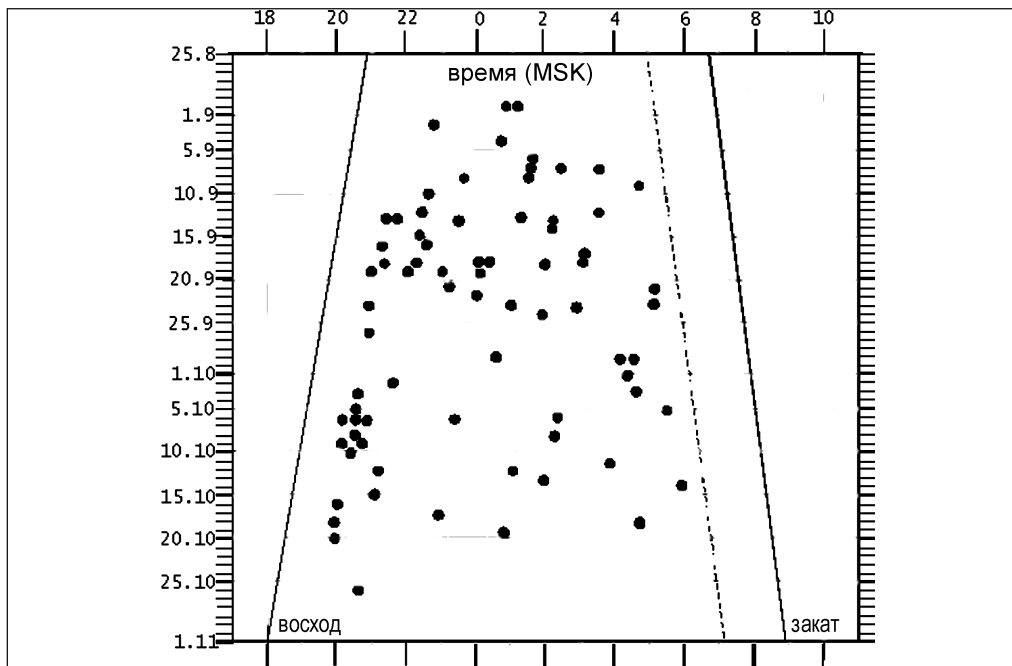
Рис. 24. Время ночных миграционных стартов зарянок осенью 1997–2003 гг. на Куршской косе Балтийского моря по данным отлова в высокие паутинные сети (из Bulyuk, Tsvey, 2006).
