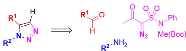
Схема 1. Ранее разработанная трёхкомпонентная реакция для получения 1,5-дизамещённых 1,2,3-триазолов
