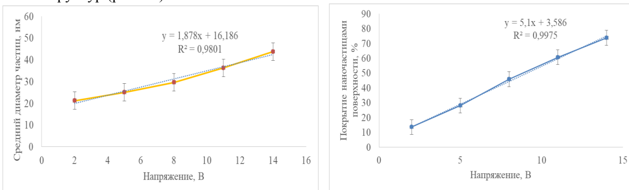
Рис. 1. а – влияние напряжения на размер образующихся наночастиц; б – влияние напряжения на распределение образующихся наночастиц.
