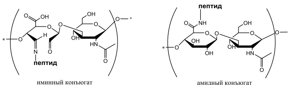
Рисунок 1. Структура конъюгатов гиалуроновая кислота-пептид.
