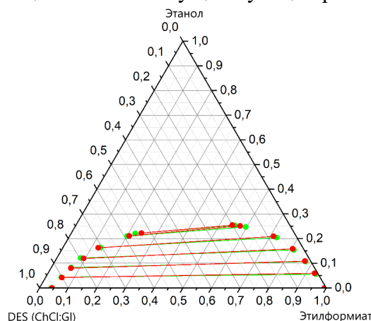
Рис. 1. Равновесие жидкость-жидкость в системе этанол – этилформиат – DES (ChCl:Gl) при 20 (●) и 40 (●) °C
