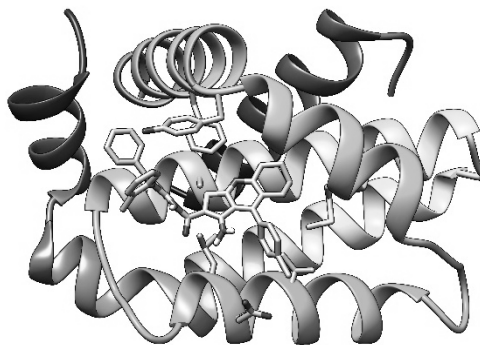
Рисунок 1. Прогнозируемая структура протеин-лигандного комплекса соединения 9b и регулятора апоптоза Bcl-2 (PDB ID 7LHB, UniProt ID P10415).
