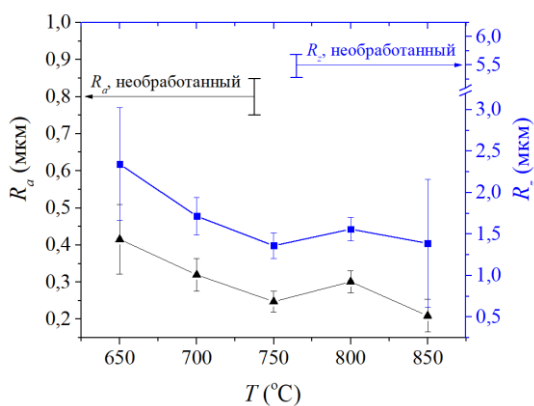
Рис. 1. Шероховатость R_a и R_z образцов из стали 12X18Н10Т до и после анодного азотирования при различных температурах.
