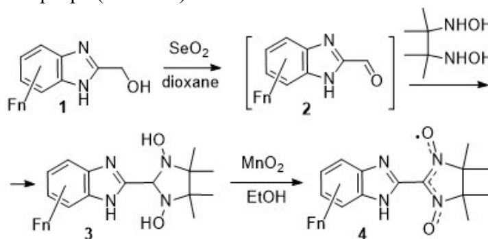
Схема 1. Синтез фторированных бензимидазоллил-замещённых нитронилнитроксилов 4
