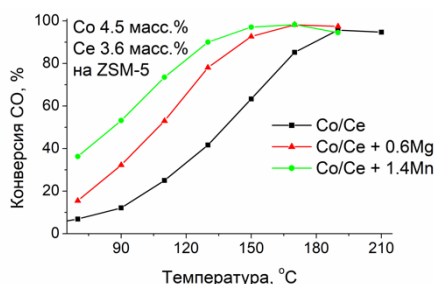
Рис.1. Влияние добавок на температурную зависимость конверсии CO в процессе PROX на катализаторах 4.5Co/3.6Ce-M/ZSM-5 (M = Mg, Mn)
