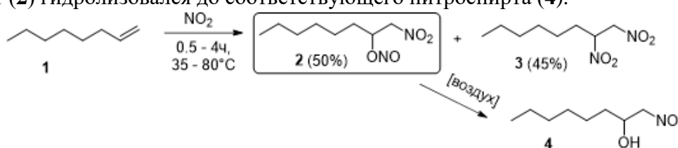
Схема 1. Нитрование октена-1 оксидом азота (IV) в среде ск- CO 2
