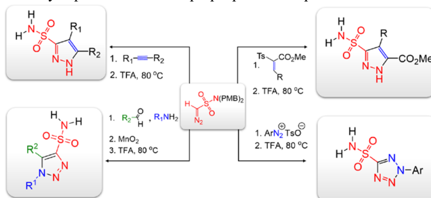
Схема 2. Построение пиразолов, триазолов и тетразолов из терминального диазометансульфонамида
