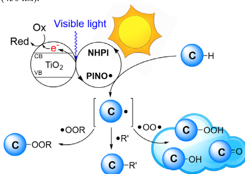
Схема 1. Реакции, осуществимые в системе NHPI/TiO 2 : окисление, окислительное С-С и С-О сочетание
