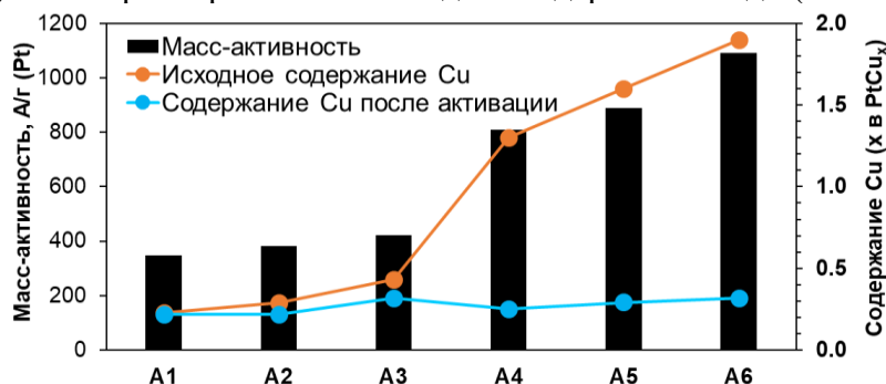
Рис. 1. Масс-активность в РВК и содержание меди до и после электрохимической активации в PtCu/C материалах.
