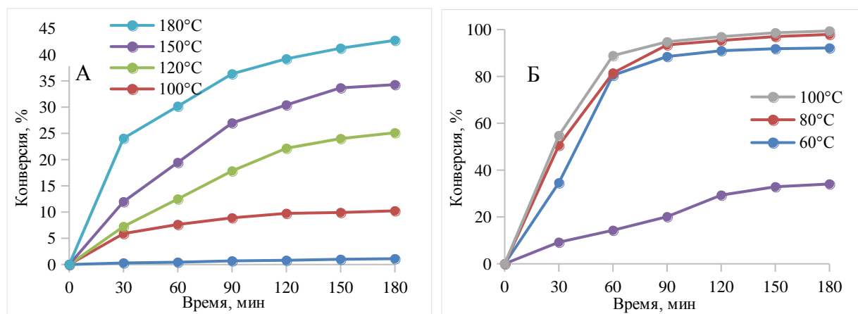
Рис.1. Зависимость конверсии бензола в водно-органической фазе от времени реакции на катализаторе Ni@ГНТ-C 16 (А), Ru@ГНТ-C 16 (Б).
