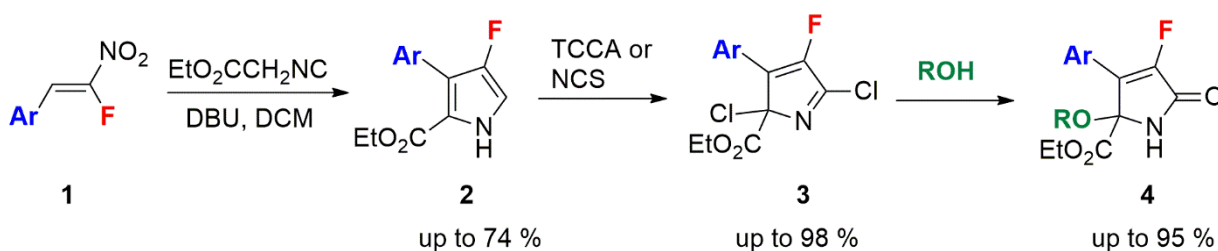
Схема 1. Получение новых 3-фтор-3-пирролин-2-онов
