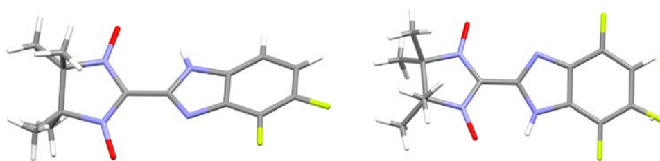
Рис. 1. Молекулярные структуры избранных фторированных нитронилнитроксилов
