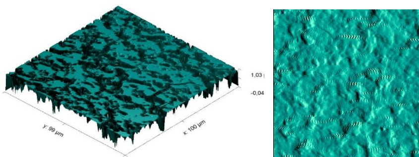
Рис.1. Морфология гальванических блестящих покрытий цинком, полученных из электролитов-коллоидов методом АСМ в «полуконтактном» режиме.
