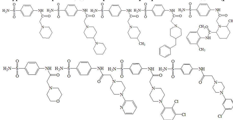
Рис. 1 Структурные формулы продуктов N-алкилирования
