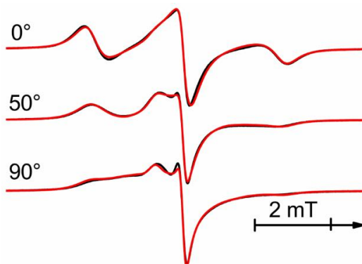
Рис. 1. Угловая зависимость спектров ЭПР системы TEMPOL-mHGO-CH 3 OH; черным - экспериментальный спектр, красным - результат моделирования.
