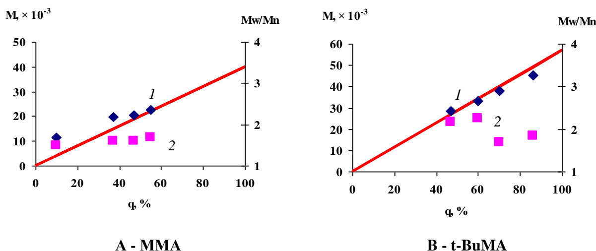
Рис. 1. Зависимости: 1 – среднечисловой молекулярной массы; 2 – коэффициента полидисперсности от степени превращения метилметакрилата (А) и трет.бутилметакрилата (В) при мольном соотношении [мономер]:[2F-BiB]:[РТН] = 400:1:0,4. Прямая линия – теоретически рассчитанное значение молекулярной массы.
