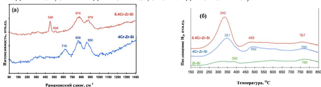
Рис. 1. КР-спектры (а); результаты H_2 -ТПВ (б).
