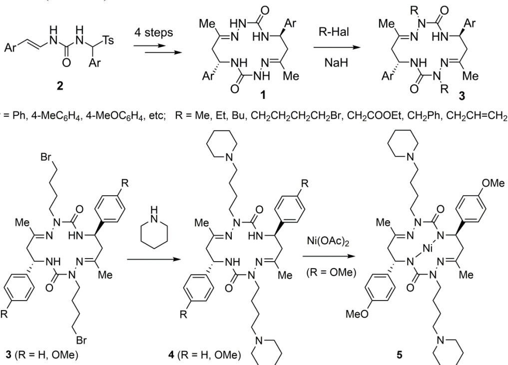
Схема 1. Синтез 2,9-диалкилзамещенных 14-членных 1,2,4,8,9,11-гексаазамакроциклов
