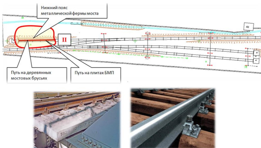
Рисунок 2 – Локация № 4 «Металлический мост с безбалластным мостовым полотном»
