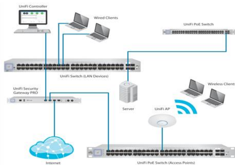
Рисунок 1 - Экосистема Ubiquiti UniFi
