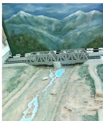
Рисунок 4 – Макет рельефа местности с участком железной и автомобильной дорог при пересечении реки Ангаракан на БАМе; показаны последствия схода селевого потока и разрушения дамбы
