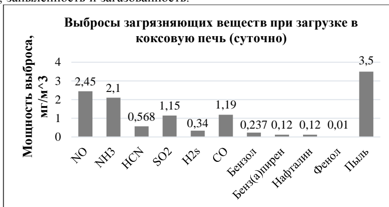
Рисунок 3. Диаграмма выбросов загрязняющих веществ при загрузке в коксовую печь
