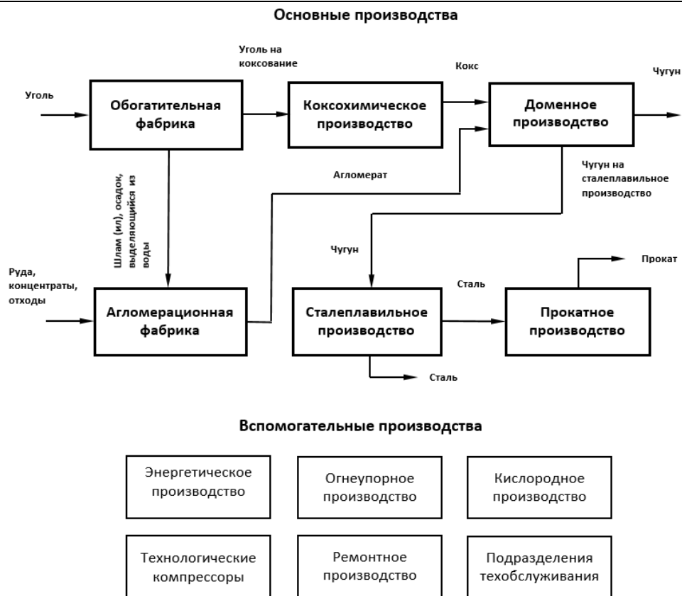
Рисунок 1. Состав основного и вспомогательных производств ПАО «НЛМК»
