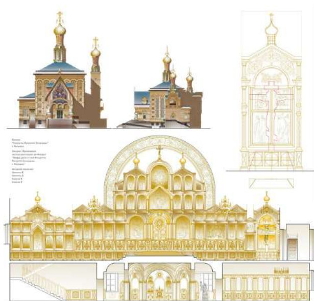
Рис. 4. Проект церкви Рождества Пресвятой Богородицы в Рыбачком. Источник: http://lovkachev.com/projects#gallery-69-2
