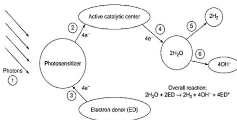
Рис. 1. Концептуальное описание гомогенных систем, выделяющих водород из разделения воды.
