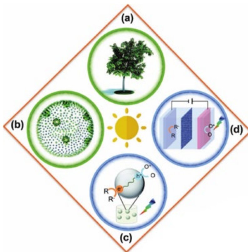
Рис.2. Типы фотокаталитических реакций. а) естественный фотосинтез в растениях, б) фотосинтез микроводорослями, в) фотокатализ наночастиц, г) фотоэлектрокатализ.
