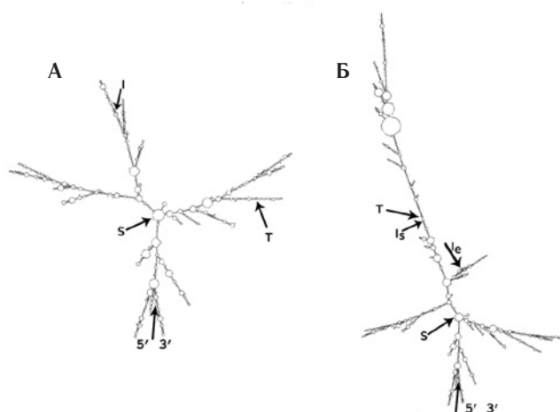
Рис. 2. Вторичная структура универсального (А) и содержащего кассетный интрон 5–6 (Б) транскриптов гена Dm nxf1 ( sbr ) Drosophila melanogaster . Примечание: стрелками указаны 5' и 3'- начало и конец транскрипта соответственно; S и T — положение иницилирующего и терминирующего кодона соответственно; I — граница 5-го и 6-го экзонов; Is и Ie — начало и конец кассетного интрона, соответственно
