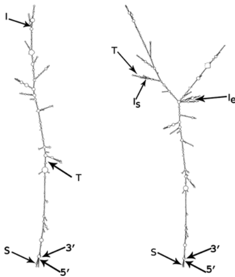
Рис. 3. Вторичная структура универсального (А) и содержащего касетный интрон 10–11 (Б) транскриптов гена Hs nxf1 Homo sapiens . Примечание: обозначения те же, что и на рисунке 2
