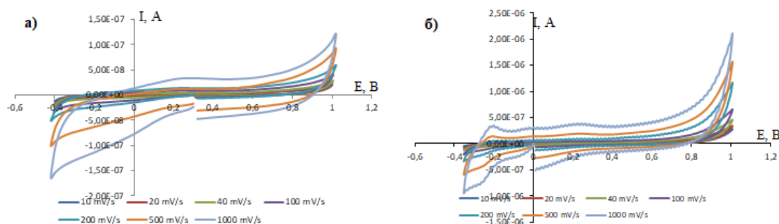
Рис. 1. Вольтамперограммы измеренные на графит-пастовом электроде, содержащем ТВАHM (VI): а) (1 : 10) масс. %, б) (1 : 1) масс. %
