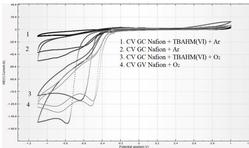
Рис. 2. Циклические вольтамперограммы, измеренные на GC электроде в нафionoвой пленке с добавлением ТВАHM (VI), в растворах, продуваемых аргоном и кислородом
