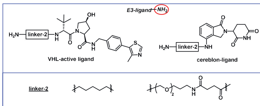
Схема 2. Использованные лиганды для E3-лигазы
