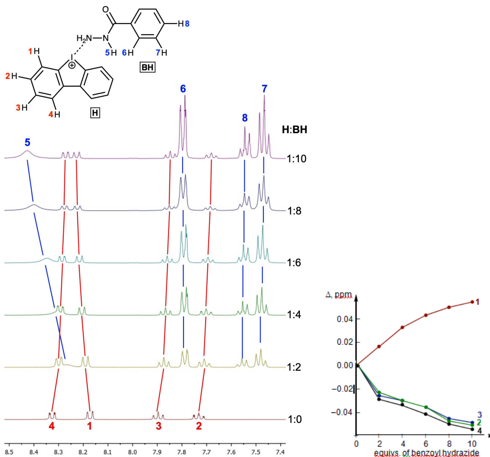
Рис. 1. ЯМР 1 H-титрование катализатора бензоилгидразидом (слева). Изменение химических сдвигов протонных сигналов катализатора в результате титрования (справа)
