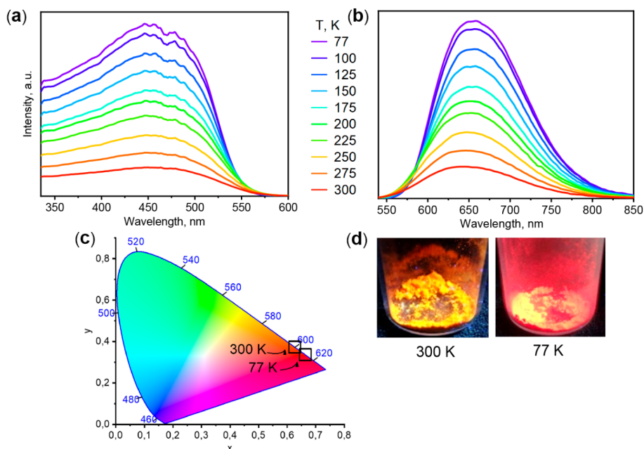
Рис. 1. Спектры возбуждения (а, \lambda_{em} = 650 нм) и эмиссии (b, \lambda_{ex} = 450 нм) [Cu_8I_8(dppz)_6] при 77–300 К; (с) Термохромизм на диаграмме цветности (d) Люминесценция [Cu_8I_8(dppz)_6] при 300 и 77 К
