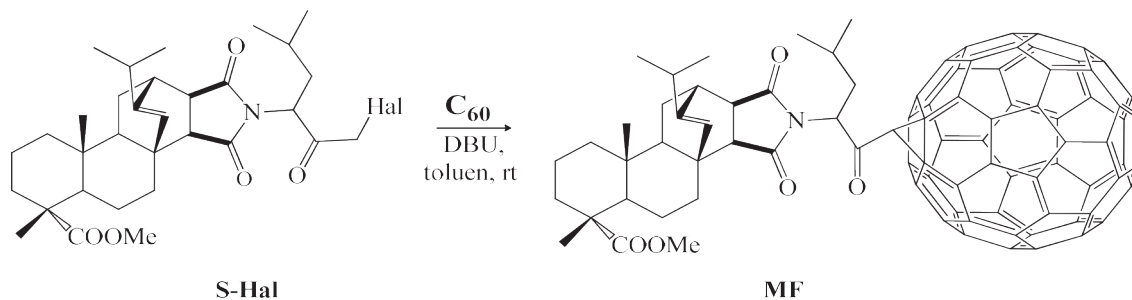
Схема 1. Взаимодействие галогенметилкетона ( S-Hal , где Hal = Cl, Br, I и F) с фуллереном с образованием метанофуллера ( MF )
