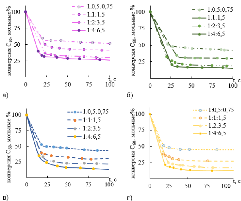
Рис. 1. Кинетические кривые расходования C_{60} при T = 10\text{ }^{\circ}\text{C} при взаимодействии с: а) Cl-; б) Br-; в) F-; г) I-метилкетон
