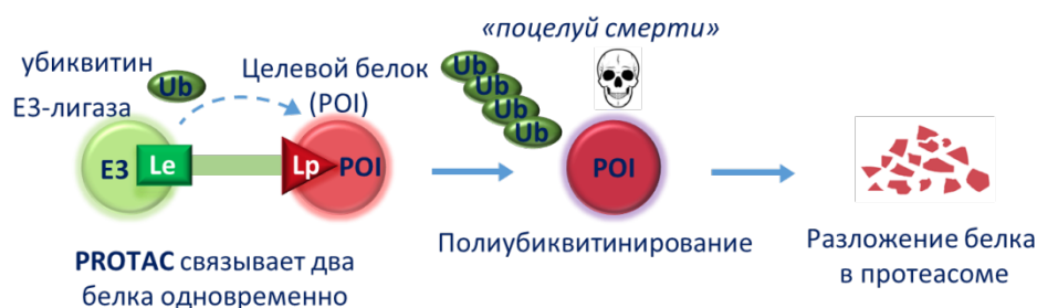
Рис. 1. Принцип действия молекул PROTACs
