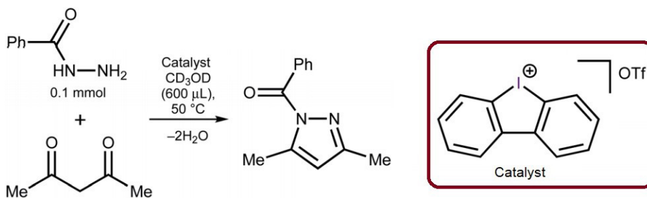
Схема 1. Схема синтеза N-ацилпиразолов
