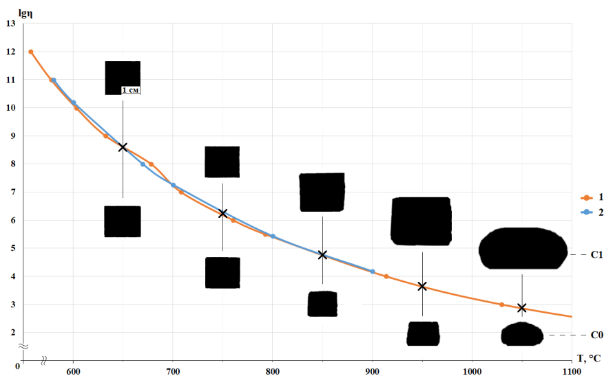
Рис. 1. Динамика плавления и вспенивания стекломатериалов в зависимости от температуры и вязкости: 1 – расчет по методу МТШ-ФФТ; 2 – расчет по методу Охотина; С0 – состав С0; С1 – состав С1
