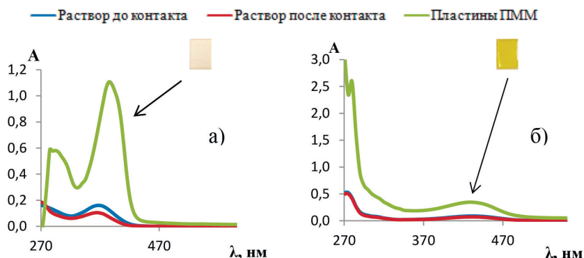
Рис. 1. Спектры поглощения тетрациклина в ПММ и в растворе до и после контакта с ней при разных значениях рН: 8,2 (а); рН 0,5 (б)
