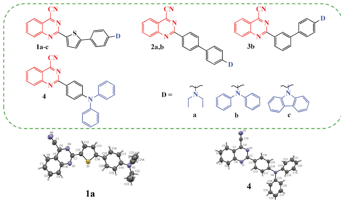
Схема 1. Молекулярная структура хи­назолинов 1a и 4 согласно РСА
