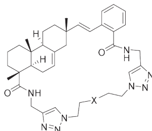
Макроцикл I тип
