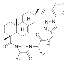
Макроцикл II тип
