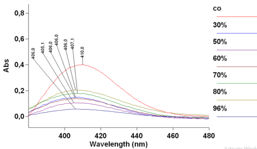
Рис. 1. Спектры поглощения комплекса рутина с алюминием в спиртовой среде (CO), и флавоноидов из растительного экстракта С (%) этилового спирта 30, 50, 60, 70, 80, 96
