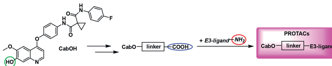
Схема 1. Синтез молекул PROTACs на основе кабозантиниба
