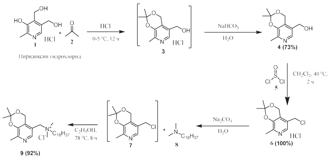
Схема 1. Опытный-промышленный способ получения соединения 9 В квадратных скобках приведены вещества получаемые in situ
