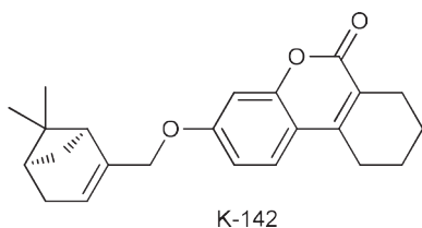
Рис. 1. Структурная формула агента К-142
