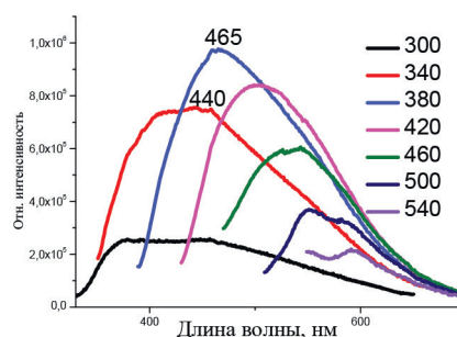
Рис. 3. Спектр возбуждения и спектр эмиссии для комплекса (3)
