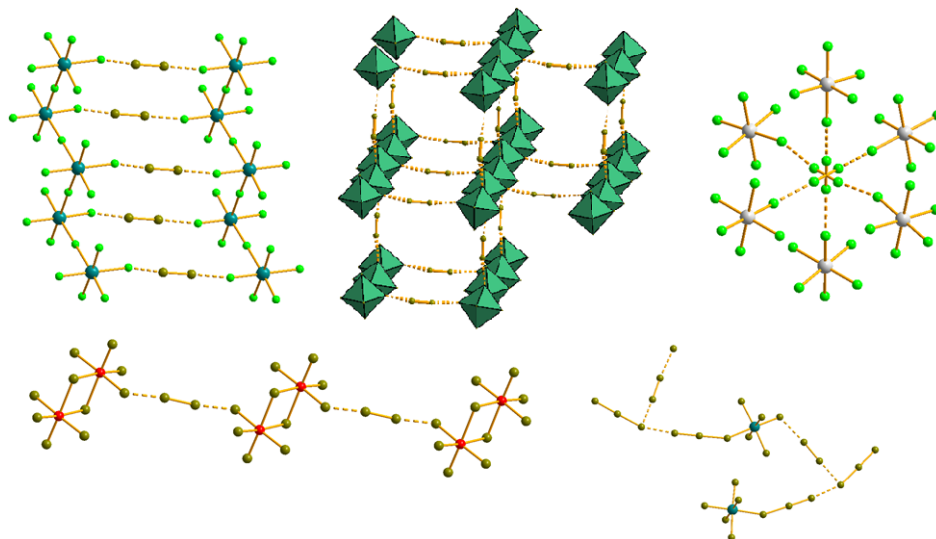
Рис. 1. Примеры анионных структур полигалогенидов различных р-элементов
