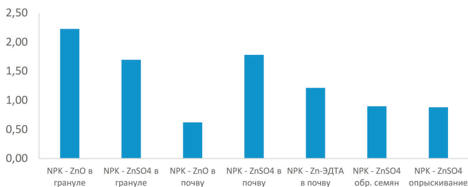
Рис. 1. Прибавка урожая зерна яровой пшеницы в зависимости от формы и способов применения цинка, г/сосуд
