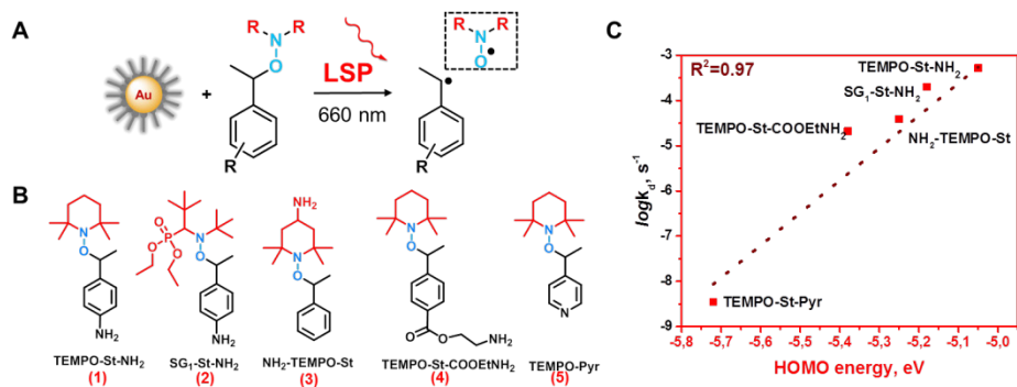
Рис. 1. А) Принцип плазмон-иницируемого гомолиза. В) Структуры исследуемых алкоксиаминов. С) Зависимость \log k_d от величины ЕНОМО
