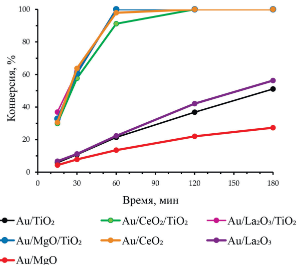
Рис. 1. Влияние природы носителя на окисление глицерина на Au/M x O y катализаторах: эволюция конверсии с течением времени. Условия реакции: T = 50 °C, 0,3 М глицерин (H 2 O), NaOH/глицерин = 4 экв., R = 1000, скорость перемешивания = 1100 об/мин
