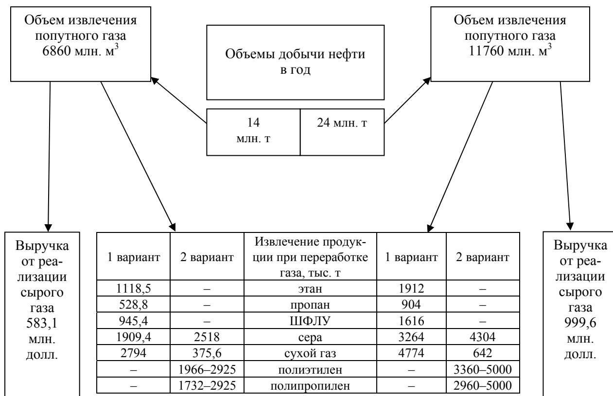
Рисунок 1. Варианты переработки попутного газа
