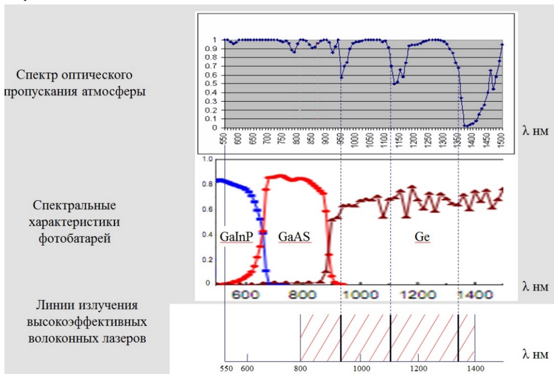
Рисунок 5. Спектр оптического пропускания атмосферы, спектральные характеристики ФЭП и линии излучения лазеров
