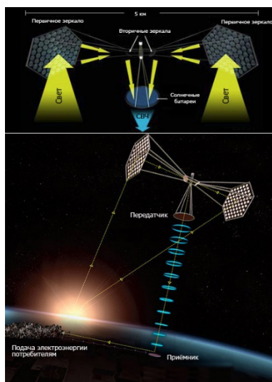
Рисунок 2. КСЭС по программе США (2007 г.)
