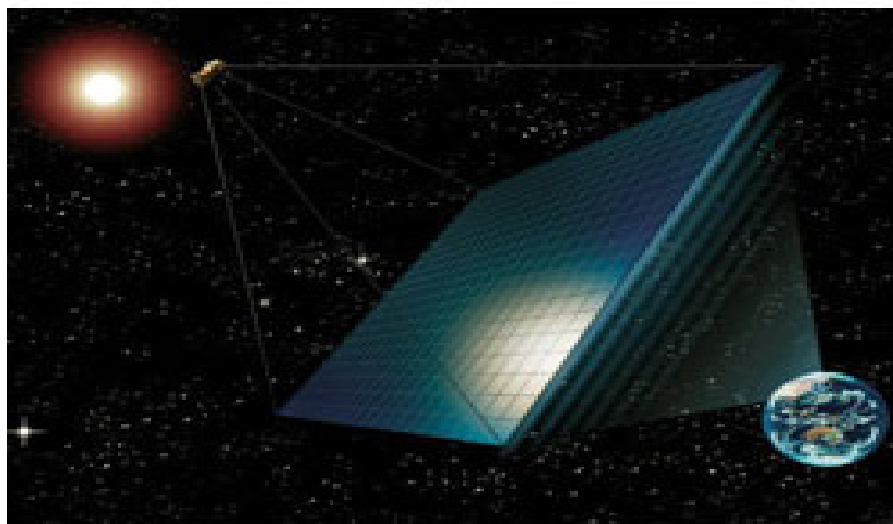
Рисунок 3. Базовый сегмент японской КСЭС размером 100×95 м и мощностью 2,2 МВт в гравитационной стабилизации
