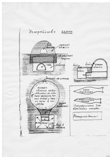
Рис.2. Устройство горна и инструменты гончара (д. Забелино, Арзамасский район, Нижегородская область).
