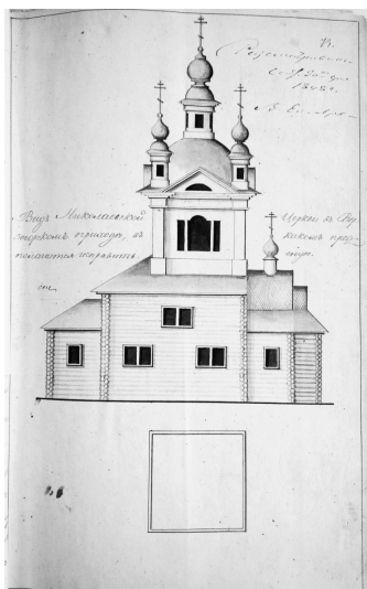
Ил. 3. «Вид Николаевской церкви в Ворзгорском приходе, в каком предполагается исправить оную. Рисовал Соловецкого монастыря монах Вениамин». Чертеж фасада. 1848 год. ГААО. Ф. 29. Оп. 4. Т. 3. Д. 137. О дозволении на место часовни во имя Преподобных Отцов Зосимы и Савватия Соловецких Чудотворцев со стоящей Онежского уезда в Ворзгорском приходе при деревне Яковлевской выстроить новый храм. Л. 73.
