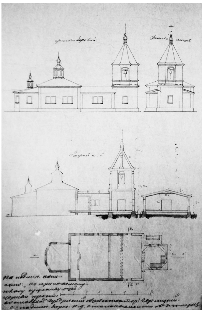
Ил. 7. Копия проекта на перестройку в Ворзогорской кладбищенской церкви пономарни и увеличения паперти и на постройку ограды. 1888 – 1889 гг. ГААО. Ф. 29. Оп. 4. Т. 3. Д. 978. О пристройке паперти и колокольни к Ворзогорской кладбищенской церкви Онежского уезда. Л. 5 об.
