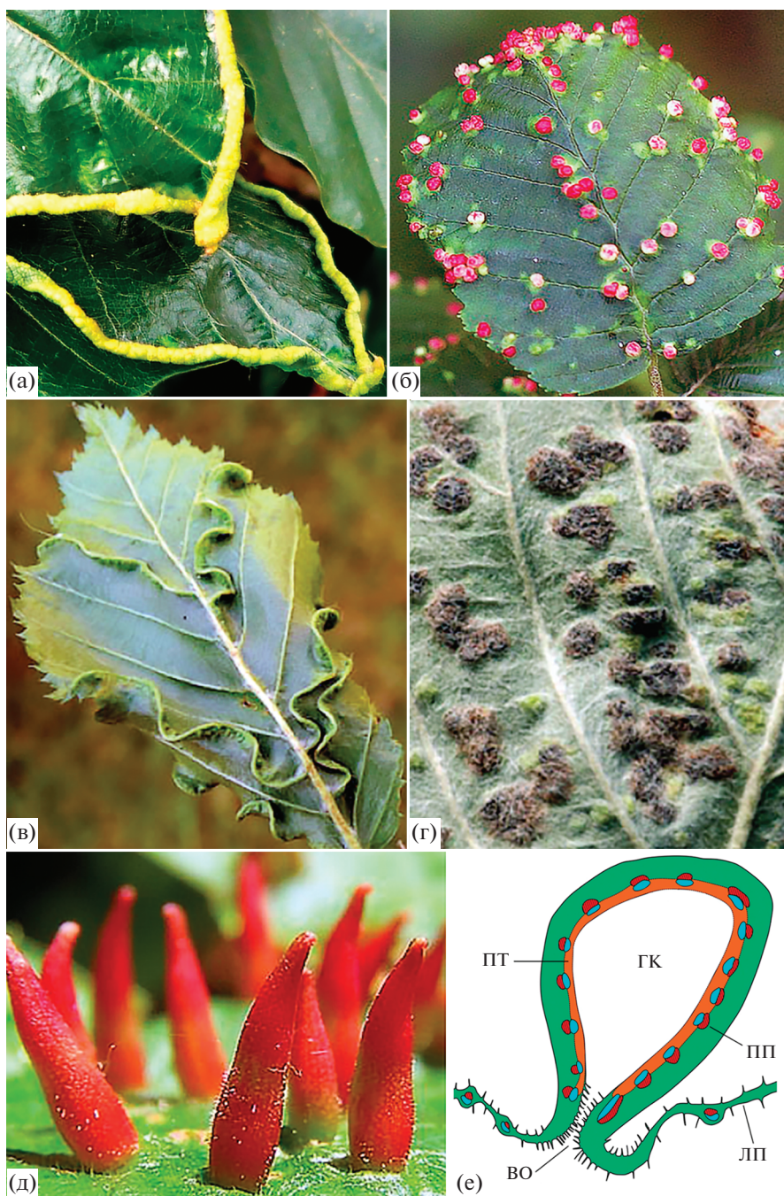
Рис. 2. Некоторые распространенные типы листовых галлов, вызываемые эриофиоидными клещами. (а) – закручивание края листа на букке Fagus sylvatica , вызываемое клещом Acalitus stenaspis Nalepa; (б) – мешковидные галлы на ольхе Alnus incana , вызываемые клещом Eriophyes laevis Nalepa; (в) – жилковые галлы на листе граба Carpinus orientalis , вызываемые клещом Aculops macrotricus Nalepa; (г) – parenхиматозные (бляшковидные) галлы на рябине Sorbus torminalis , вызываемые клещом Eriophyes sorbi Canestrini; (д) – рожковидные галлы на липе Tilia cordata , вызываемые клещом Eriophyes tiliae Pagenstecher; (е) – схематическое строение мешковидного галла. (а–д) – ориг. данные. (е) – по: Ferreira et al., 2019, с изменениями. Обозначения: ВО – входное отверстие, ГК – галловая камера, ЛП – листовая пластинка, ПТ – питательная ткань, ПП – проводящий пучок.
