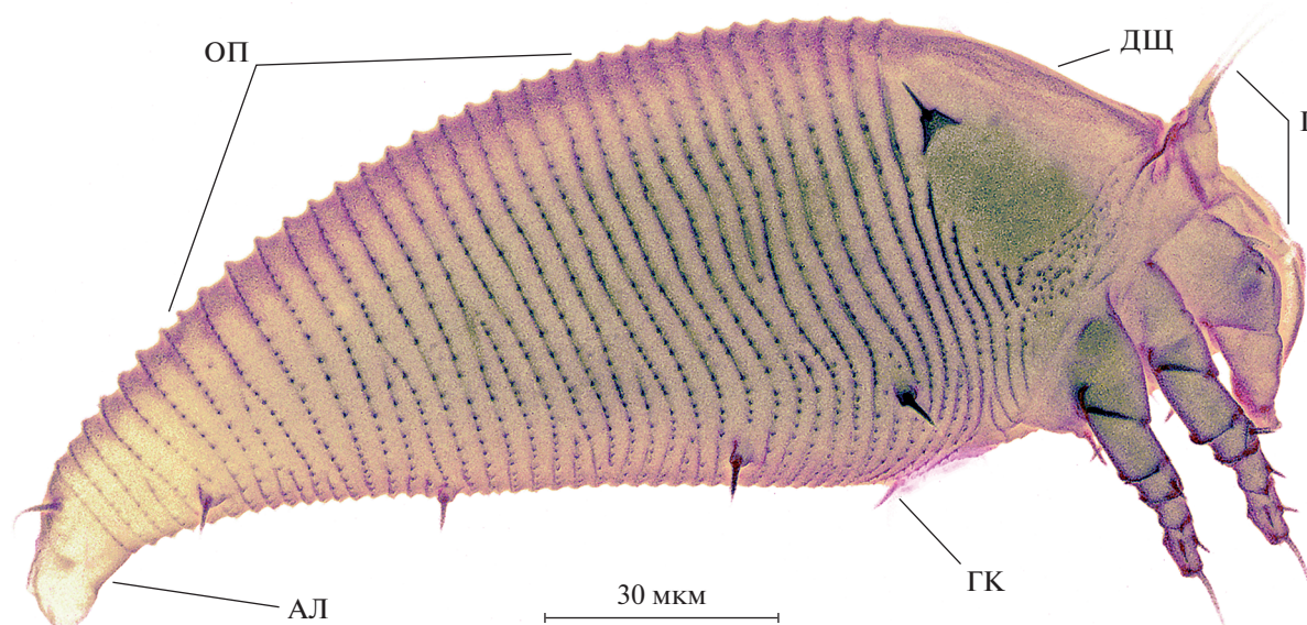
Рис. 1. Строение галловых клещей на примере самки Phyllocoptes bilobospinosus (конфокальная лазерная сканирующая микроскопия). Обозначения: АЛ – анальная лопасть, Г – гнатосома (игловидные хелицеры вывернуты вверх), ГК – генитальная крышка, ДЩ – дорзальный щиток, ОП – опистосома, покрытая кольцевидными кутикулярными складками (по: Chetverikov et al., 2019).
