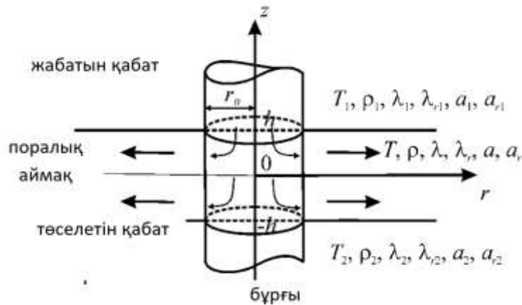
Сурет 1. Жылу алмасу есебінің геометриясы
