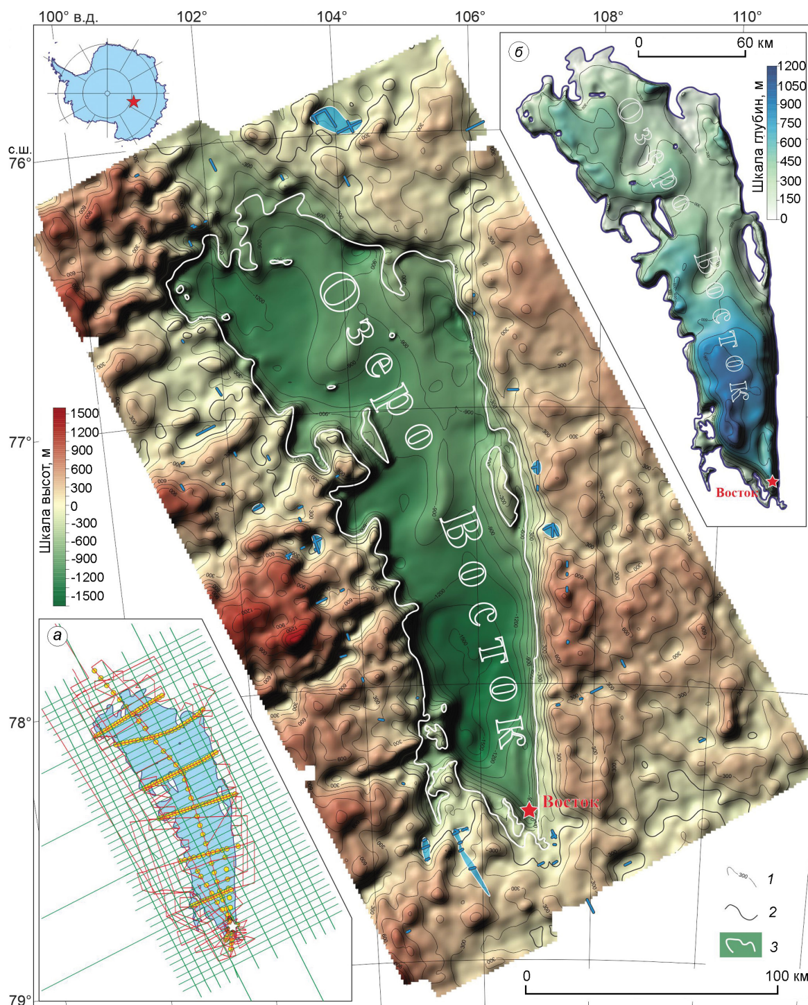
Рис. 7. Коренной рельеф и глубины подледникового озера Восток.
