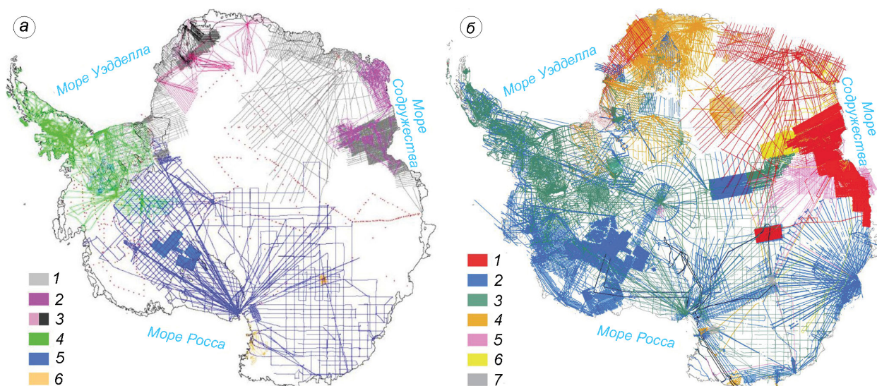
Рис. 6. Радиолокационные и сейсмические маршруты, выполненные до 1999 г. (а) и 2020 г. (б).
