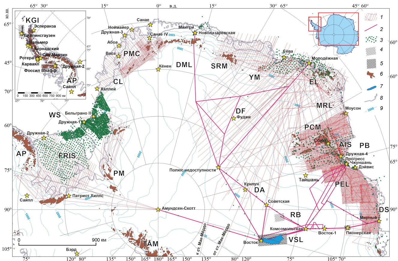
Рис. 3. Отечественные сейсмические и радиолокационные исследования в Антарктиде.
