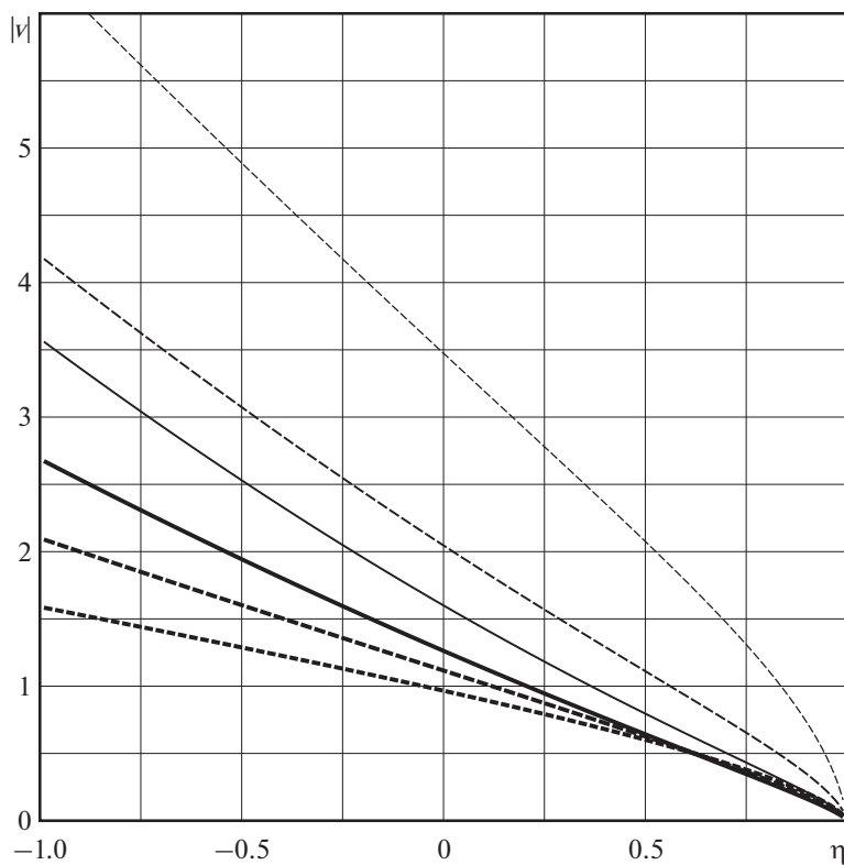
Рис. 4. Амплитуда |v| в сечениях x = 0 (жирные линии) и y = 0 (тонкие линии) на эллипсоидах с полуосями 200k^{-1} , 20k^{-1} и 15k^{-1} (сплошная линия), 200k^{-1} , 20k^{-1} и 10k^{-1} (штриховая линия), 200k^{-1} , 20k^{-1} и 5k^{-1} (пунктир).
