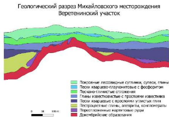
Рисунок 4. Геологический разрез Михайловского месторождения. Веретеннинский участок
