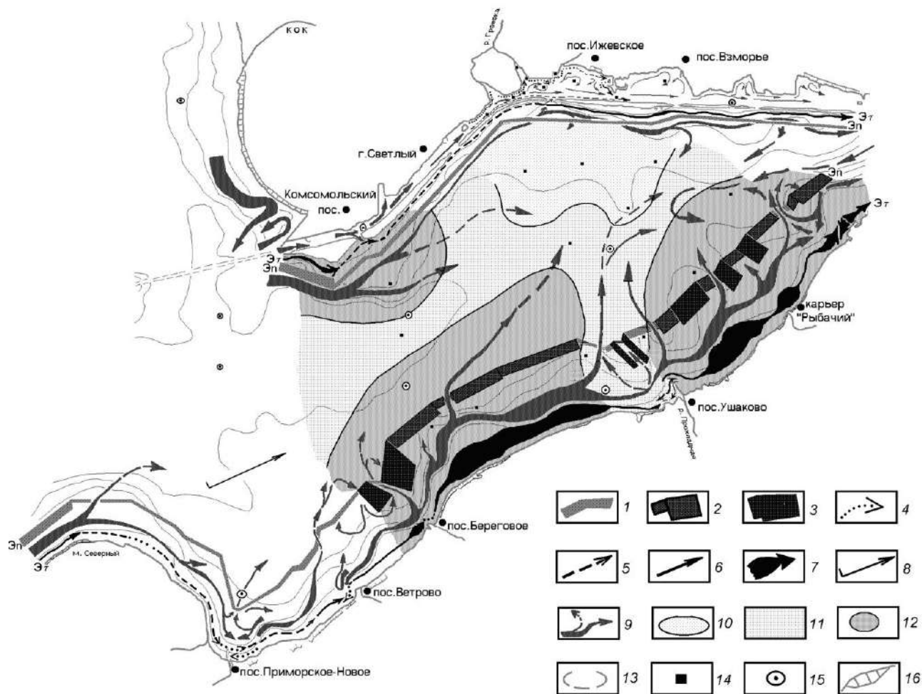
Рис. 2. Гидро- и литодинамика эстуария Калининградского залива [3]. Потоки волновой энергии, Т/с: 1, 2 и 3 – поперечные к берегу, \text{Э}_n = 1-500, 501-1000 \text{ и } 1001-1496 соответственно; 4, 5, 6 и 7 – вдольбереговые, \text{Э}_t = 0,01-1,1; 1,2-10; 11-50 \text{ и } 51-104 соответственно; 8 – результирующая ветра направлением 242^\circ повторяемостью 62 % за период отбора проб соответствовала среднегодовым параметрам (метеостанция «Калининград»); 9 – преобладающий перенос воды, взвесей и ЗВ; 10, 11 и 12 – взвешенные вещества, мг/л: 12-50, 51-100 и 101-231 соответственно; 13 – рельеф дна, 14-15 – точки отбора проб, 16 – уступы размыва берега.
