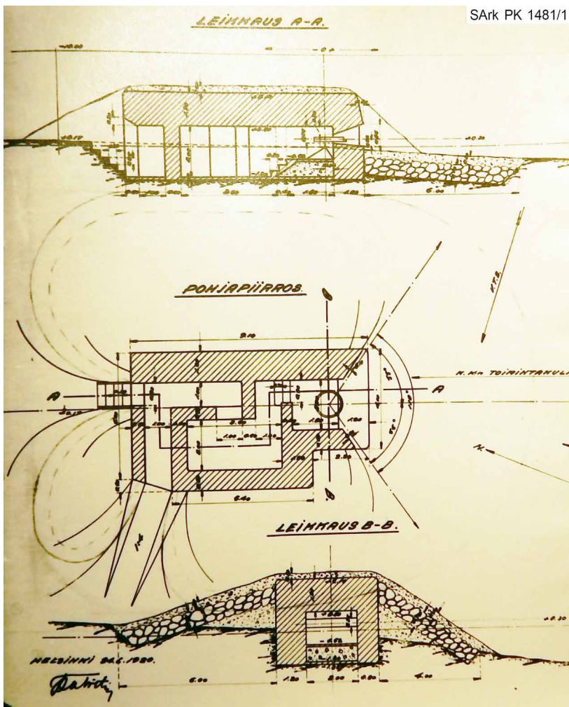
Илл. 5. Чертеж типового ДОТа постройки 1921 г.
