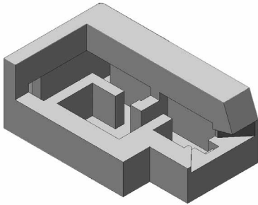
Илл. 6. 3D модель ДОТа Lă-3 в разрезе, выполненная И. А. Шереметьевым
