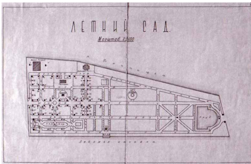
Илл. 2. Схема Летнего сада, где указаны места закопанных скульптур
