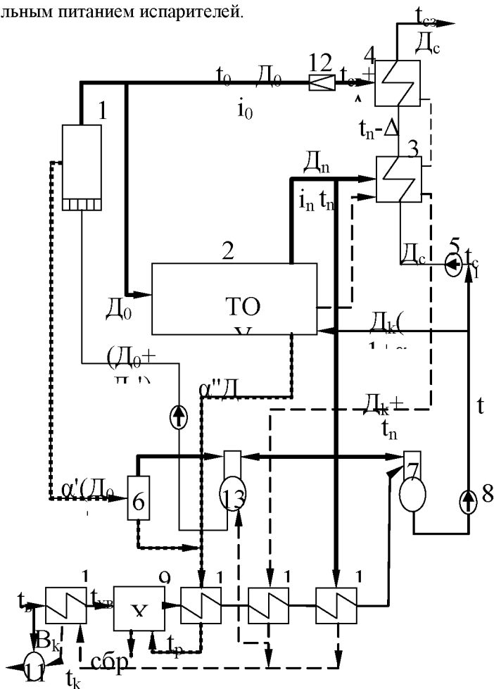
Рис. 1. Принципиальная тепловая схема паровой котельной с комбинированной выработкой тепловой энергии и обессоленной воды
