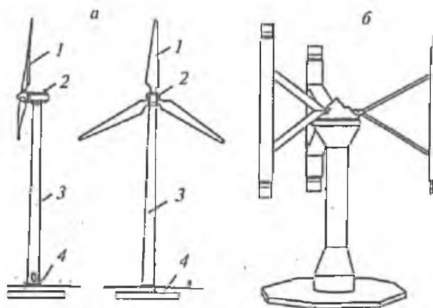
Рис. 1. Виды ветроэнергетических установок: а – ВЭУ с горизонтальной осью вращения; б – ВЭУ с вертикальной осью вращения; 1 – рабочее колесо; 2 – гондола с двигателем и редуктором; 3 – башня; 4 – фундамент
