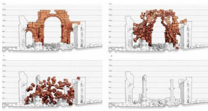
Трехмерная кинетическая модель Триумфальной арки (ICONEM)
