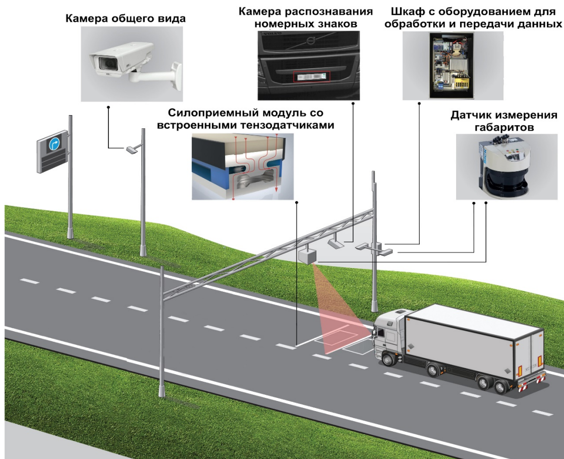
Рисунок 3. Типовая система автоматического весогабаритного контроля
