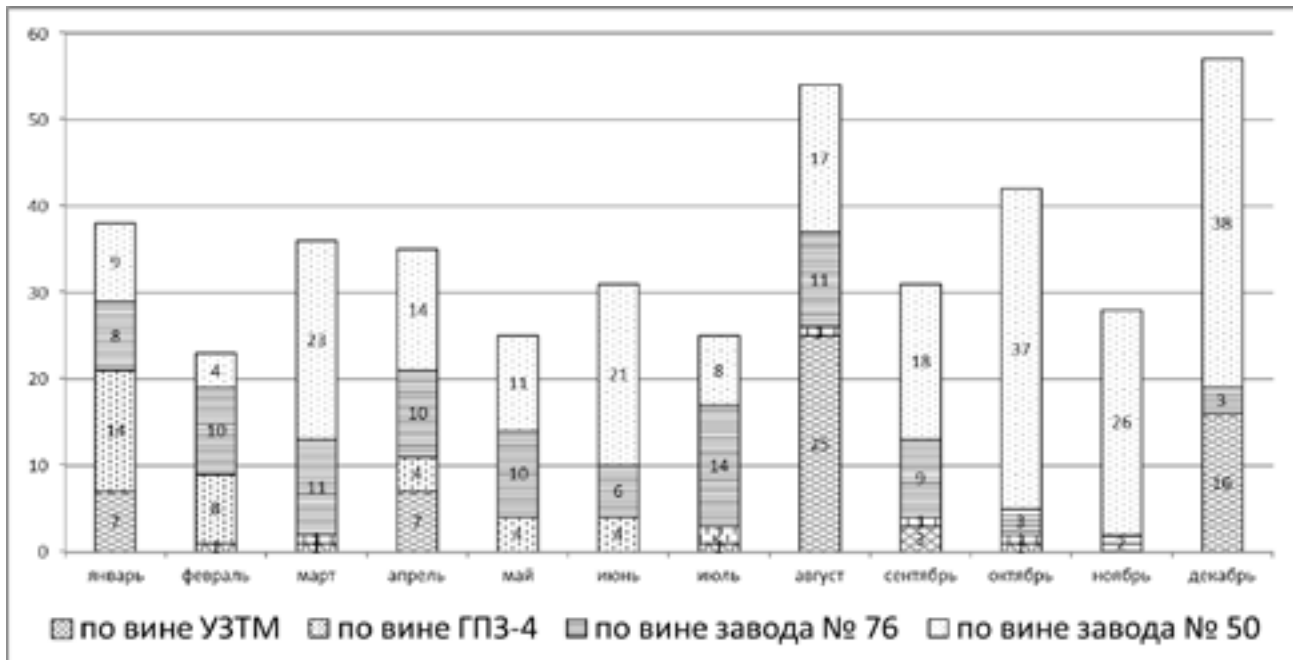
Рисунок 1 Повторные контрольно-сдаточные пробеги САУ на УЗТМ в 1944 г. (в %) [29, л. 199]
