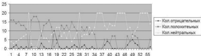
Рисунок 7. Графики изменения коррелированности процессов, сумм коэффициентов корреляции, двадцати функциональных систем организма при мысленной декламации стихов на русском и английском (после 28-го цикла измерений) языках
