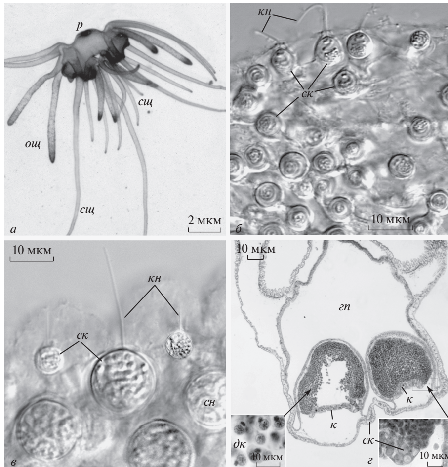
Рис. 1. Общий вид свободноживущего Polypodium hydriforme и стрекательные клетки в разных отделах тела. а – Общий вид живой 24-х щупальцевой особи, из: Raikova, 2002 с изменениями, публикуется по лицензии John Wiley and Sons № 4412061166599. б – Стрекательные клетки вокруг рта, дифференциальный контраст по Номарскому; из: Raikova, Raikova, 2016 с изменениями, публикуется по лицензии ELSEVIER № 4412051007103. в – Стрекательные клетки в опорном щупальце; дифференциальный контраст по Номарскому. г – Гистологический срез через половозрелую особь с гонадами-гаметофорами. Фиксация сулемой с уксусной кислотой, окраска гемалауном Майера. Врезка: внизу слева – двуядерные клетки, справа – участок крышечки гаметофора. Обозначения: гп – гастральная полость, дк – двуядерные клетки, к – крышечка гаметофора, кн – книдоциль, ош – опорные (локомоторные) щупальцы, р – рот, ск – стрекательные клетки, сш – осязательные (сенсорные) щупальцы.
