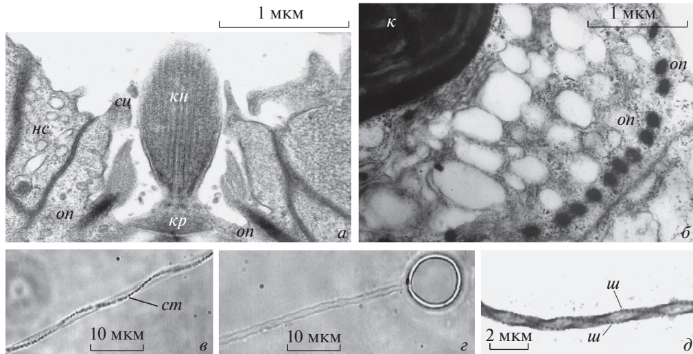
Рис. 3. Электронограммы стрекательных клеток и выстреливших стрекательных нитей.
