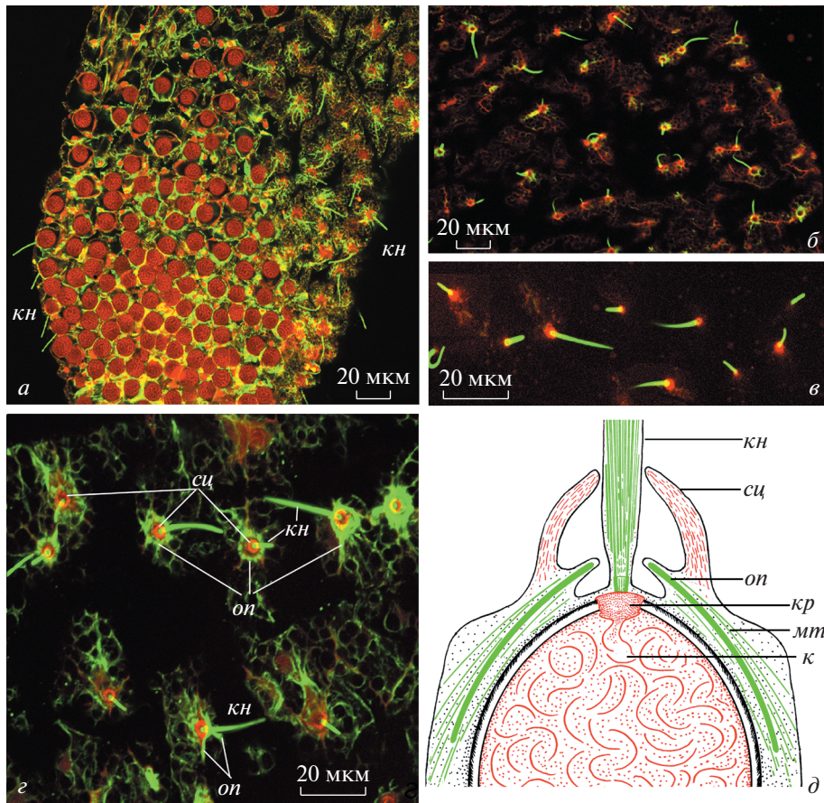
Рис. 2. Стрекательные клетки в щупальцах. Двойное окрашивание фаллоидином (красный) и антителами к \alpha -тубулину (зеленый).
