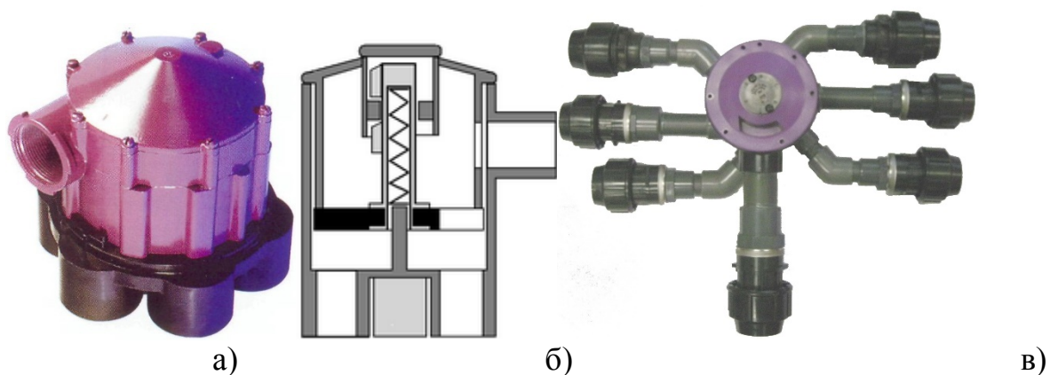
а – общий вид клапана распределительного; б – разрез; в – клапан в сборе Рисунок 4 – Распределительный клапан серии RCW
