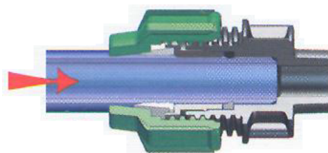
Рисунок 5 – Фитинг соединительный компрессионный
