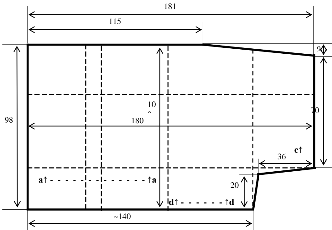
Схема 1. Размеры листа (мм), линии сгибов и расположение архивных помет. Лицевая сторона
