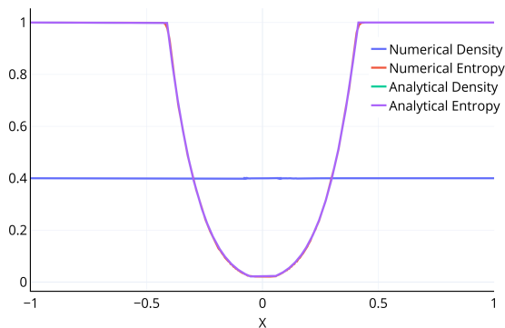
Рис. 1. Профиль плотности и энтропии ( P/\rho^\gamma , \gamma - показатель адиабаты) при решении задачи Эйнфельдта
