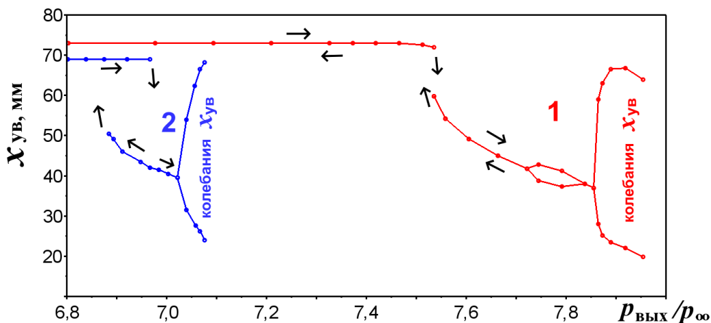
Рисунок 3 – Зависимость координаты ударной волны УВ от отношения противодавления p_{вых} к давлению в набегающем потоке p_\infty при разных числах Маха набегающего потока: 1– M_\infty=2,7 , 2– M_\infty=2,55
