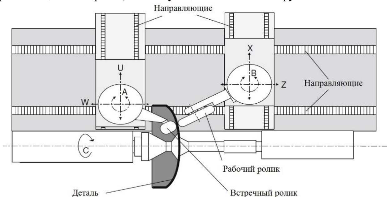
Рис. 4. Устройство станка с ЧПУ для «гибкой» ротационной обкатки [2]
