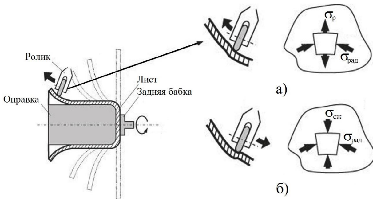
Рис. 2. Напряжения в рабочей зоне при обычной ротационной обкатке: а – движение к краю заготовки; б – движение к оправке [5, 6] локальной зоне рабочего ролика и прилегающих областях (рис. 2) [5, 6].
