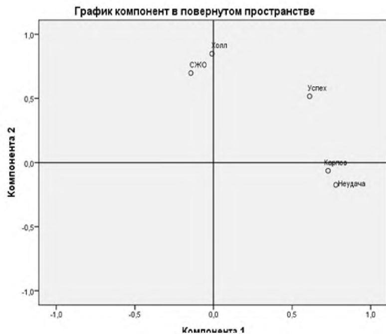
Рис. 5.2. График компонент
