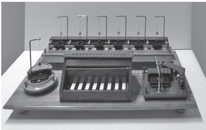
Илл. 2. Электромагнитный телеграф П.Л. Шиллинга
