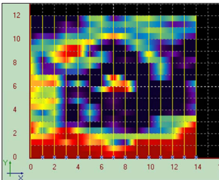
Рис. 4. Горизонтальный разрез на глубине 1,27 м при условной скорости волны в среде 5 см/нс
