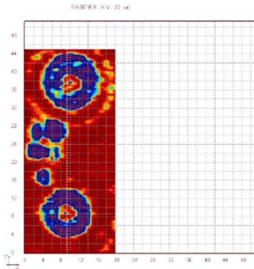
Рис. 5. Горизонтальный разрез 3D-блока георадиолокационных данных, полученных в ходе съёмки курганного могильника Кок-Жар 1 на глубине 1,3 м
