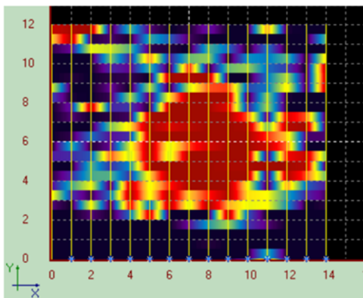
Рис. 1. Горизонтальный разрез на глубине 0,88 м при условной скорости волны в среде 5 см/нс
