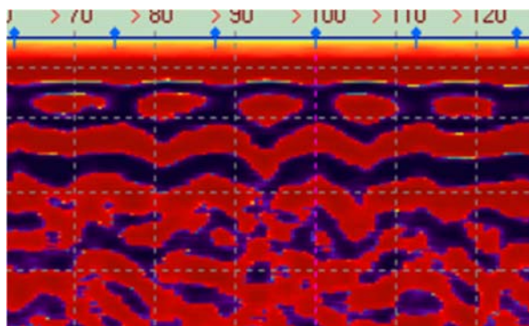
Рис. 2. Вертикальные разрезы профилей 6–9 на глубине 0–4 м при условной скорости волны в среде 5 см/нс
