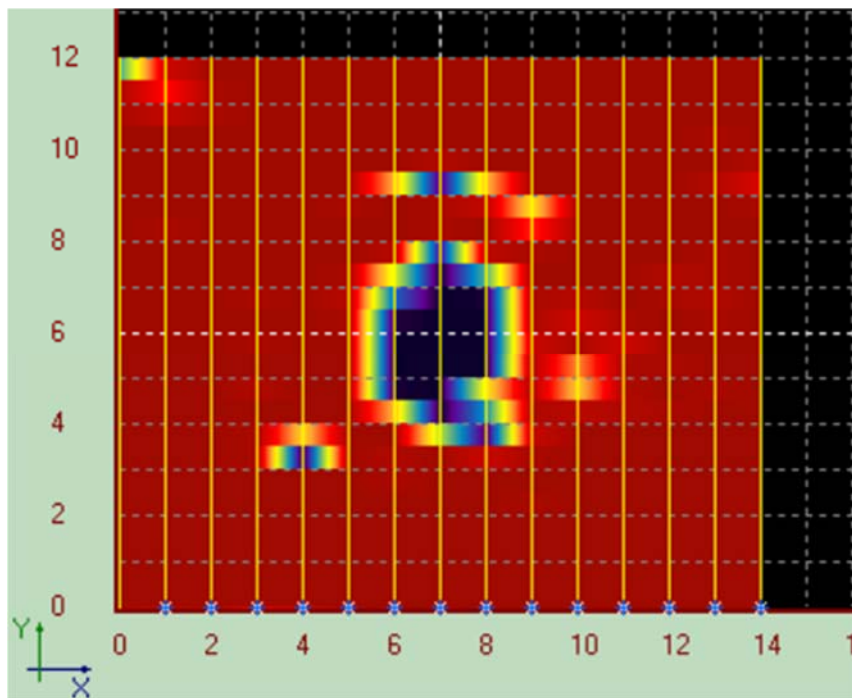
Рис. 3. Горизонтальный разрез на глубине 1,27 м при условной скорости волны в среде 5 см/нс
