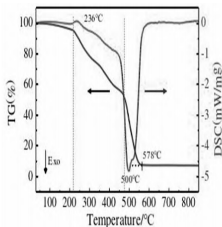
Рис 1 Кривая термического разложения геля диоксида циркония
