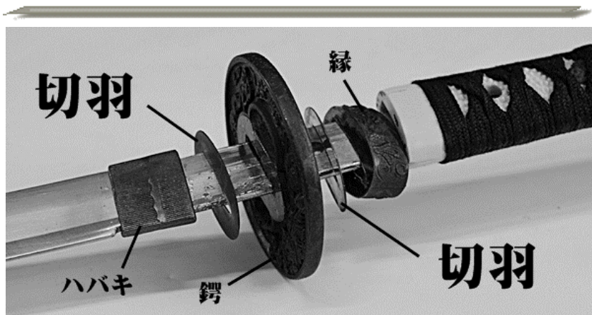
Рис. 1. Элементы японского меча 1
