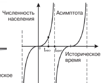
Рис. 1.3. Рост численности населения по тангенсоиде
