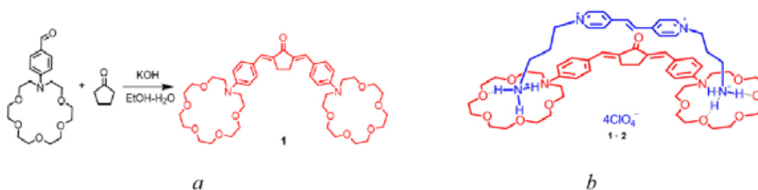
Рисунок 1. Синтез, структура диенона 1 (а) и его комплекса с диаммониопропильным производным дипиридилэтилена ( б )
