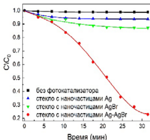
Рисунок 1. Дegrадация водного раствора МО без фотокатализатора и при наличии образцов стеклокерамики в кювете.
