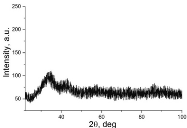
Рисунок 1. Рентгенограмма образца Sc_{33}Gd_{32}Co_{19}Al_{16}
