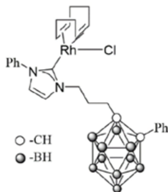
Рисунок 1. Пример полученного комплекса родия
