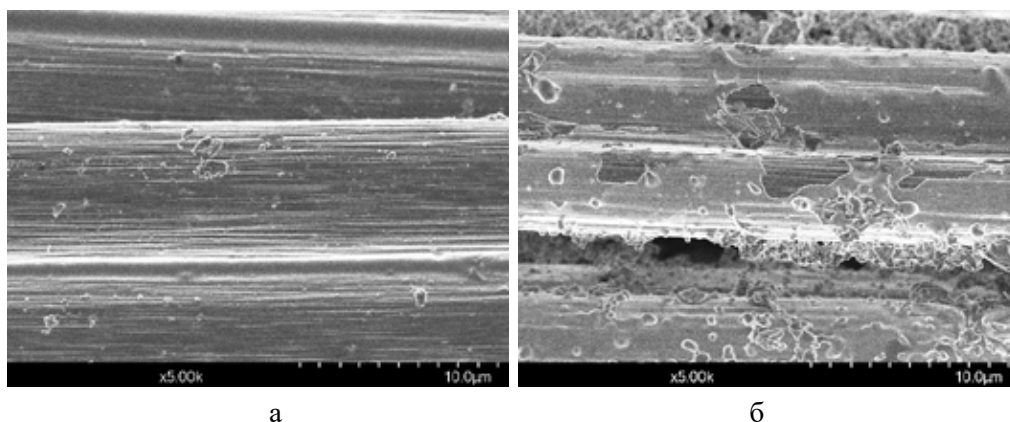
Рисунок 1. СЭМ-изображения поверхности углеродным волокон: а) после обработки ДГПЦ; б) с \text{SiO}_2 покрытием
