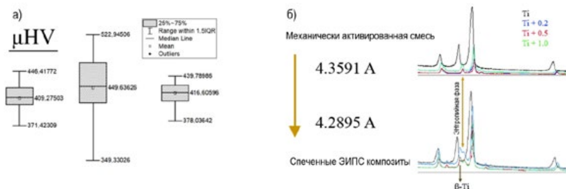
Рисунок 1. (а) Дисперсия значений твердости. (б) Фазовые изменения в процессе ЭИПС
