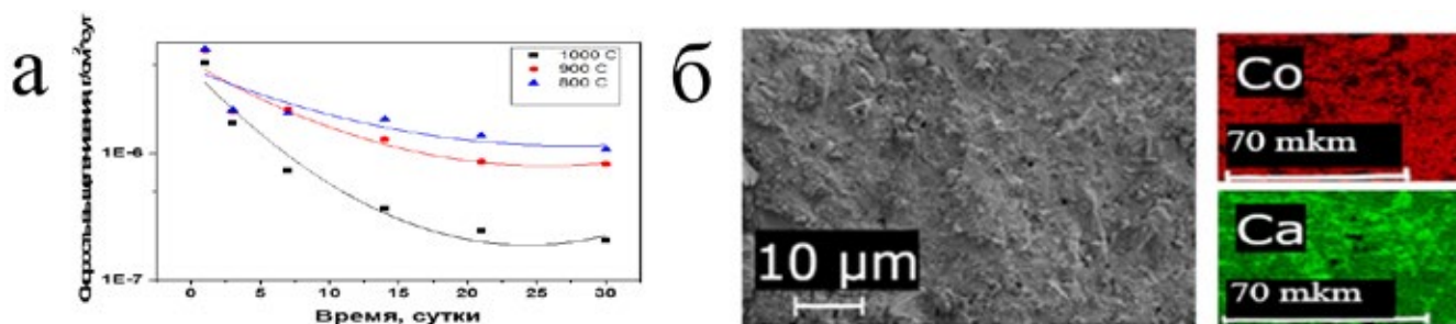
Рис.1. Скорость выщелачивания \text{Co}^{2+} из керамических матриц на основе \text{CaSiO}_3 , полученного из отходов гидротермальным методом (а), и РЭМ-ЭДС изображения \text{Co} -насыщенного и консолидированного при 1000 °С \text{CaCoSi}_2\text{O}_6 (б)
