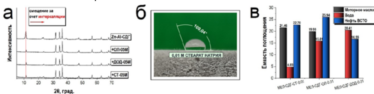
Рисунок 1. Дифрактограммы модифицированных материалов (а), контактные углы поверхности губчатого материала и воды (б), и значения емкости поглощения различных абсорбтивов модифицированными материалами (в)
