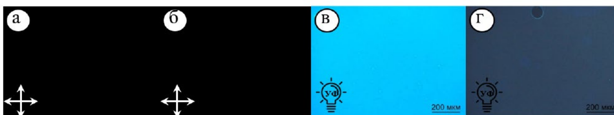
Рисунок 1. Фотографии ЛЖК на основе C_{12}EO_{10} , полученные на поляризационном и флуоресцентном микроскопе: а, в – с «синими» CD, б, г – с «желтыми» CD.
