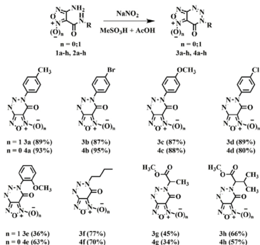
Рисунок 1. Схема синтеза новых триазинонов
