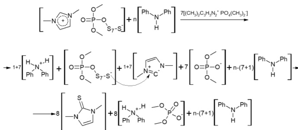
Рисунок 1. Взаимодействие ФООС с органическими основаниями на примере дифениламина.
