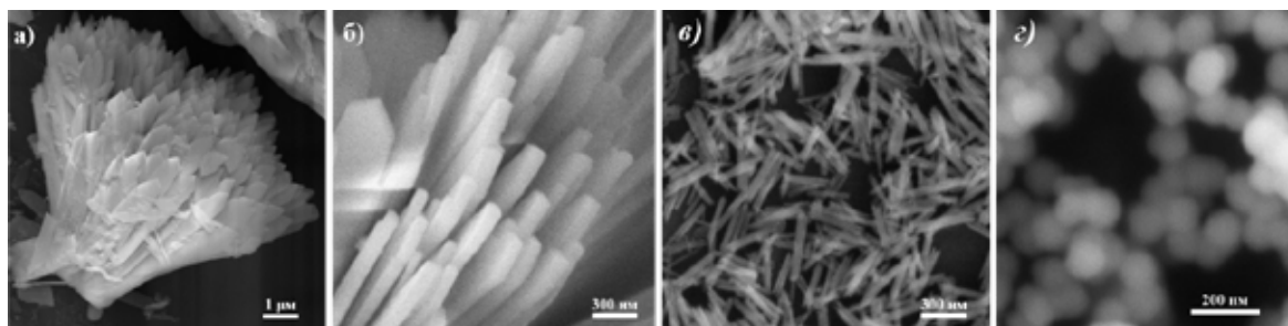
Рисунок 1. Морфология полученных наноматериалов: а), б) микрочастица \text{Sm}_2\text{O}_3 , состоящая из массива иглоподобных наночастиц; в), г) наноленты и сферические наночастицы \text{Sm}_2\text{O}_3 .
