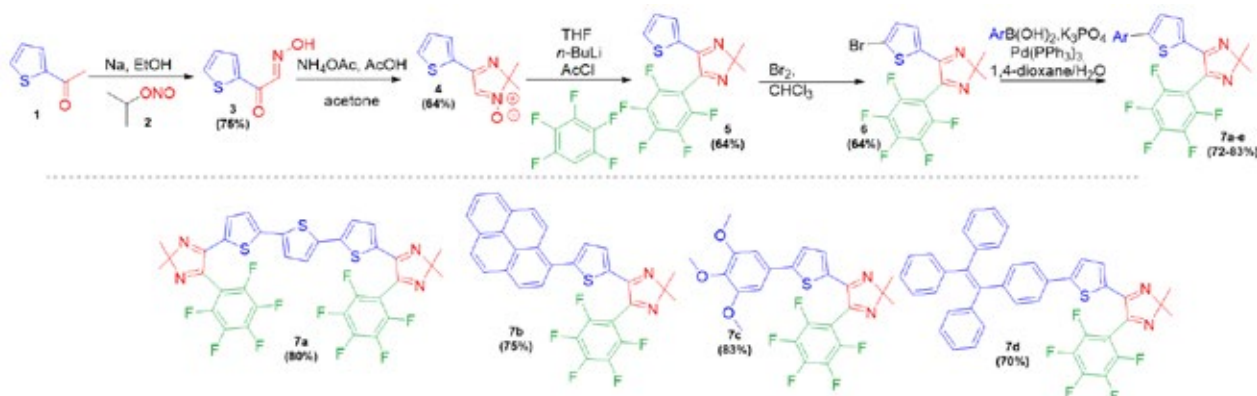
Рисунок 1. Синтез производных 2 H -имидазола, содержащих пентафторфенильный и тиофеновый фрагменты
