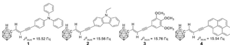
Рисунок 1. (E)-(4-арилбут-1-ен-3-ин-1-ил)- o -карбораны
