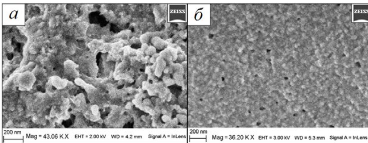
Рисунок 1. СЭМ-изображение порошков ZrO_2-4 мол. % Y_2O_3-4 мол. % Sc_2O_3 : а – полученного методом аммиачного соосаждения с последующей криогрануляцией; б – полученного методом нитрат-органического синтеза
