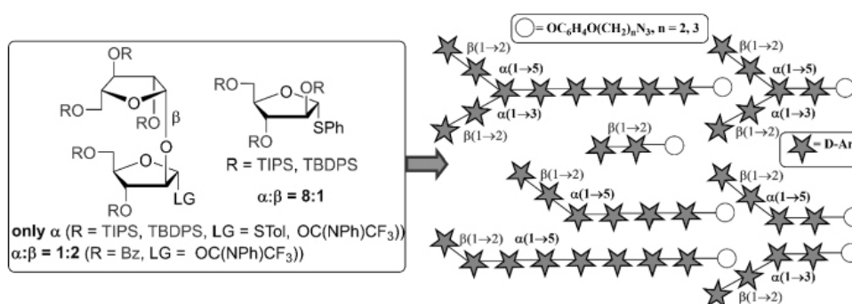
Рисунок 1. Использование гликозил-доноров, содержащих силильные группы в синтезе олигоарабинофуранозидов микобактерий с 4-( \omega -азидоалкокси)фенильным агликоном.
