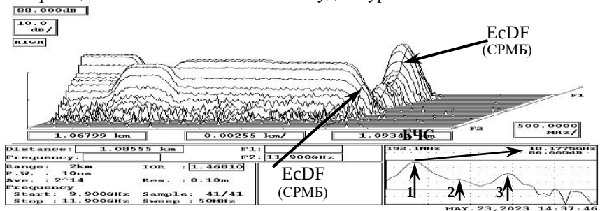
Рис. 1. Пространственное распределение СРМБ для ОБ-ЕсДФ
