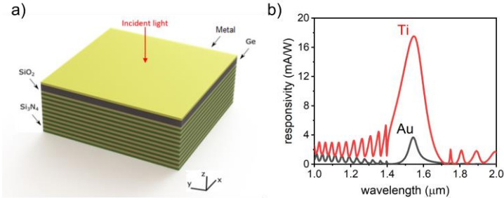
Рис. 1. Схематическое изображение исследуемой структуры: толщины слоёв \text{SiO}_2 и \text{Si}_3\text{N}_4 равны 140 нм и 120 нм, соответственно, толщина германиевой плёнки равна 50 нм, количество слоёв фотонного кристалла N = 10 (a); зависимость фоточувствительности устройства от длины волны света и материала металлической плёнки, толщина плёнки золота равна 15 нм, а титана – 7 нм (b)
