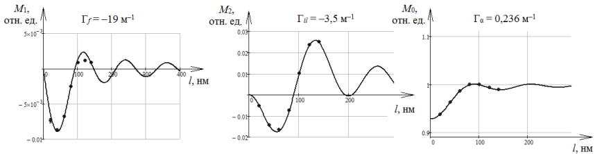
Рис. 2. Коэффициенты сигнала фазовой демодуляции для среза ( \bar{1}\bar{1}\bar{1} )
