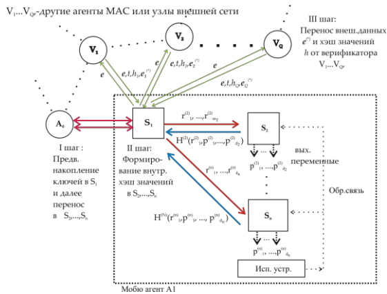
Рис. 1. Базовая схема построения верифицирующих смешанных массивов из квантовых ключей и технических параметров в паре основных взаимодействующих агентов A_0 – A_1 и в лояльных узлах V_i
