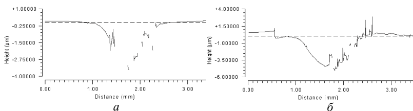
Рис. 1. Профилограммы лазерных пятен на поверхности Си в воде, плотность энергии 32 Дж/см 2 , без покрытия (а), с покрытием (б)
