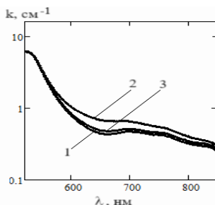
Рис. 2. Спектральные зависимости показателя поглощения в кристалле ВТО:Zn,P до (1) и после облучения светом с \lambda_i = 532 нм (2) и \lambda_n = 655 нм (3)
