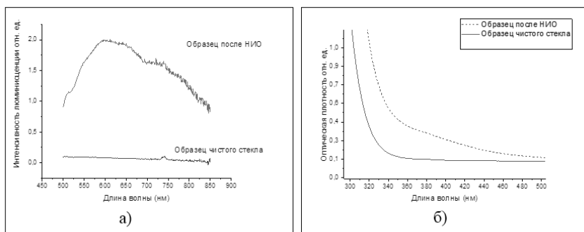
Рис. 1. Спектр интенсивности люминесценции на длине волны возбуждения 370 нм для образца до и после НИО (а), спектр поглощения образца до и после НИО (б)
