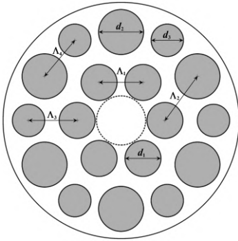
Рис. 1. Структура МВС-18
