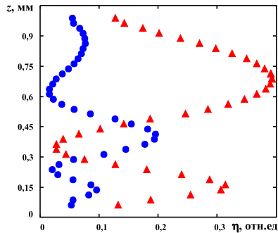
Рис. 1. Зависимости эффективности дифракции от положения зондирующего пучка вдоль оси Z кристалла, треугольники и круги — первый и второй порядки дифракции
