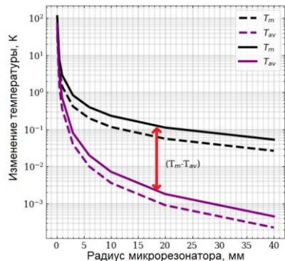
Рис. 2. Изменение температуры объёма микрорезонатора T_{av} и в области ЭМ моды T_m при мощности накачки 0,1 Вт (штриховые линии) и 0,2 Вт (сплошные линии)
