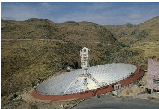
Рис. 1. Радиооптический телескоп РОТ-54/2.6 (общий вид)
