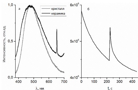
Рис. 1. Нормированные спектры фотолюминесценции (а) исследуемых образцов. Кинетика затухания фотолюминесценции керамического образца (б)
