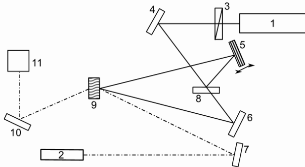
Рис. 1. Схема экспериментальной установки: 1 – импульсный Nd:YAG лазер (532 нм), 2 – He-Ne лазер (632,8 нм), 3 – полуволновая пластинка, 4, 6, 7, 10 – глухое зеркало, 5 – колеблющееся зеркало, 8 – полупрозрачное зеркало, 9 – кристалл силиката висмута (BSO), 11 – ПЗС-камера.
