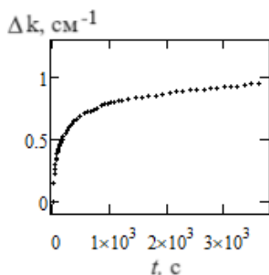
Рис. 1. Динамика изменения показателя поглощения света в кристалле ВТО:Zn,P, индуцированная излучением с длиной волны 532 нм
