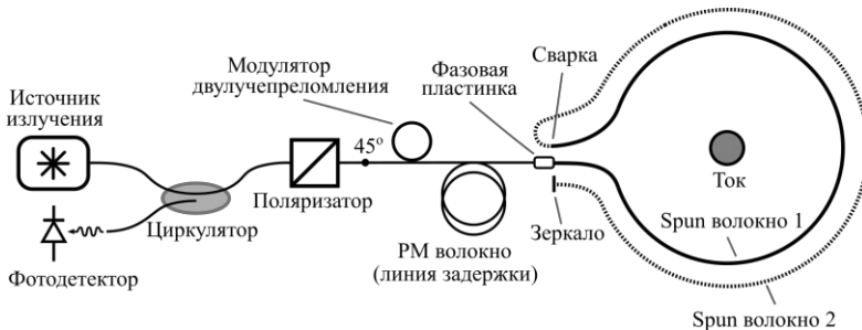
Рис. 1. Схема датчика
