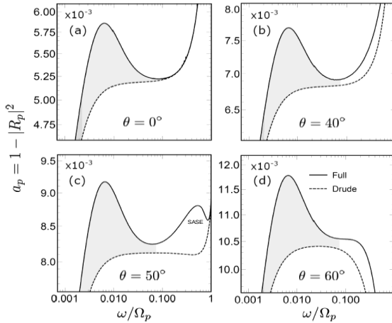
Рис. 1. Спектр способности поглощения a_p для p -поляризованных волн, рассчитанный для значений угла падения \theta = 0^\circ (а), \theta = 40^\circ (б), \theta = 50^\circ (с), и \theta = 60^\circ (д), результаты для модели (1) показаны сплошной линией, приближение Друде показано пунктирной линией, серая и светло-серая заливка представляют частотные диапазоны ASE и SASE
