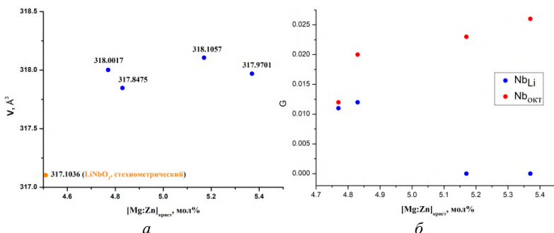
Рис. 1. Концентрационная зависимость объёма элементарной ячейки (а); концентрационная зависимость количества точечных дефектов ( \text{Nb}_{\text{Li}} , \text{Nb}_{\text{Okt}} ) (б)
