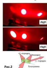
Рис. 2. Вид дифракции на холестерической жидкокристаллической линзе
