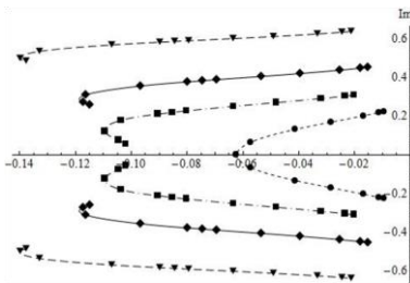
Рис. 2. Зависимость внешних поперечных волновых чисел вытекающих мод (трёх наименьших по модулю) на длине волны \lambda = 1.55 \mu\text{м} (1●), (2▼), (4◆) и одного на \lambda = 2 \mu\text{м} (3■) от значений n_2 = 1 (1), 1.36 (7), 1.453 (12)
