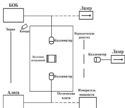
Рис. 1. Экспериментальная установка
