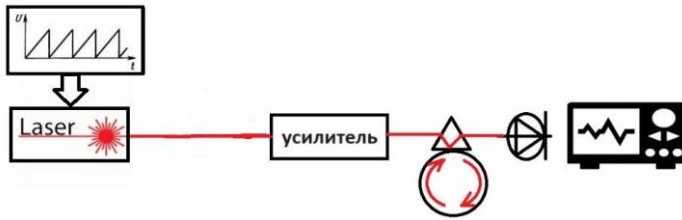
Рис. 1. Схема экспериментальной установки для измерения сдвигов частоты
