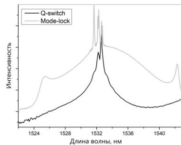
Рис. 2. Спектр лазера при разных режимах генерации
