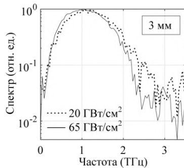
Рис. 2. Терагерцовые спектры при различной интенсивности накачки для кристалла толщиной 3 мм
