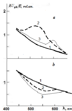
Рис. 1. Спектры фотоЭДС образцов кремния n -типа (а) и p -типа (б)
