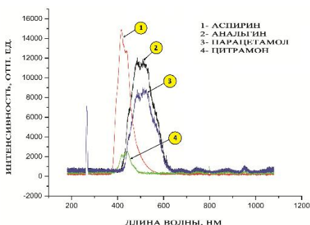
Рис. 2. Фотолуминесцентные спектры лекарственных препаратов (1 – анальгин; 2 – цитрамон; 3 – парацетамол; 4 – аспирин)
