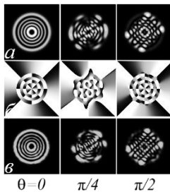
Рис. 1. Теоретические (а) и экспериментальные (б) картины интенсивности и фазы (б) сЛГ-пучка для амплитудного параметра \varepsilon = 1 и некоторых значений фазового параметра \theta
