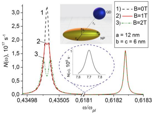
Рис. 1. Спектр люминесценции комплекса «квантовая точка – сфероидальная наночастица»
