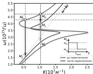
Рис. 1. Дисперсионные кривые при различных значениях плазменной частоты в модели Лоренца
