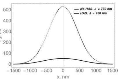
Рис. 2. Зависимость силы давления от координаты x частицы
