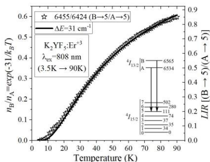
Рис. 1. LIR переходов ( B \rightarrow 5 ) и ( A \rightarrow 5 ) отношения населенностей пв/па в больцмановском распределении
