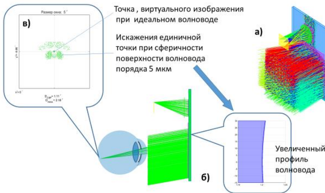
Рис. 1. Моделирование искажений в схеме HMD с наложенными решётками
