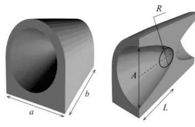
Рис. 2. Модель преломляющей рентгеновской микролинзы с параболическим профилем
