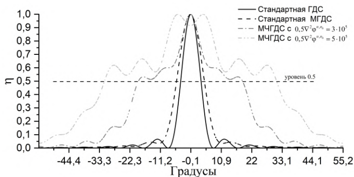
Рис. 1. Угловая селективность стандартной, мультиплексированной и мультиплексированной чирпированной ГДС
