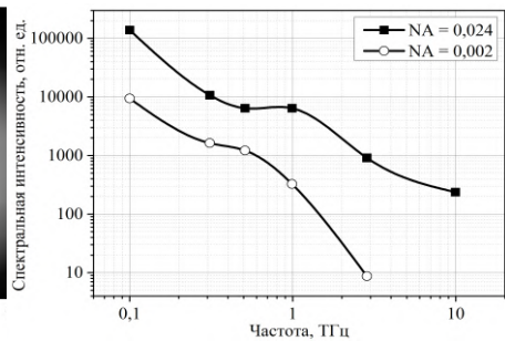
Рис. 2. Спектр плазменного канала в терагерцовом диапазоне при различных числовых апертурах
