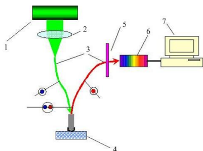
Рис. 1. Схема контактной регистрации флуоресцентных спектров вторичного излучения с двухканальным зондом (1 – лазерное излучение; 2 – оптический зонд; 3 – одноканальные световоды; 4 – исследуемый образец; 5 – абсорбционный фильтр; 6 – миниспектрометр; 7 – управляемый компьютер)
