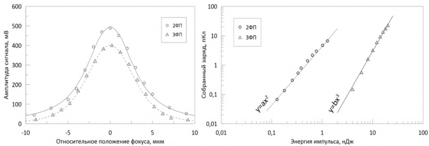
Рис. 1. Зависимость характеристик электрического отклика от смещения фокуса лазерного пучка (слева) и энергии лазерного импульса (справа)
