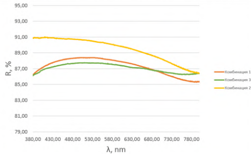
Рис. 1. Спектральные зависимости отражения алюминиевых покрытий, полученных разными методами
