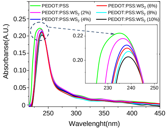
Рис. 1. Спектры поглощения нанокомпозитных плёнок PEDOT:PSS:WS 2
