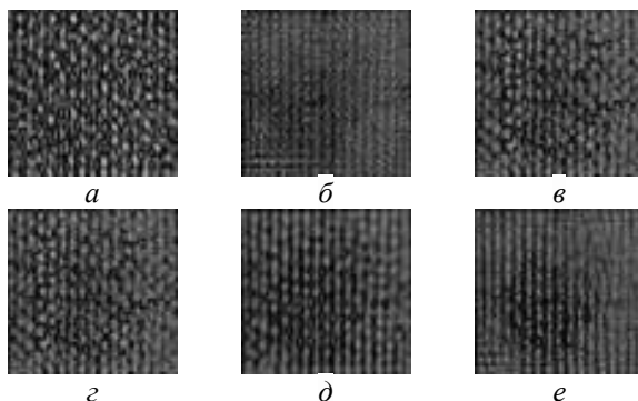
Рис. 1. Фрагменты восстановленных изображений, полученных методом фурье-птихографии, без использования компенсации шумов ( a, z ), с вычетом уровня чёрного ( б, д ), с вычетом минимального значения ( в, е ) для времён экспозиции 50 мс и 500 мс соответственно
