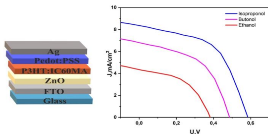
Рис. 1. Структура ячейки (слева), вольтамперная характеристика (справа)
