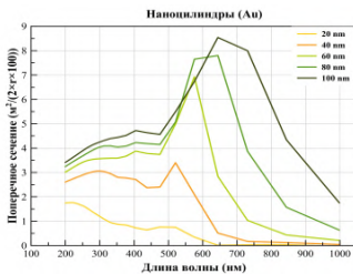
Рис. 1. Максимальные значения напряжённости ( E ) поля золотых наночилиндров распределённые по резонансной длине волны
