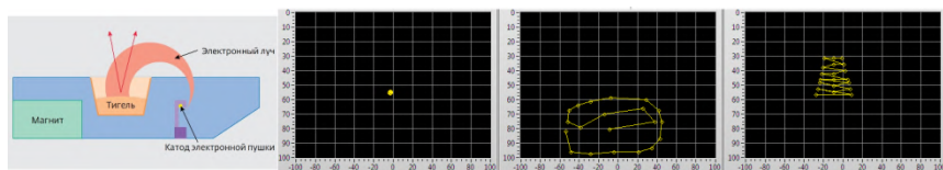
Рис. 1. Схема работы электронно-лучевой пушки и паттерны лучей для материалов: Al, \text{HfO}_2 , \text{Nb}_2\text{O}_5
