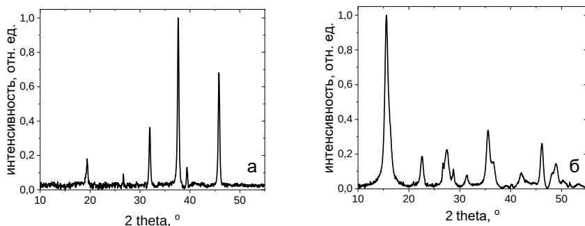
Рис. 1. Дифрактограммы образцов щёлочно-алюмоборатной стеклокерамики с концентрацией \text{B}_2\text{O}_3 30 мол. % (а) и 85 мол. % (б)
