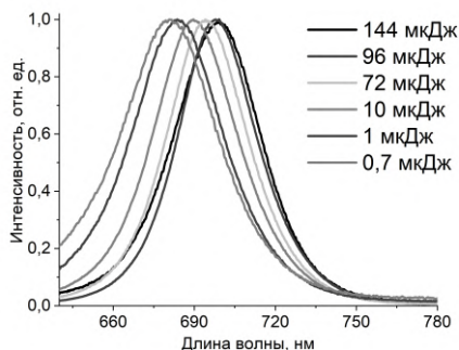
Рис. 1. Спектры люминесценции нанокристаллов \text{CsPbI}_3 в стекле, полученные после воздействия лазерным излучением с различной энергией
