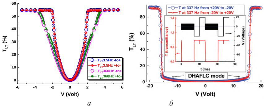
Рис. 1. Безгистерезисные зависимости светопропускания T_{LT} электрооптических ячеек: на основе жидкокристаллического ферриэлектрика FerriLCM-1 [2], толщина слоя которого 2.3 мкм (а); на основе жидкокристаллического антисегнетоэлектрика AFLC-036 [1], толщина слоя которого 1.5 мкм (б), на вставках показаны: частоты знакопеременного электрического напряжения, приложенного к ячейке (а), сверху – частота приложенного напряжения, на вставке в центре, вверх форма приложенного напряжения, внизу форма электрооптического отклика (б)
