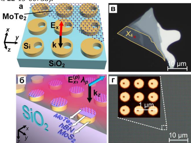
Рис. 1. Изображения усилителя фотолюминесценции на основе MoTe 2 плёнки, размещённой поверх поддерживающей КЗМ метаповерхности (а) и гетероструктурной MoS 2 /hBN/MoTe 2 -метаповерхности в режиме лазерной генерации (б), оптические изображения MoTe 2 флейки с областью X 4 в три атомных слоя (в) и кремниевой метаповерхности, длина волны КЗМ которой соответствует пику фотолюминесценции флейки (г)
