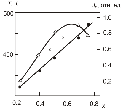
Рис. 2. Зависимости температуры фазового перехода и интенсивности рассеянного света от концентрации бария в кристаллах НБС
