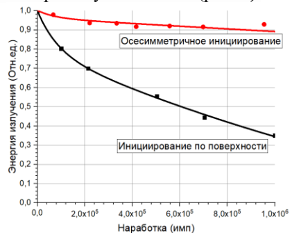
Рис. 2. Срок службы импульсной лампы при различных режимах эксплуатации
