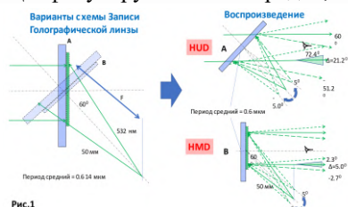
Рис. 1. Варианты конфигурации работы голографических совместителей пучков (beam-combiners) для HUD и HMD-дисплеев
