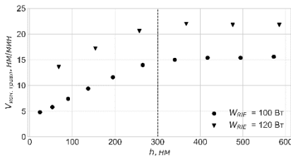
Рис. 1. Профиль скорости ионного травления по глубине
