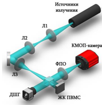
Рис. 1. Эквивалентная схема установки для анализа квазистатических волновых фронтов
