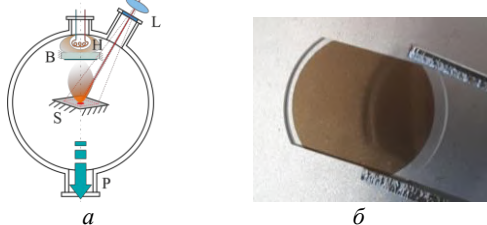
Рис. 1. Принципиальная схема напыления разработанной установки: L – фокусирующая система линз; H – нагреватель; B – подложка; S – мишень; P – система вакуумных насосов (а). и плёнка на подложке (б)
