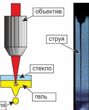
Рис. 2. Схема воздействия и кадр скоростной съёмки со струей геля
