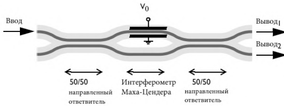
Рис. 1. Оптическая схема модулятора Маха-Цендера
