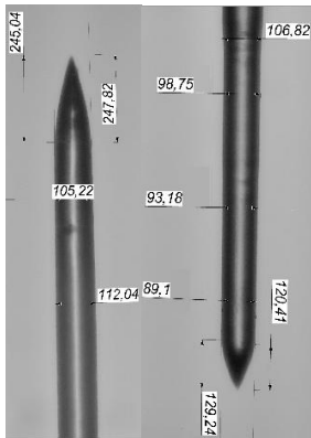
Рис. 1. Линзованные оптические волокна, полученные методом химического травления
