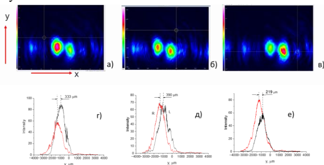
Рис. 1. Профили интенсивностей отражённого пучка: \theta_i = 33.43^\circ (а, г); \theta_i = 33.46^\circ (б, д); \theta_i = 33.49^\circ (в, е)
