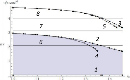
Рис. 3. Частоты отсечки основной (1), первой нечётной (2) и второй чётной (3) мод W-световода, а также нижние границы переходных зон (кривые 4 и 5) в зависимости от n_2 ( 1 \leq n_2 \leq n_3 )
