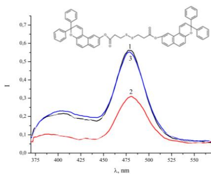
Рис. 2. Спектры флуоресценции (до (1), после УФ-облучения (2) и после последующего видимого облучения (3)) фотохромных нанокомпозитов на основе квантовых точек и бисдифенилбензохромена G620 в толуоле
