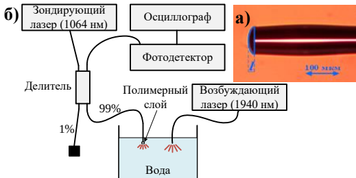
Рис. 1. Снимок волокна с полимером (синяя область) на торце под микроскопом (а), блок-схема экспериментальной установки (б)
