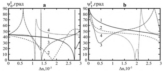
Рис. 2. Зависимость азимутов поляризации прошедшей дифрагированной волны нулевого порядка \psi_0^t (а) и первого порядка \psi_1^t (б) на ГР в слое от амплитуды изменения показателя преломления \Delta n при различных толщинах слоя h : 1 (1), 1.5 (2), 2 (3), 2.5 мм (4) (кристалл GaAs, n_1 = n_3 = 1 , n_2 = 3.18 , \lambda_0 = 1.15 мкм, \varphi_1 = 2^\circ , \psi_0 = 45^\circ )
