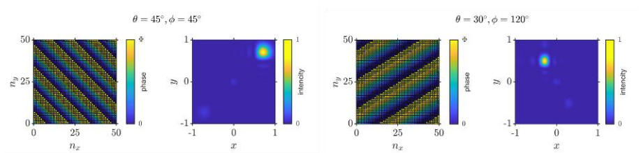
Рис. 2. Распределение фазы вдоль метаповерхности и распределение интенсивности в дальнем поле при различных значениях углов \theta и \phi
