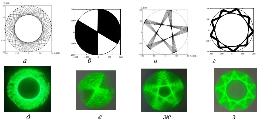
Рис. 1. Расчётные проекции траекторий косых лучей на выходной торец ОВ (а - г), фото распределений интенсивности излучения \lambda = 532 нм на выходном торце КП-СИЭЛ 40 мкм при различных условиях ввода излучения (д - з)
