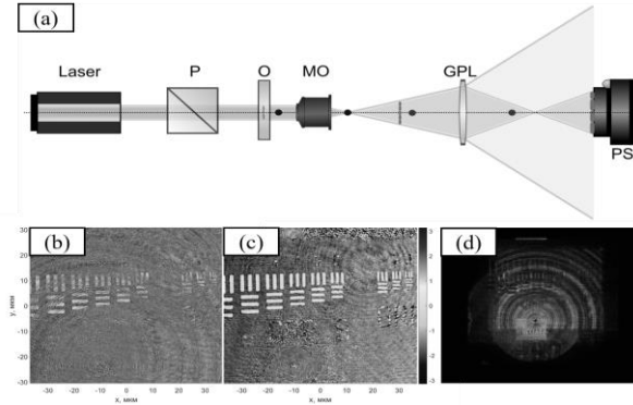
Рис. 1. Схема голографического микроскопа с геометрической фазовой линзой: P – призма Глана–Тейлора, O – плоскость расположения исследуемого объекта, MO – объектив микроскопа, GPL – геометрическая фазовая линза, PS – поляризационный матричный фотодетектор (a); восстановленное фазовое изображение объекта (b); фазовое изображение после фильтрации (c); распределение амплитуды численно распространённого поля, содержащего несколько дифракционных порядков (d)
