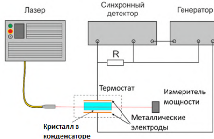
Рис. 1. Блок-схема экспериментальной установки для измерения коэффициентов оптического поглощения методом ПРЛК, отклик кристалла на воздействие радиочастотного поля от генератора регистрируется с помощью измерения напряжения на нагрузочном сопротивлении синхронным детектором
