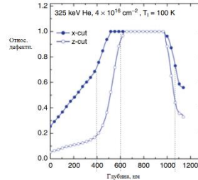
Рис. 2. Распределение дефектов структуры НЛ по глубине (отн.ед. 1.0 – аморфное состояние) [3]
