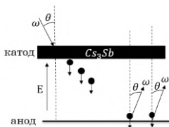
Рис. 1. Схема фотодиода
