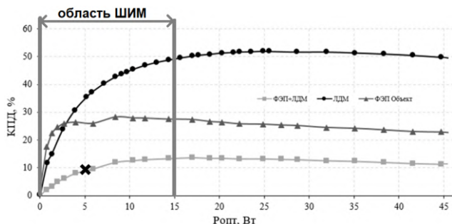
Рис. 1. Зависимость КПД компонентов PoF от оптической мощности: ФЭП объект, ЛДМ и ФЭП+ЛДМ, X – значение, используемое для оценки работы ШИМ – 5 Вт (200 Ом)
