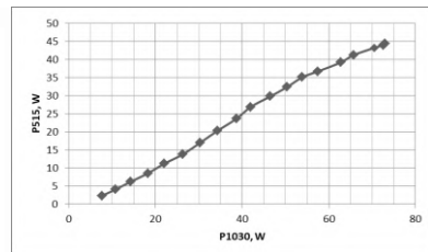
Рис. 2. Ватт-ваттная характеристика генерации второй гармоники
