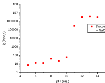
Рис. 1. Кинетика хемилюминесценции люцигенина в зависимости от pH раствора
