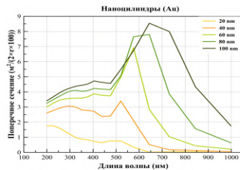
Рис. 2. Нормированные значения поперечного сечения экстинкции золотых наночилиндров распределённые по длине волны
