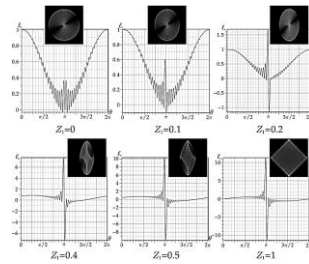
Рис. 2. Осцилляции ОУМ \varepsilon_z(\theta) при вариации \theta -управляющего параметра аСЛГ пучка с n = 20 , \ell = 1 , \varepsilon = 1 на различных длинах пучка Z_1 , выноски: картины интенсивности для первого всплеска ОУМ
