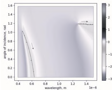
Рис. 4. Эволюция точек фазовой сингулярности для s-поляризации
