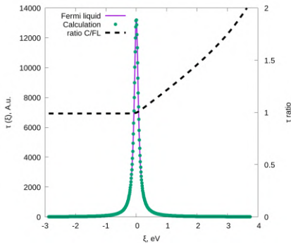
Рис. 1. Рассчитанное время релаксации в зависимости от энергии квазичастицы ( F = 3.0 эВ, k_F = 0.5\pi/a , T = 300 K), штриховой линией показано сравнение с формулой из теории ферми-жидкости
