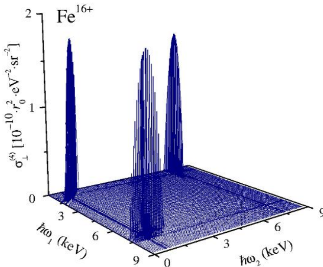
Рис. 1. Четырежды дифференциальное сечение расщепления фотона ионом \text{Fe}^{16+} для \perp -схемы эксперимента. Энергия падающего фотона \hbar\omega = 9 \text{ keV} [1], \hbar\omega_{1,2} – энергии рассеянных фотонов, энергия порога ионизации 1s^2 -оболочки I_{1s} = 7.7 \text{ keV} , естественная ширина распада 1s – вакансии \Gamma_{1s} = 1.046 \text{ eV} [2]
