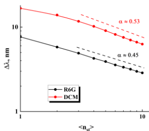
Рис. 2. Зависимости полуширины спектров флуоресценции от среднего числа актов индуцированной эмиссии
