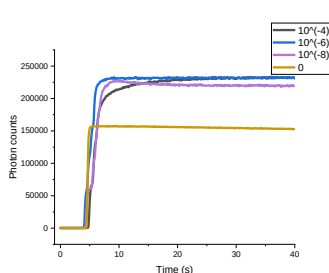
Рис. 2. Кинетика хемилюминесценции люцигенина в зависимости от концентрации наночастиц
