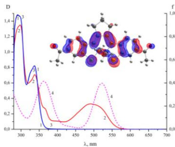
Рис. 2. Спектры электронного поглощения (до (1), после УФ-облучения (2) и после последующего видимого облучения (3)) фотохромного диарилэтена ДАЭ2 в толуоле, расчётные спектры электронного поглощения (4) и формы граничных МО, участвующих в формировании спектра поглощения ДАЭ2
