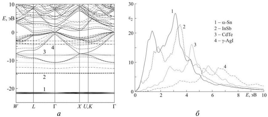
Рис. 1. Зонные структуры (а) и спектры мнимой части диэлектрической функции (б)
