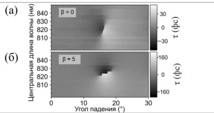
Рис. 2. \lambda - \theta зависимости задержки \tau лазерных импульсов для \beta = 0 (а) и \beta = 5 (б)
