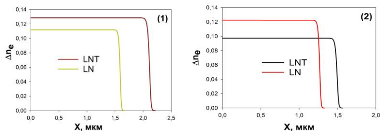
Рис. 1. Профили оптических волноводов (ПО 190 °C-2 ч.): X-срез (1) и Z-срез (2)
