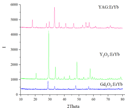
Рис. 1. Дифрактограмма наноккомпозитов YAG:Er/Yb, Y_2O_3 :Er/Yb и Gd_2O_3 :Er/Yb
