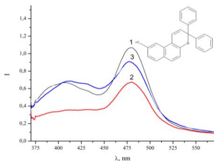
Рис. 1. Спектры флуоресценции (до (1), после УФ-облучения (2) и после последующего видимого облучения (3)) фотохромных нанокомпозитов на основе квантовых точек и дифенилбензохромена G618 в толуоле
