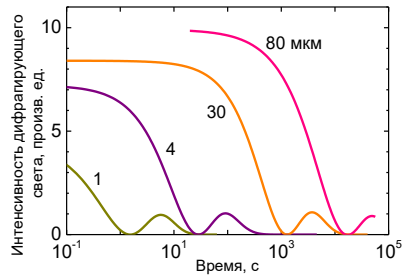
Рис. 2. Кривые релаксации фотоиндуцированных решёток с пространственными периодами 1 - 80 мкм, записанных с использованием фотовосстановления КХ
