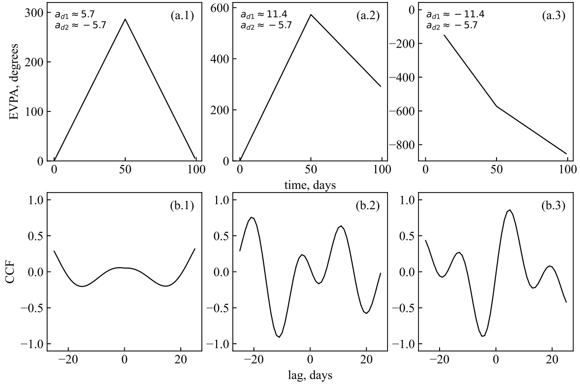
Рис. 4. Случаи n = 2 . На верхней панели (a.1), (a.2), (a.3) изображены различные случаи нескольких участков монотонного изменения EVPA с разной скоростью. Скорости вращений a_{dn} указаны в градусах в сутки. На нижней панели (b.1), (b.2), (b.3) приведены соответствующие оценки кросс-корреляции параметров q и u .
