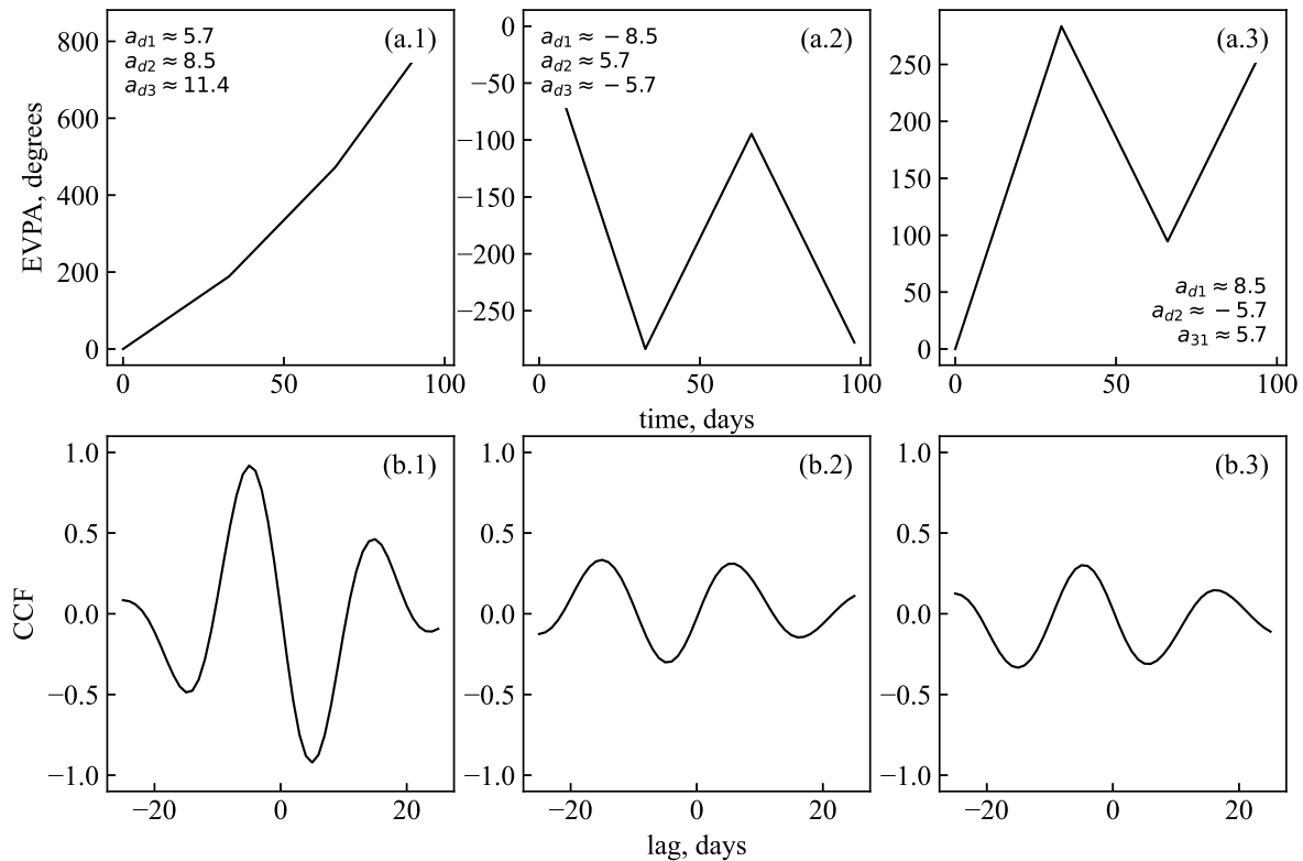
Рис. 5. Случаи n = 3 . На верхней панели (a.1), (a.2), (a.3) изображены различные случаи нескольких участков монотонного изменения EVPA с разной скоростью. Скорости вращений a_{dn} указаны в градусах в сутки. На нижней панели (b.1), (b.2), (b.3) приведены соответствующие оценки кросс-корреляции параметров q и u .
