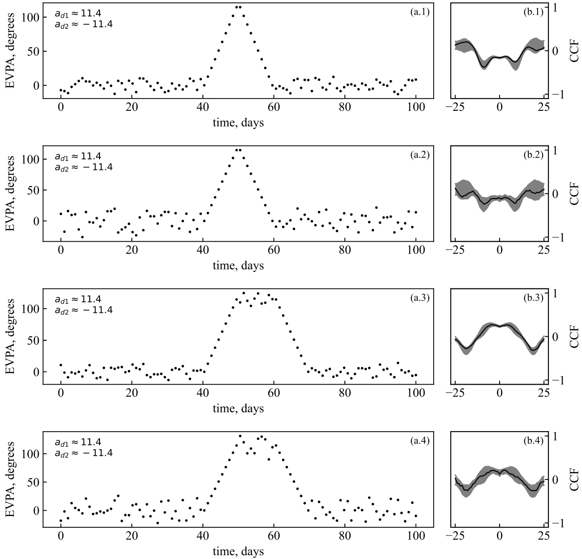
Рис. 9. События двойного вращения со сменой направления, которое предваряется и затем сменяется участками случайного равновероятного изменения EVPA. Слева приведены кривые EVPA для случаев последовательного двойного вращения с изменением направления (a.1), (a.2) и двойного вращения с изменением направления, прерываемого участком равновероятного изменения EVPA (a.3), (a.4). Пары реализаций отличаются амплитудой случайных равновероятных изменений EVPA. Справа приведены соответствующие оценки (b.1), (b.2), (b.3), (b.4) кросс-корреляционной функции параметров q и u . Скорости вращений a_{dn} указаны в градусах в сутки.
