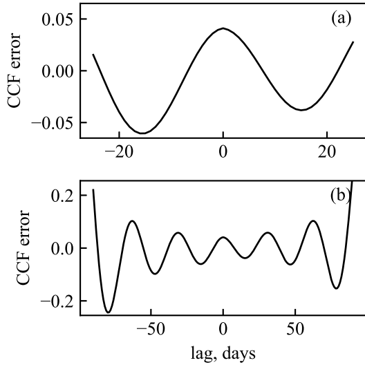
Рис. 2. Отклонения используемой численной оценки кросс-корреляционной функции от значений, полученных аналитически, для случая монотонного изолированного вращения. На панели (a) приведены отклонения оценки для малых задержек, соответствующих панели (b) рис. 1. На панели (b) показано поведение отклонений с увеличением диапазона рассматриваемых задержек.
