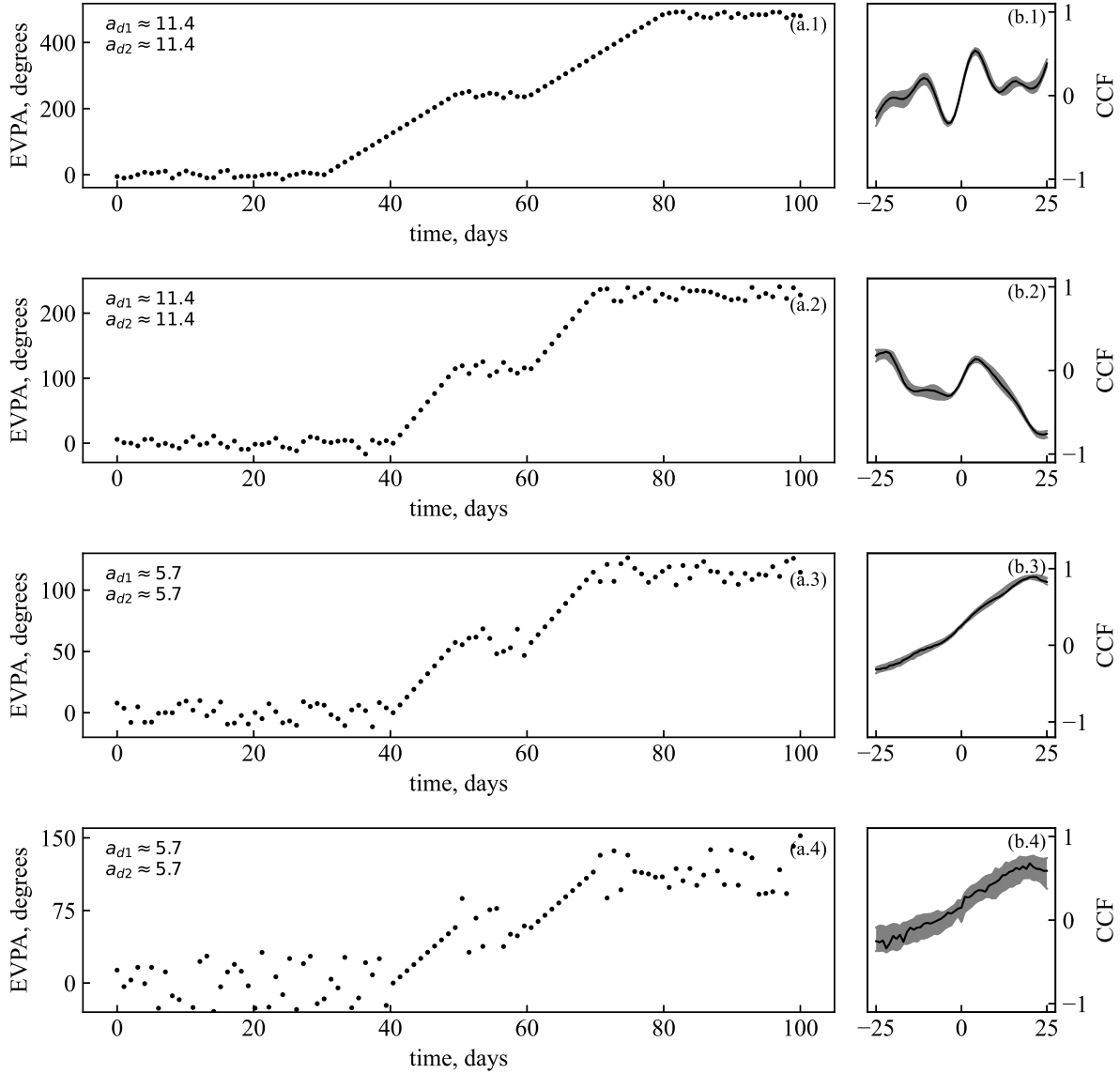
Рис. 8. События двойного вращения по часовой стрелке, которое предваряется и затем сменяется участками случайного равновероятного изменения EVPA. Слева приведены кривые EVPA для случаев длительного двойного вращения (a.1), двойного вращения (a.2), медленного вращения (a.3), медленного вращения с участками случайного равновероятного изменения EVPA с большой амплитудой. Справа приведены соответствующие оценки (b.1), (b.2), (b.3), (b.4) кросс-корреляционной функции параметров q и u . Скорости вращений a_{dn} указаны в градусах в сутки.
