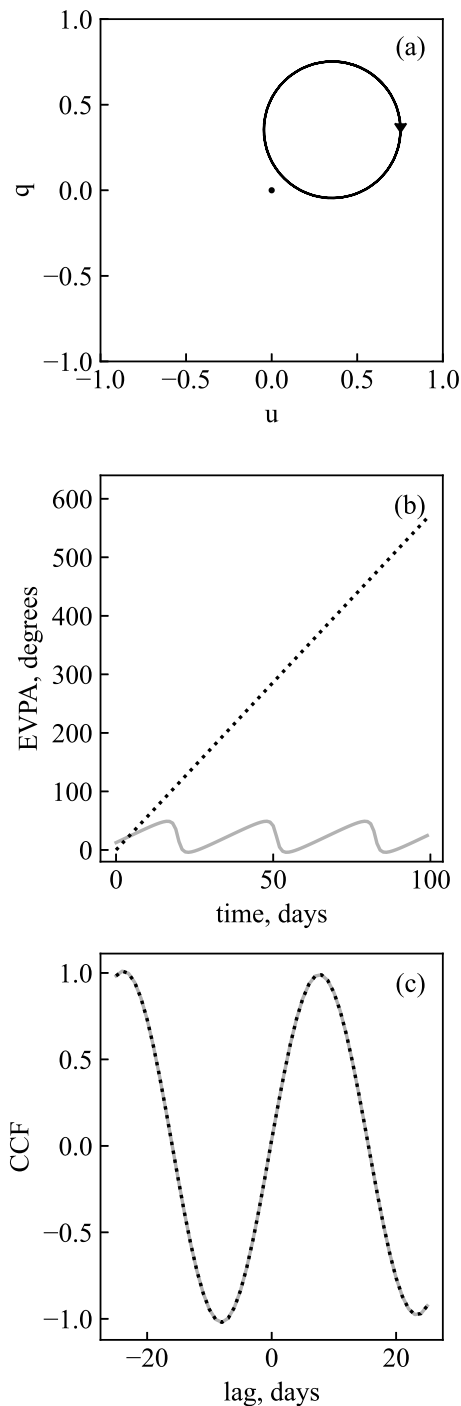
Рис. 3. Простейший случай двух источников. (a) вид плоскости q - u для q_{obs} - u_{obs} , стрелкой указано направление вращения; (b) изменение EVPA наблюдаемое obs (линией) и принадлежащее переменному var (пунктиром) источнику; (c) оценки кросс-корреляции параметров q_{obs} - u_{obs} (линией) и q_{var} - u_{var} (пунктиром).
