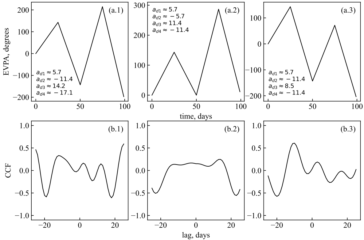
Рис. 6. Случаи n = 4 . На верхней панели (a.1), (a.2), (a.3) изображены различные случаи нескольких участков монотонного изменения EVPA с разной скоростью. Скорости вращений a_{dn} указаны в градусах в сутки. На нижней панели (b.1), (b.2), (b.3) приведены соответствующие оценки кросс-корреляции параметров q и u .
