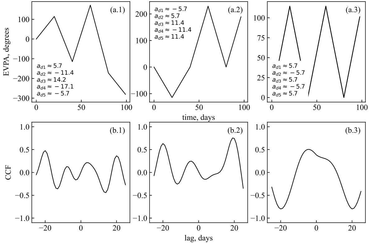
Рис. 7. Случаи n = 5 . На верхней панели (a.1), (a.2), (a.3) изображены различные случаи нескольких участков монотонного изменения EVPA с разной скоростью. Скорости вращений a_{dn} указаны в градусах в сутки. На нижней панели (b.1), (b.2), (b.3) приведены соответствующие оценки кросс-корреляции параметров q и u .
