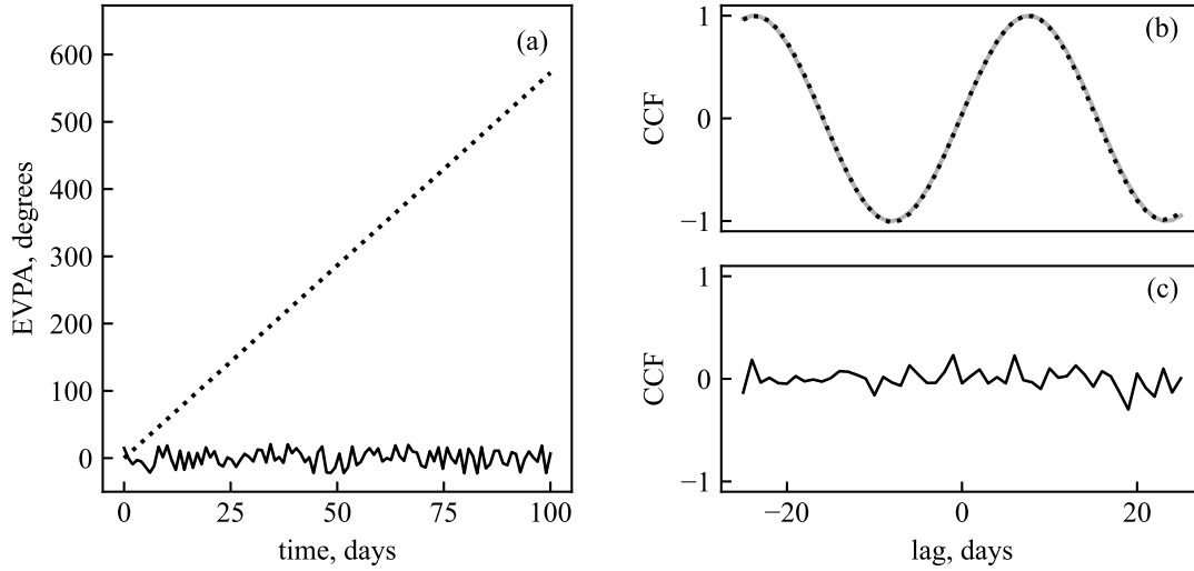
Рис. 1. Простейшие случаи изменения EVPA. На панели (a) показаны «наблюдаемые» значения EVPA: пунктиром отмечен случай монотонного вращения EVPA со скоростью a_d \approx 5.7 градусов в сутки, сплошной линией – случай равновероятного изменения EVPA. На панели (b) показана кросс-корреляционная функция для случая монотонного изолированного вращения (линией отмечены значения полученные аналитически, пунктиром – численная оценка), на панели (c) изображена кросс-корреляция параметров q и u случайного равновероятного изменения EVPA.
