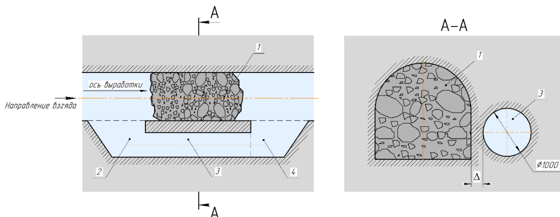
Рис. 2. Схема расположения горизонтальной спасательной скважины в обход завала: 1 – завал, 2 – камера входа, 3 – спасательная скважина, 4 – камера выхода
