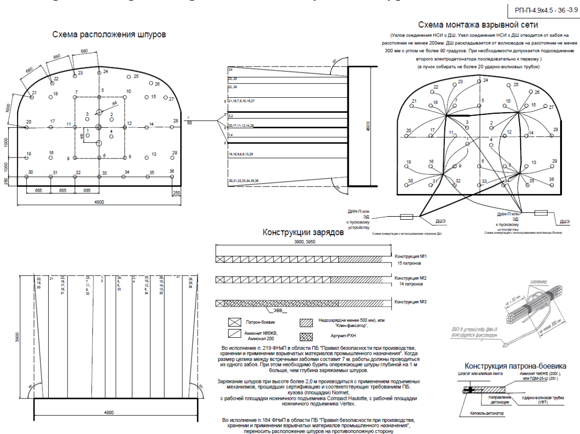
Рис. 1. Паспорт бурения для забоя с коэффициентом крепости f=4
