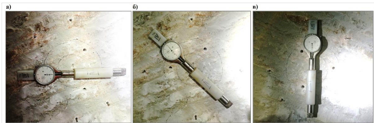
Рис. 3. Процесс измерения деформаций на стенке горной выработки механическим тензометром до бурения разгрузочной скважины:
