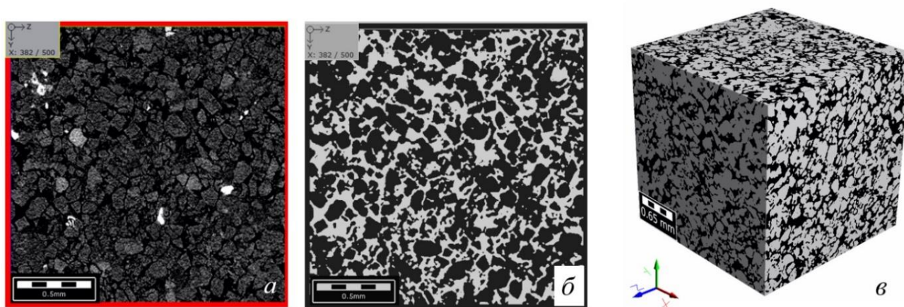
Рис. 1. Проекция, полученная после сканирования и реконструкции (а); результат сегментации (б); пример итоговой 3D модели горной породы (в)
