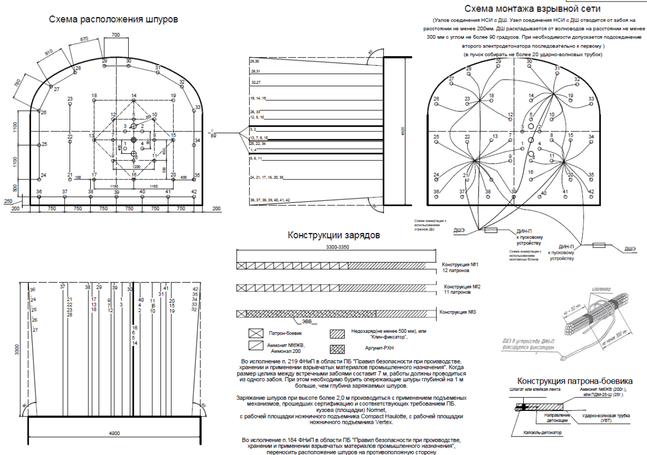
Рис. 2. Паспорт бурения для забоя с коэффициентом крепости f=10
