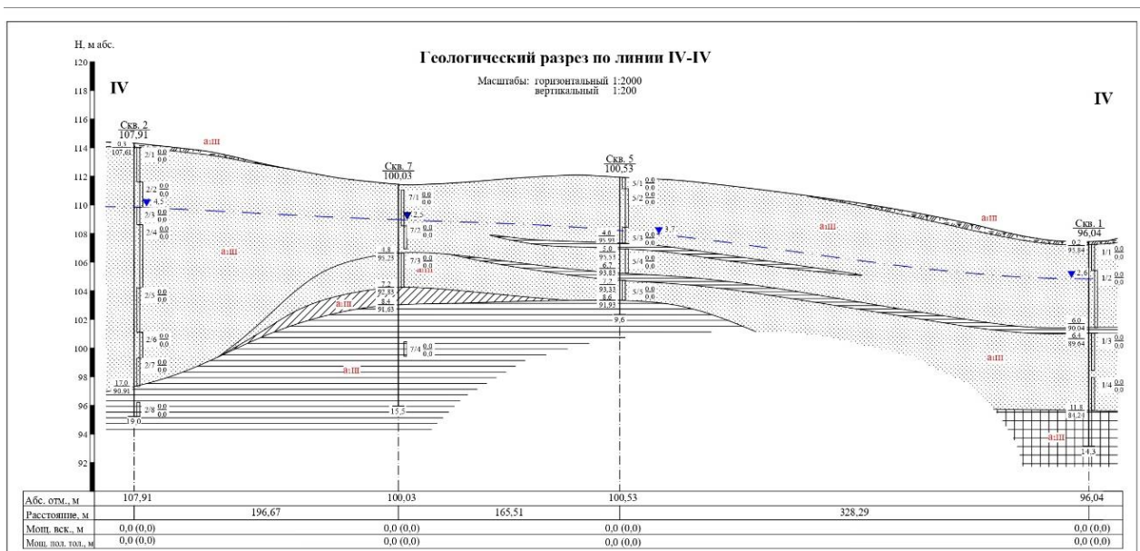
Рис. 2. Геологический разрез по линии скважин 2-7-5-1
