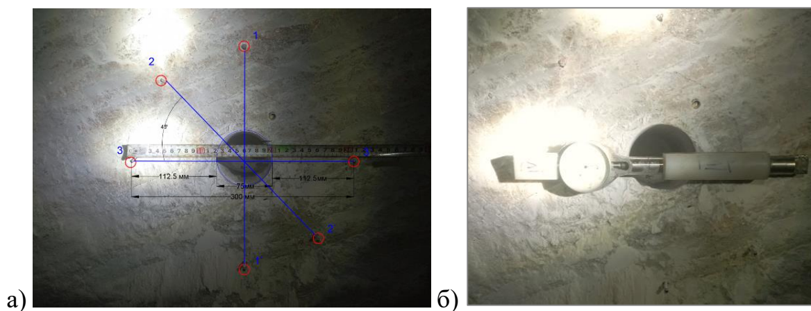
Рис. 4. Реализация расчетной схемы (а) и процесс измерения деформаций на стенке горной выработки механическим тензOMETром после бурения разгрузочной щели по базе 1-1' (б)
