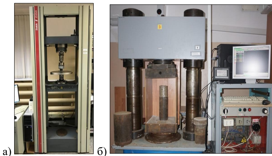
Рис. 2. Оборудование для проведения экспериментов по определению физико-механических свойств пород: а – электромеханический пресс Zwick/Z250; б – гидравлический пресс ИП 2000
