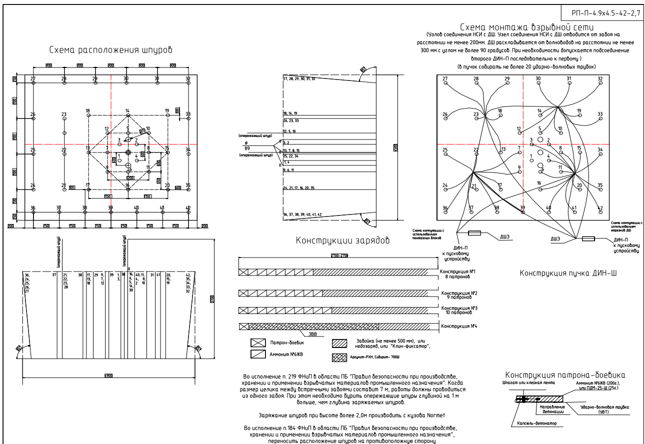
Рис. 3. Паспорт бурения с глубиной шпура 2,7 метров
