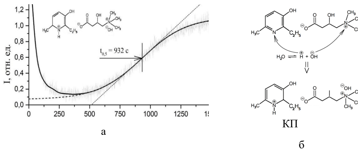
Рисунок 1. (а) Кинетическая кривая тушения хемилюминесценции ХЛ, сопровождающей инициированное АИБН окисление этилбензола (20% в хлорбензоле), карнитинатом 2-этил-6-метил-3-гидроксипиридиния: [КП]_0=5,2\cdot 10^{-6}\text{М} ; W_i=1,12\cdot 10^{-8}\text{М}\cdot\text{с}^{-1} ; активатор [ДБА]=5\cdot 10^{-3}\text{М} ; 50^\circ\text{С} , t_{0,5} – период торможения окисления. (б) Схема образования КП - гидрата карнитината 2-этил-6-метил-3-гидроксипиридиния
