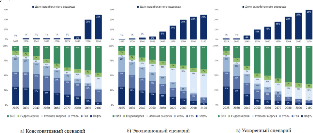
Рис. 2. Сценарии развития водородной энергетики, основанной на различной структуре мирового энергобаланса, в период с 2025 по 2100 гг.
