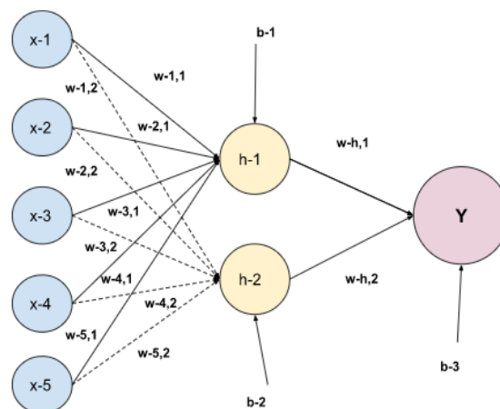
Рис. 1. Схематичное представление архитектуры нейронной сети
