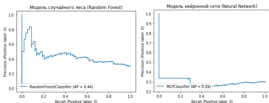
Рис. 2. Оценка метрики Precision-Recall AUC для используемых моделей
