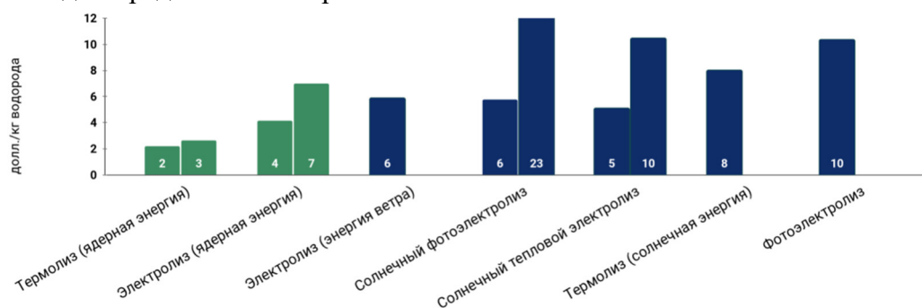
Рис. 1. Диапазон стоимости водорода при использовании различных технологий производства
