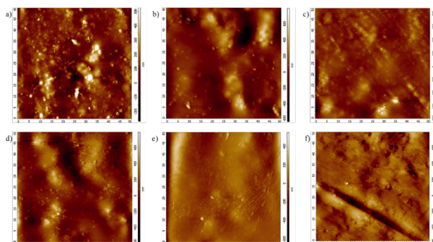
Рисунок 1 - Сканы поверхности образцов: а) Ag-TiO 2 ; б) CuO-FeCuO; в) ZnO-FeZnO; д) ZnTi 2 O 4 -TiO 2 ; е) ZnTi 2 O 4 -ZnO; ф) Bioplast-52
