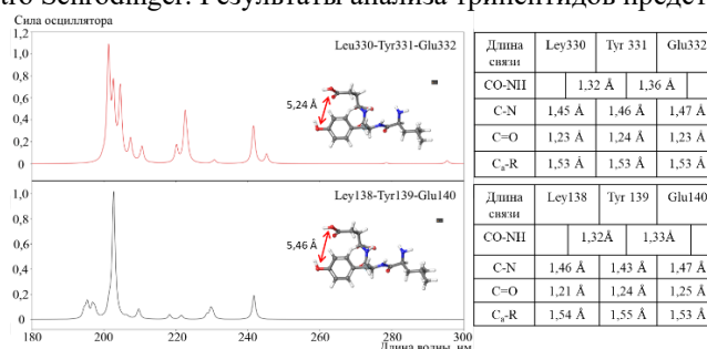
Рисунок 1. Электронные спектры поглощения трипептидов лейцин-тирозин-глутаминовая кислота в молекуле сывороточного альбумина быка
