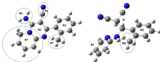
Рисунок 1. Геометрическое строение молекул I (слева) и II (справа)
