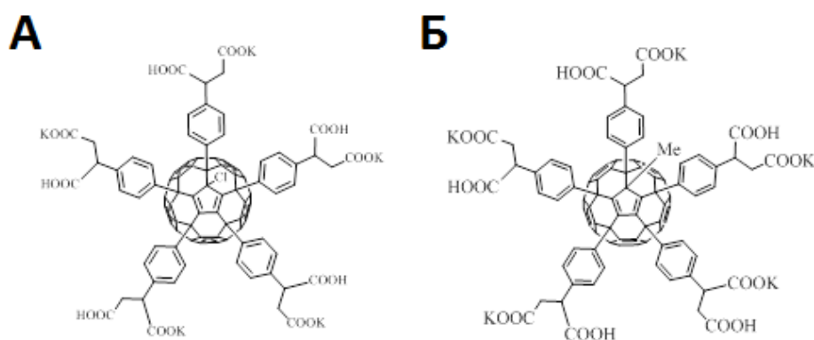
Рисунок 1. Молекулярная формула соединений Ф-225 (А) и Ф-231 (Б)
