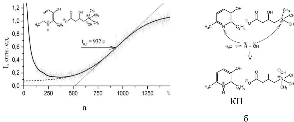
Рисунок 1. (а) Кинетическая кривая тушения хемилюминесценции ХЛ, сопровождающей инициированное АИБН окисление этилбензола (20% в хлорбензоле), карнитинатом 2-этил-6-метил-3-гидроксипиридиния: [\text{КП}]_0=5,2\cdot 10^{-6}\text{M} ; W_i=1,12\cdot 10^{-8}\text{M}\cdot\text{c}^{-1} ; активатор [\text{ДБА}]=5\cdot 10^{-3}\text{M} ; 50^\circ\text{C} , t_{0,5} – период торможения окисления. (б) Схема образования КП - гидрата карнитината 2-этил-6-метил-3-гидроксипиридиния
