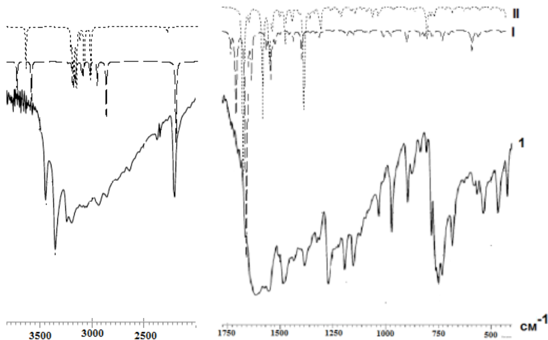
Рисунок 2. ИК спектры: экспериментальный (1) и теоретические (I, II)
