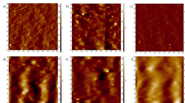
Рисунок 2 - Сканы поверхности образцов: а) Bioplast-52; б) Основа «Bioplast-52» + Ag-TiO 2 ; в) Основа «Bioplast-52» + CuO-Cu 2 O-CuFe 2 O 4 ; д) РК-Marine; е) РК-Marine + Ag-TiO 2
