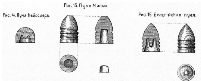
Илл. 3 Пуля типа Минье
