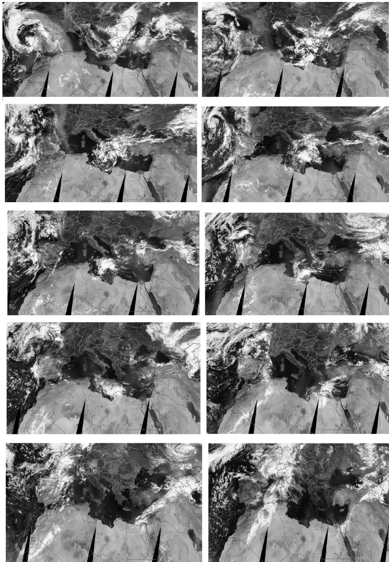
Рис. 3. Снимки облачности в период развития циклона Даниэль с 4 по 13 сентября 2023 года
