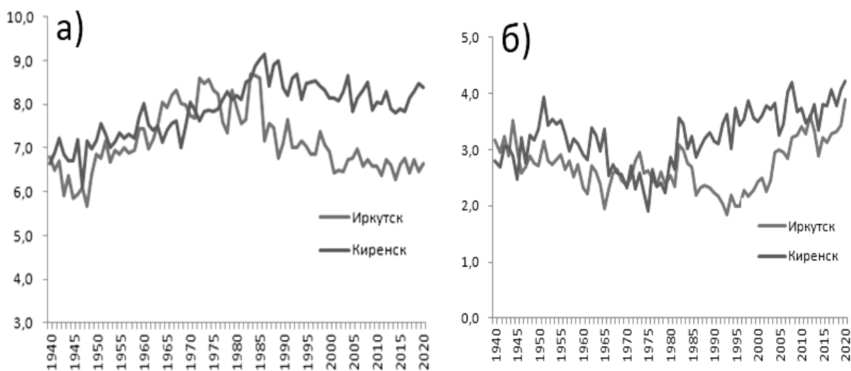
Рис. 3. Изменение количества общего количества облаков (а) и количества нижней облачности (б) в Иркутске и Киренске в 1940-2020 гг.
