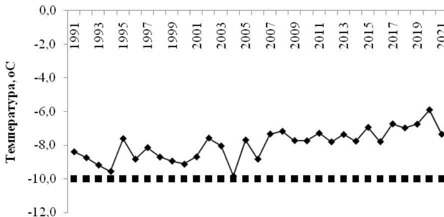
Рис. 1. Среднегодовая температура воздуха города Якутска
