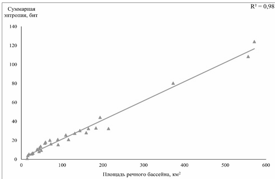
Рис. 2. График связи площади бассейна и суммарной энтропии
