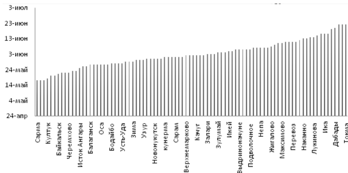
Рис. 1. Средние даты наступления последних заморозков на метеорологических станциях Иркутской области за 1950-2020 годы
