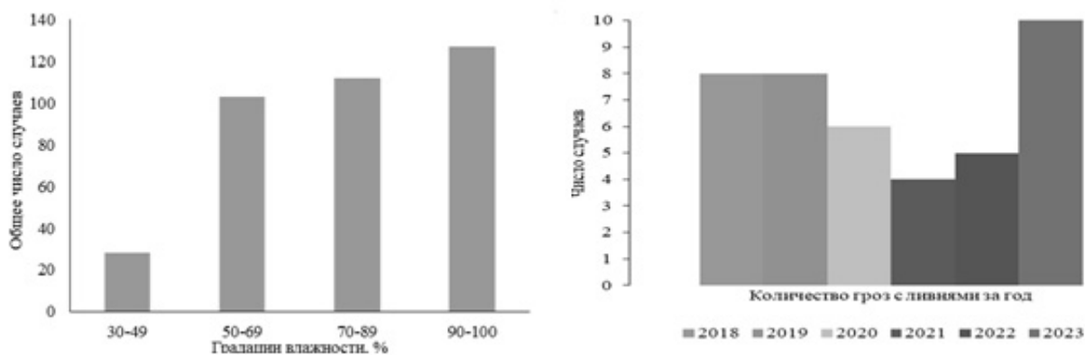
Рис. 2. Распределение градаций относительной влажности воздуха и количества гроз с ливнями в Иркутске в летние месяцы 2018-2023 гг.
