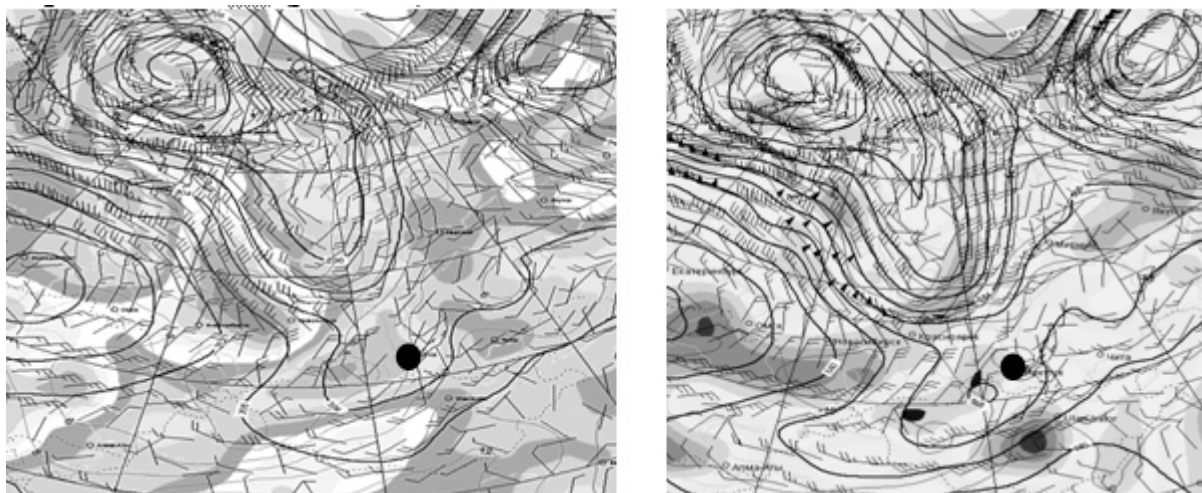
Рис. 2. Карта АТ-700 гПа (слева) и АТ-500 гПа (справа) за 00:00 ВСВ 15.07.2020 г.
