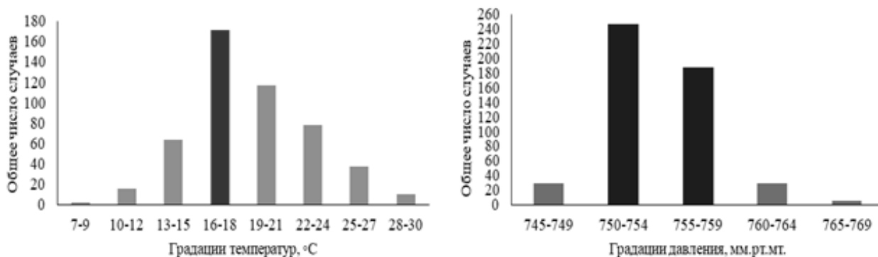
Рис. 1. Распределение градаций температуры воздуха и атмосферного давления при грозах в Иркутске в летние месяцы 2018-2023 гг.
