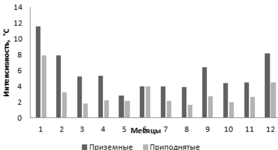
Рис. 3. Средняя интенсивность приземных и приподнятых инверсий в 2021 году в Енисейске
