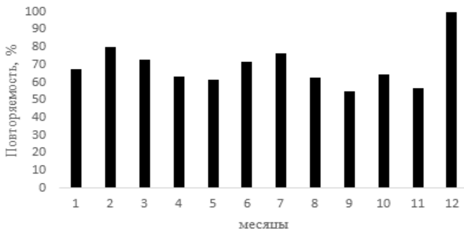
Рис. 1. Повторяемость общего количества инверсий в 2021 году в Енисейске
