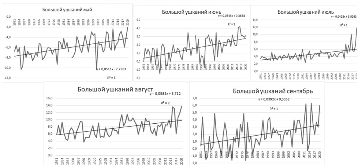
Рис. 3. Изменение значений абсолютного минимума температур на метеорологической станции Большой Ушканий за 1950-2020 годы
