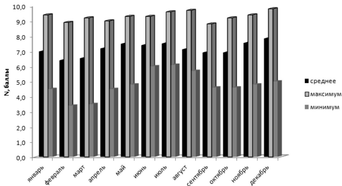
Рис. 1. Годовой ход общего количества облаков в Иркутске в 1940-2020 гг.
