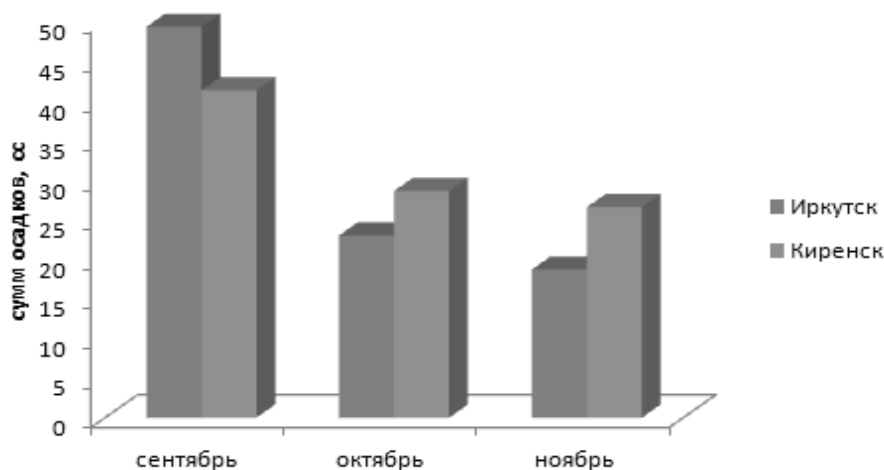
Рис. 1. Средние значения сумм атмосферных осадков в осенние месяцы в Иркутске и Киренске за период 1892-2023 гг.
