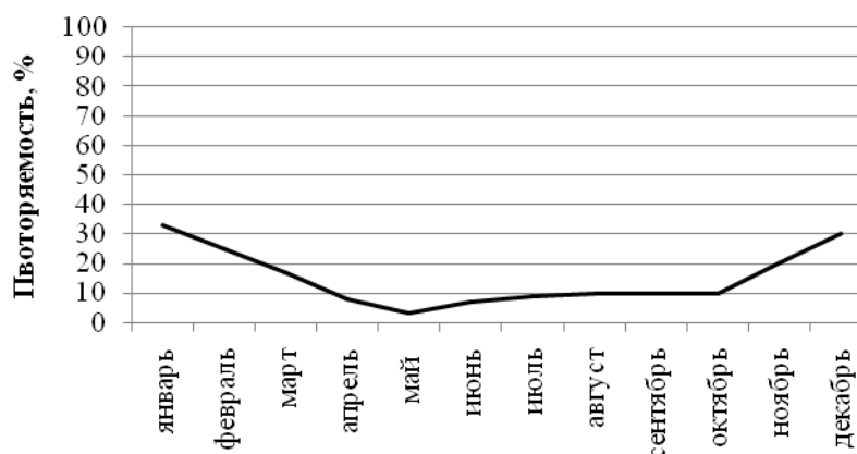
Рис. 3. Повторяемость штилей, %
