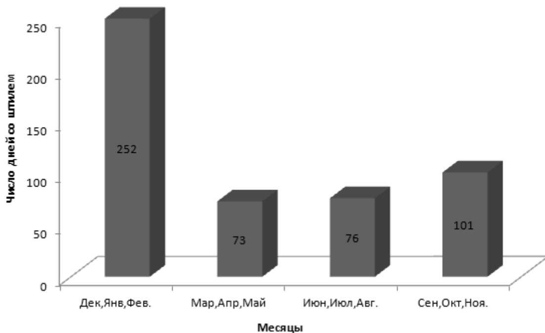
Рис. 2. Повторяемость штилей в районе аэродрома Абакан в 2009-2022 гг.
