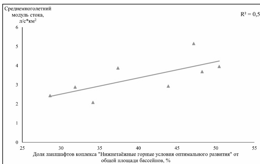
Рис. 6. График связи между долями комплекса ландшафтов «Нижнетаёжные горные условия оптимального развития» и среднемноголетним модулем стока
