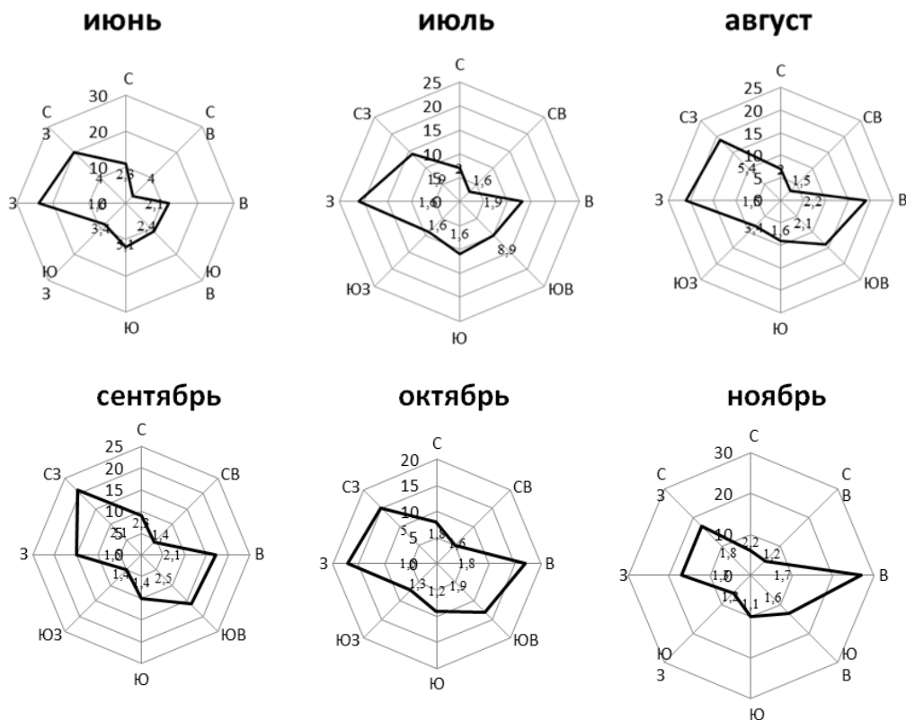
Рис. 1. Повторяемость направлений ветра города Братска
