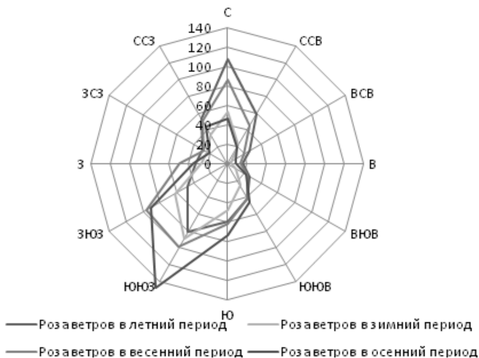
Рис. 1. Роза ветров аэродрома Абакан в 2009-2022 гг.
