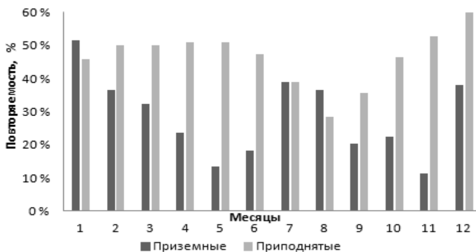
Рис. 2. Повторяемость приземных и приподнятых инверсий в 2021 году в Енисейске
