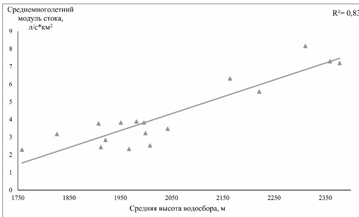
Рис. 4. График связи средней высоты водосбора и среднемноголетнего модуля стока
