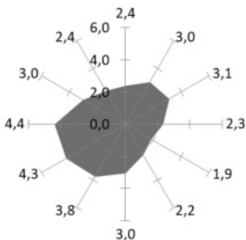
Рис. 2. Годовая роза ветров на аэродроме Киренск в 2006-2020 гг.
