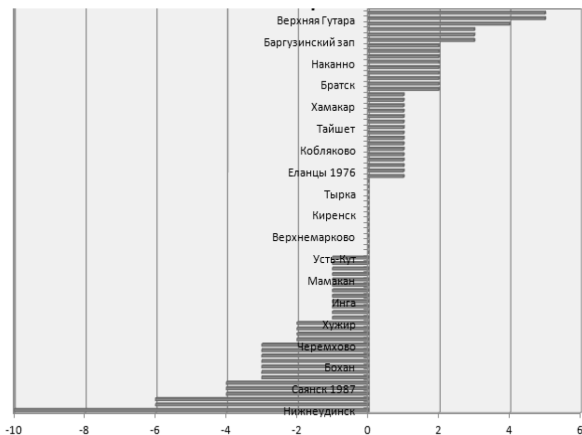
Рис. 2. Разности средних значений относительной влажности воздуха метеорологических станциях Иркутской области в январе за период 2000-2020 гг. по сравнению с 1970-1999 гг.
