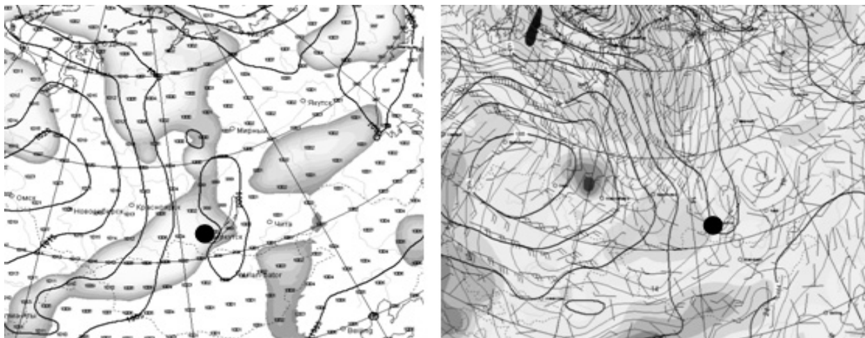
Рис. 3. Карта уровень Земли (слева) и АТ-850 гПа (справа) за 00:00 ВСВ 15.07.2020 г.
