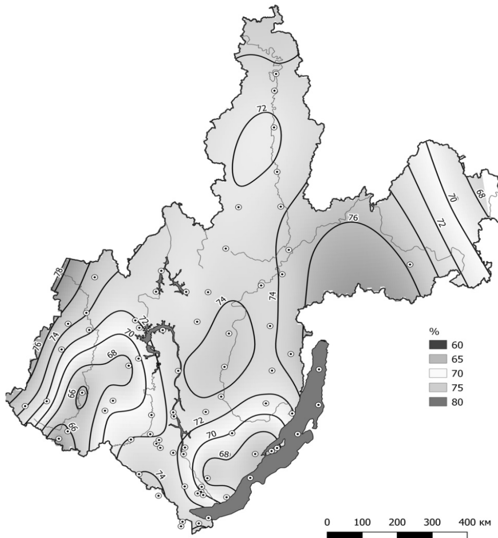
Рис. 1. Средние годовые значения относительной влажности воздуха в Иркутской области в 2000-2020 гг.
