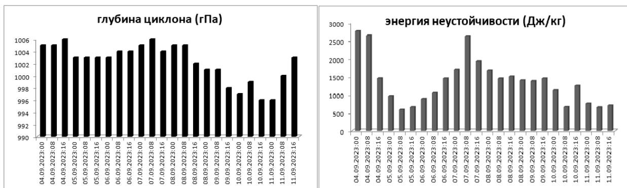
Рис. 1. Изменение давления и потенциальной энергии конвективной неустойчивости в циклоне Даниэль с 4 по 11 сентября 2023 года
