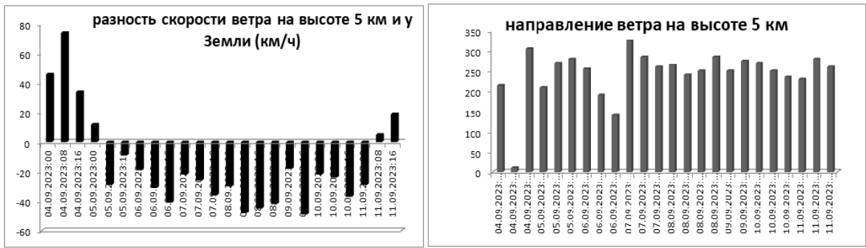
Рис. 2. Изменение характеристик ветра в циклоне Даниэль с 4 по 11 сентября 2023 года
