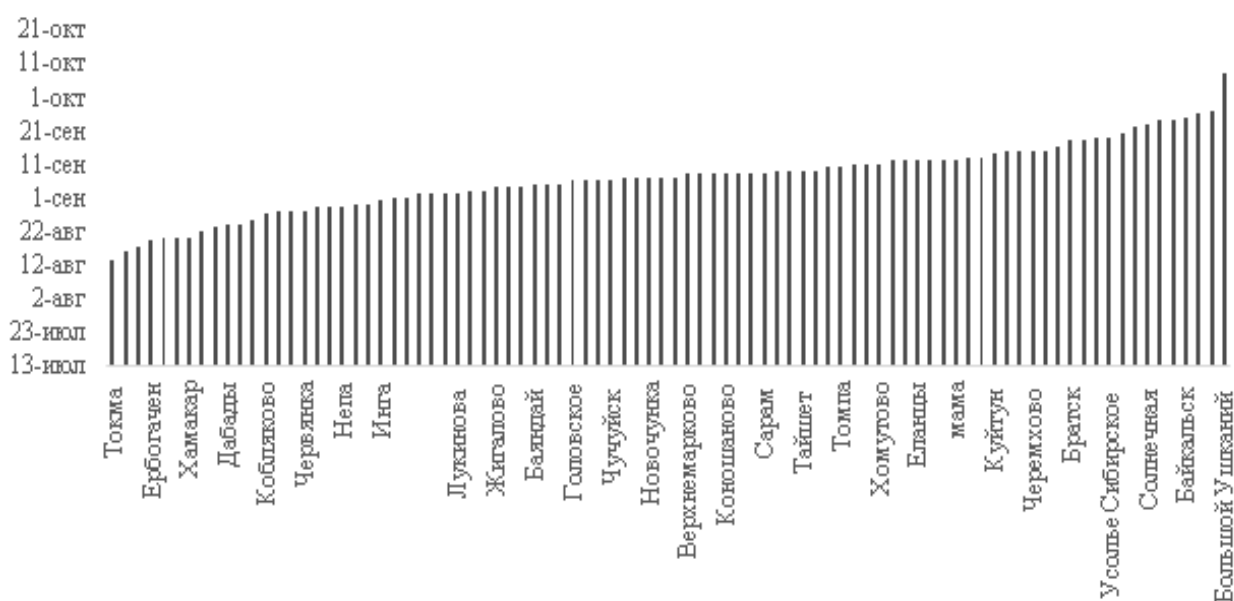
Рис. 2. Средние даты наступления первых заморозков на метеорологических станциях Иркутской области за 1950-2020 годы
