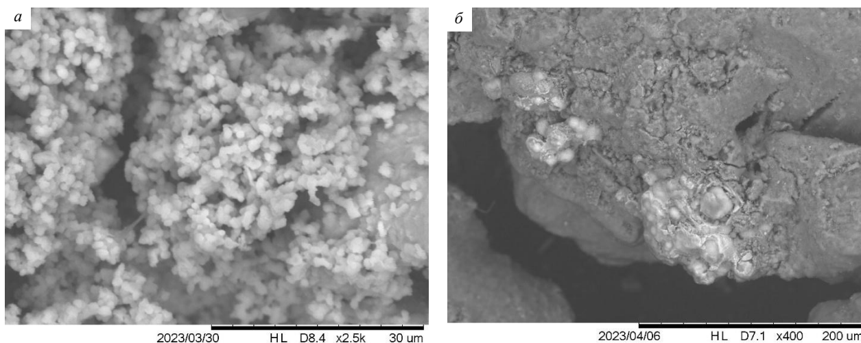
Рис.4. Минеральные фазы железа в донных осадках р. Карагайлы у отвалов Сибайского карьера: а – гидроксиды железа (в районе сброса кислых карьерных вод); б – железомарганцевые образования (светлый оттенок) с Zn, Cu и Co на фоне глинистой матрицы (темный оттенок)
