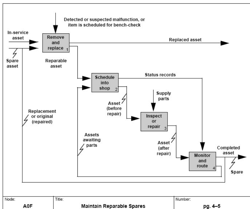
Рисунок 1.1 – Пример диаграммы в нотации IDEF0 (функциональная модель процесса)
