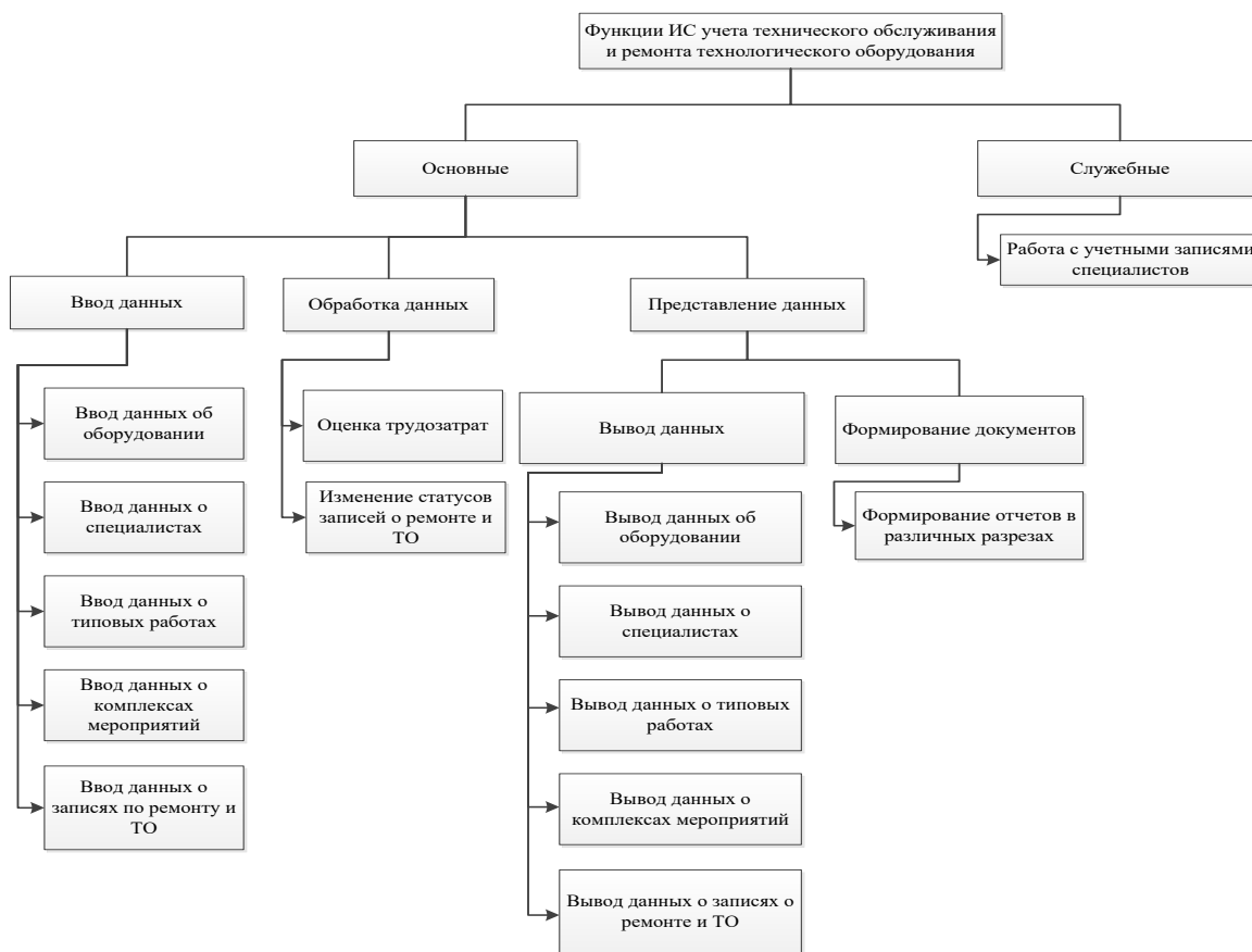
Рисунок 1.7 – Дерево функций информационной системы учета технического обслуживания и ремонта технологического оборудования цеха газоконденсатного промысла
