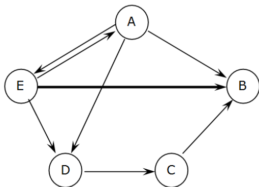
Рис. 2. Добавление ребра при улучшении через вершину А
