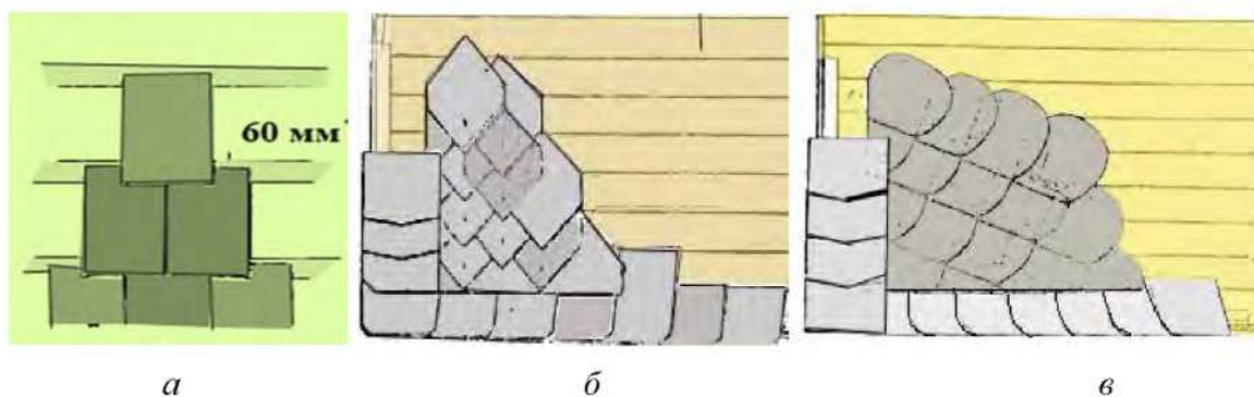
Рисунок 3 - Методы укладки сланцевой черепицы [1]
