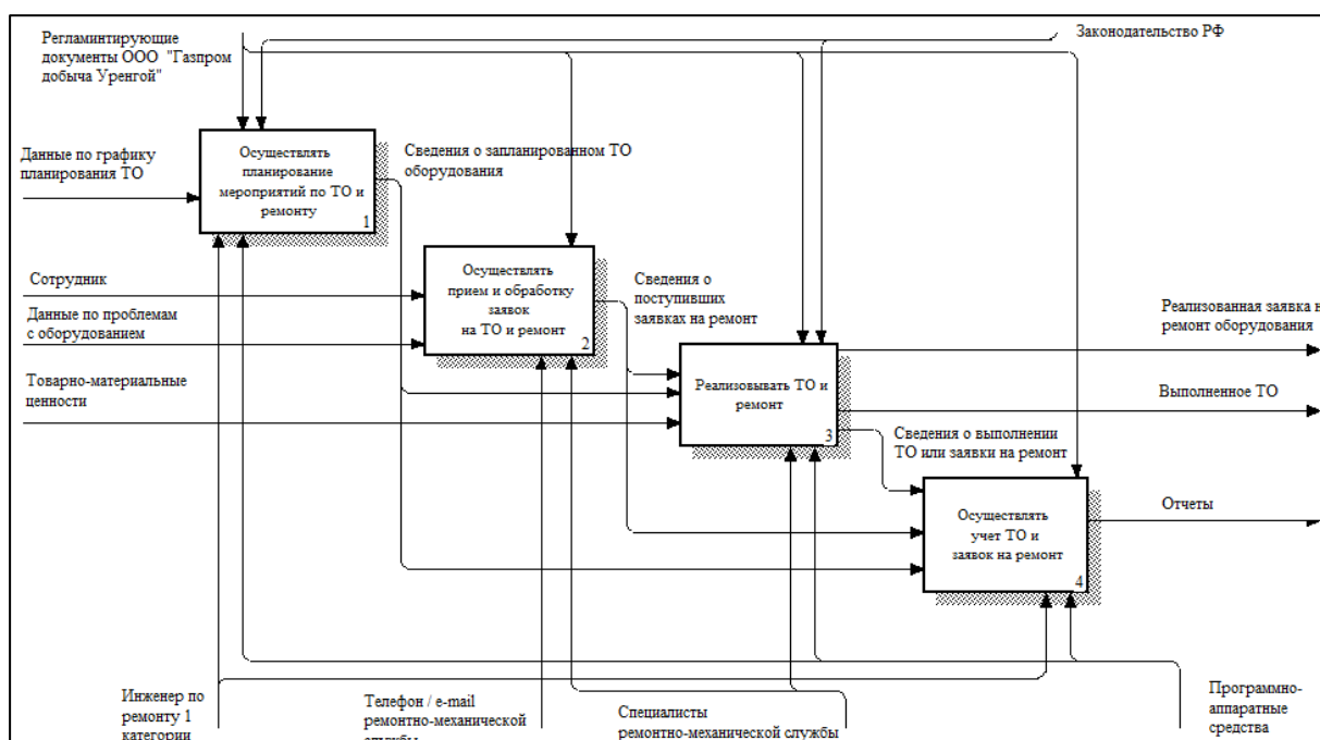
Рисунок 1.2 – Декомпозиция функциональной модели процесса технического обслуживания и ремонта технологического оборудования цеха газоконденсатного промысла
