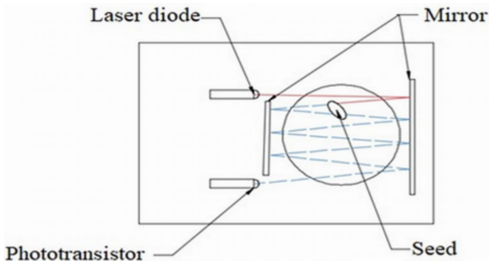
Рисунок 3 – Схема лазерного датчика с многократным отражением светового луча
