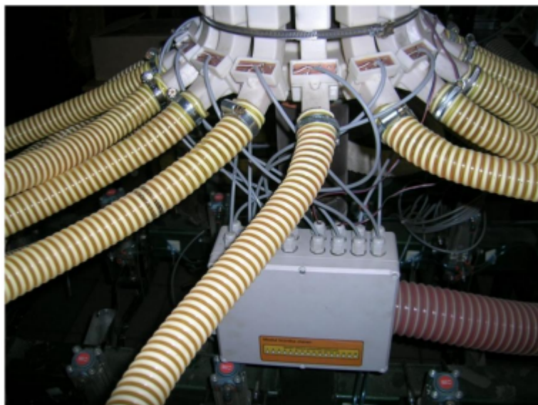
Рисунок 3 – Оригинальная конструкция распределительной головки, интегрированной с датчиками семян в пневматической сеялке
