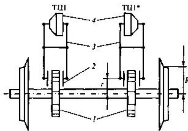
Рисунок 1 - Упрощенная конструкция дискового тормоза
