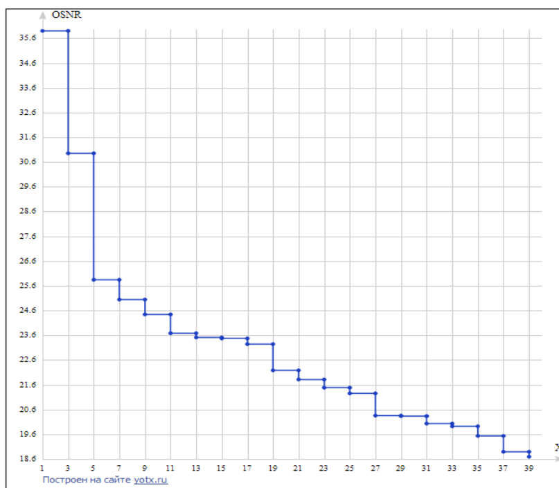
Рис. 2 График OSNR участка г. Якутск – г. Удачный
