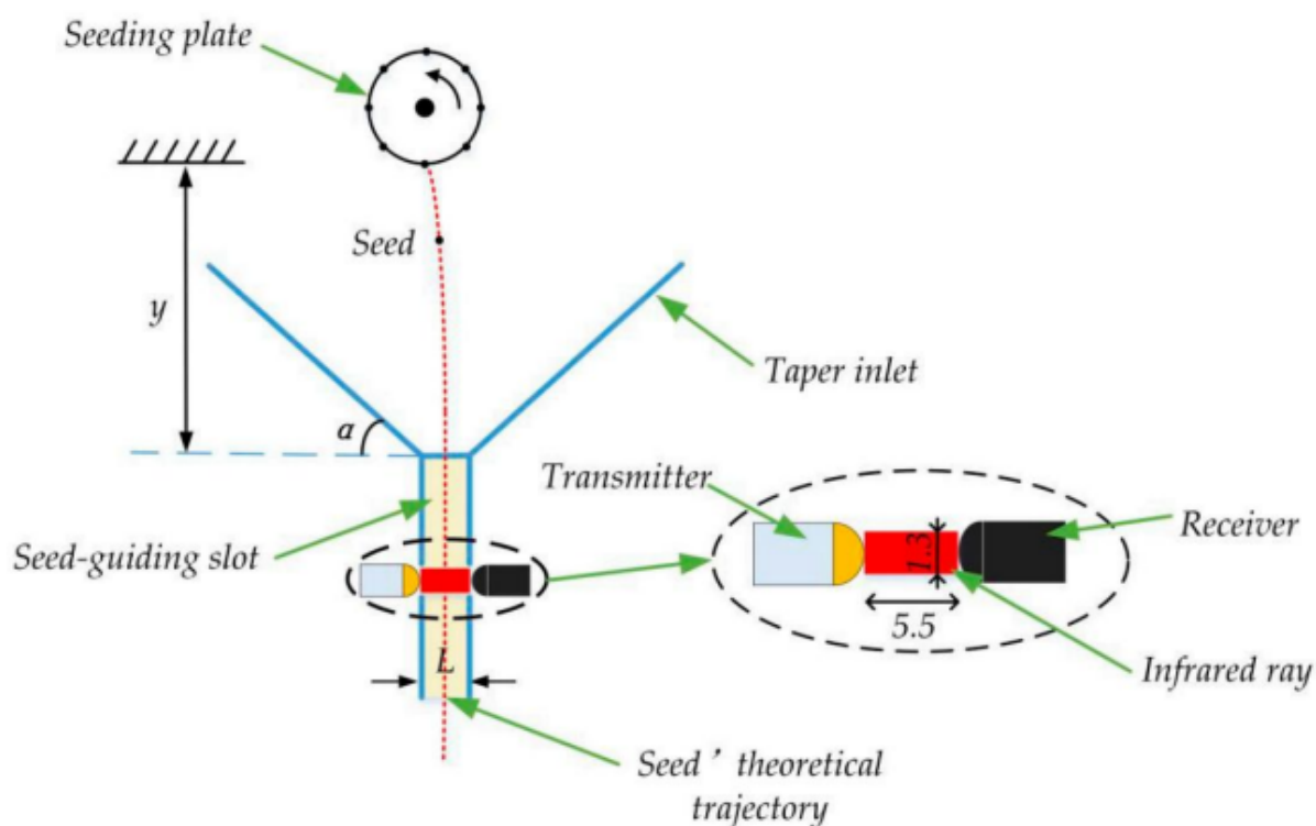
Рисунок 1 – Траектория падения, когда семя падает через направляющую щель. Единицей числа на этом рисунке является мм.
