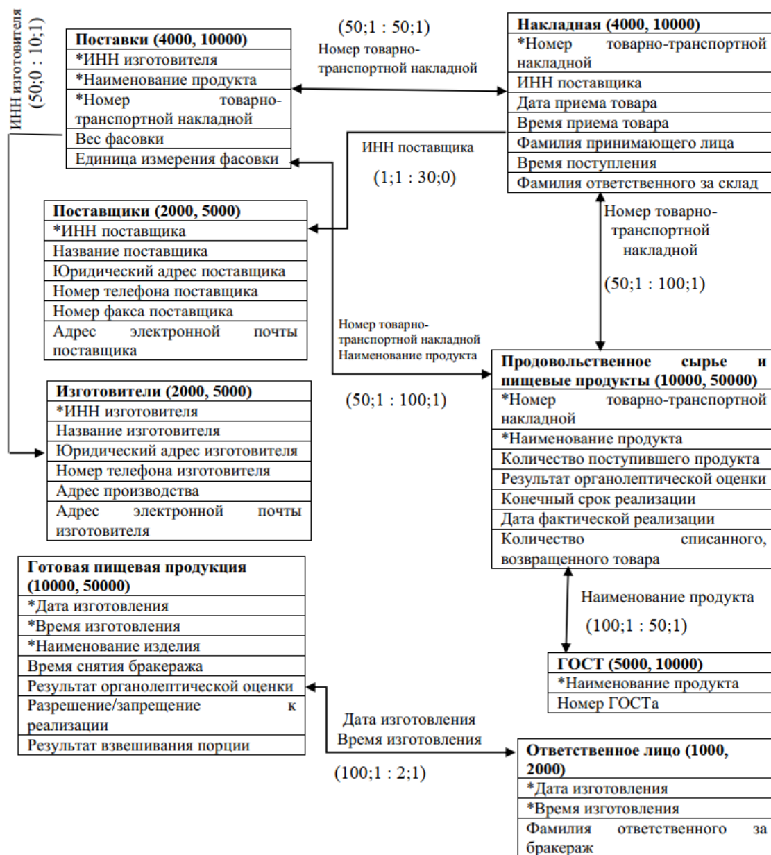
Рис. 2. Схема логической модели базы данных
