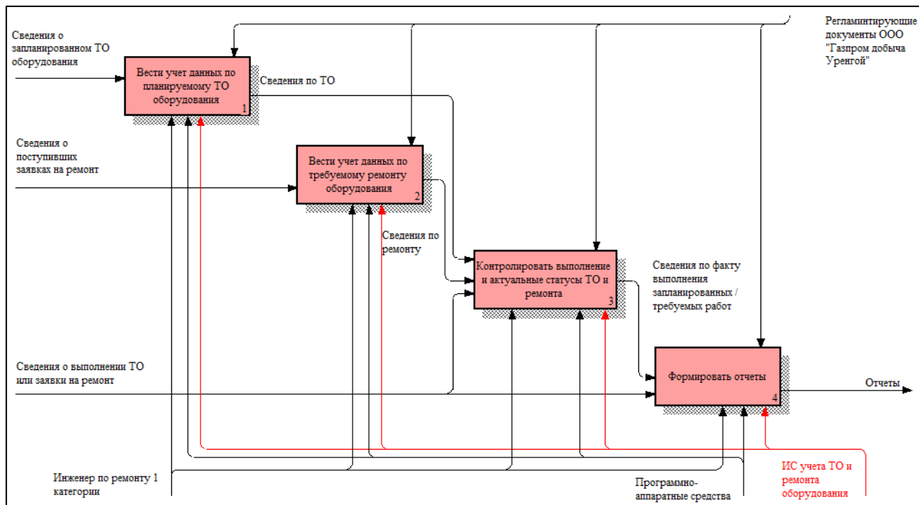
Рисунок 1.5 – Декомпозиция блока учета технического обслуживания и заявок на ремонт технологического оборудования цеха газоконденсатного промысла с учетом автоматизации
