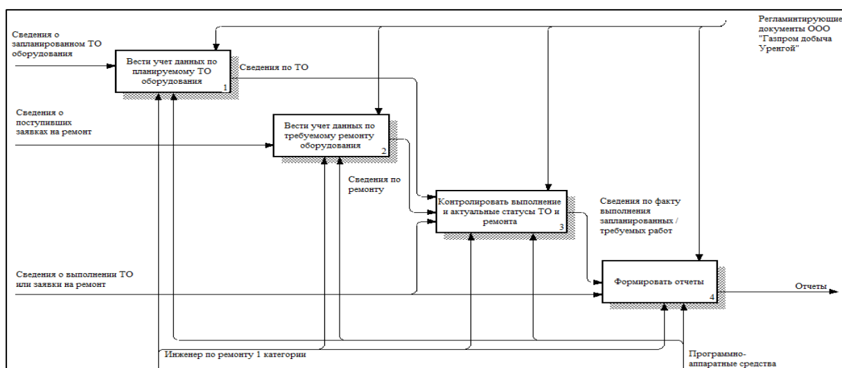
Рисунок 1.3 – Декомпозиция блока учета технического обслуживания и заявок на ремонт технологического оборудования цеха газоконденсатного промысла
