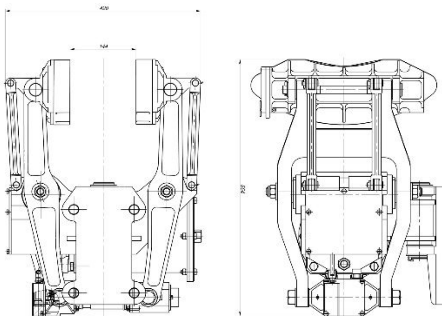
Рисунок 2 – Блок дискового тормоза
