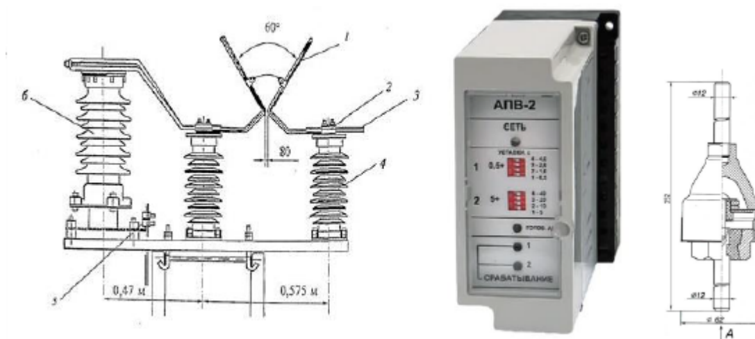
Рисунок 5 – Роговой разрядник с ОПН, АПВ, искровой промежуток
