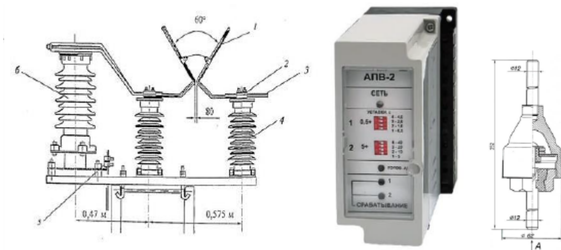
Рисунок 5 – Роговый разрядник с ОПН, АПВ, искровой промежуток
