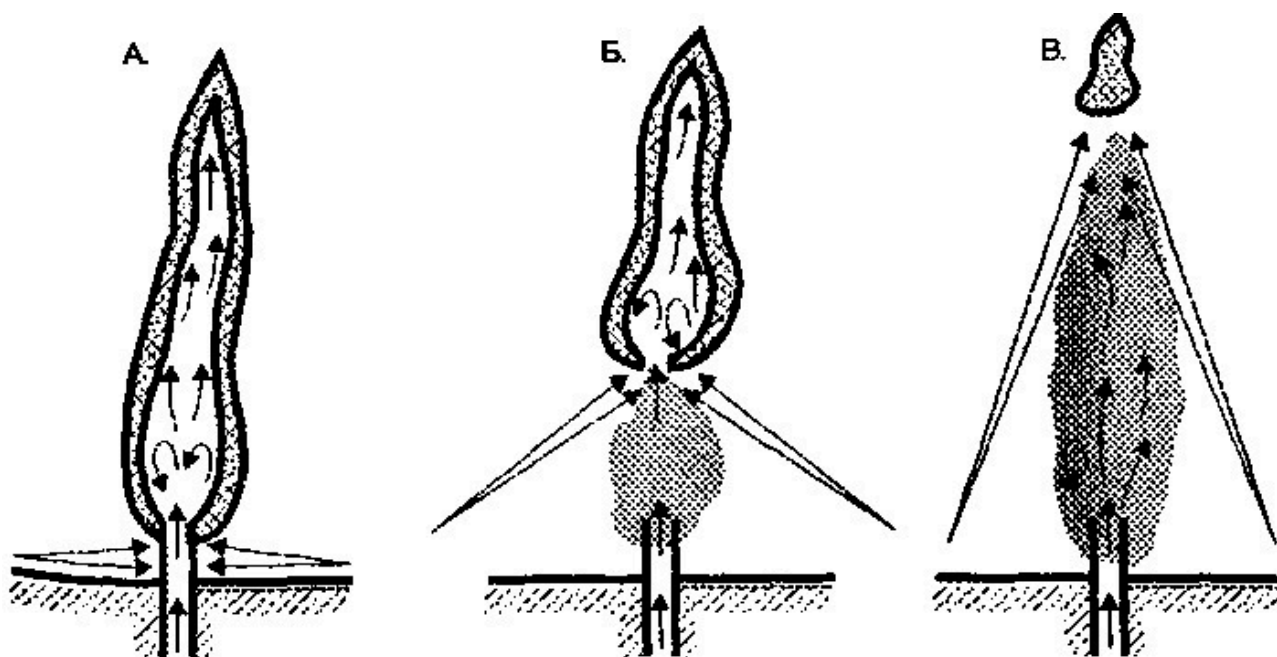
Рисунок 7 – Тушение фонтана способом отрыва пламени от горючего вещества
