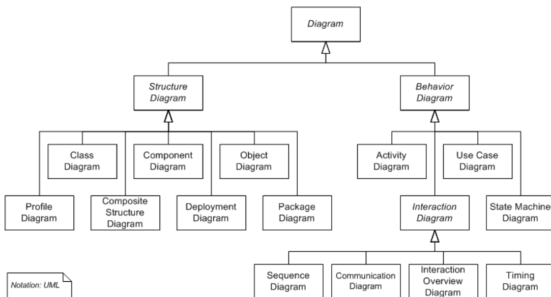
Рисунок 1.3 – Структура диаграмм UML
