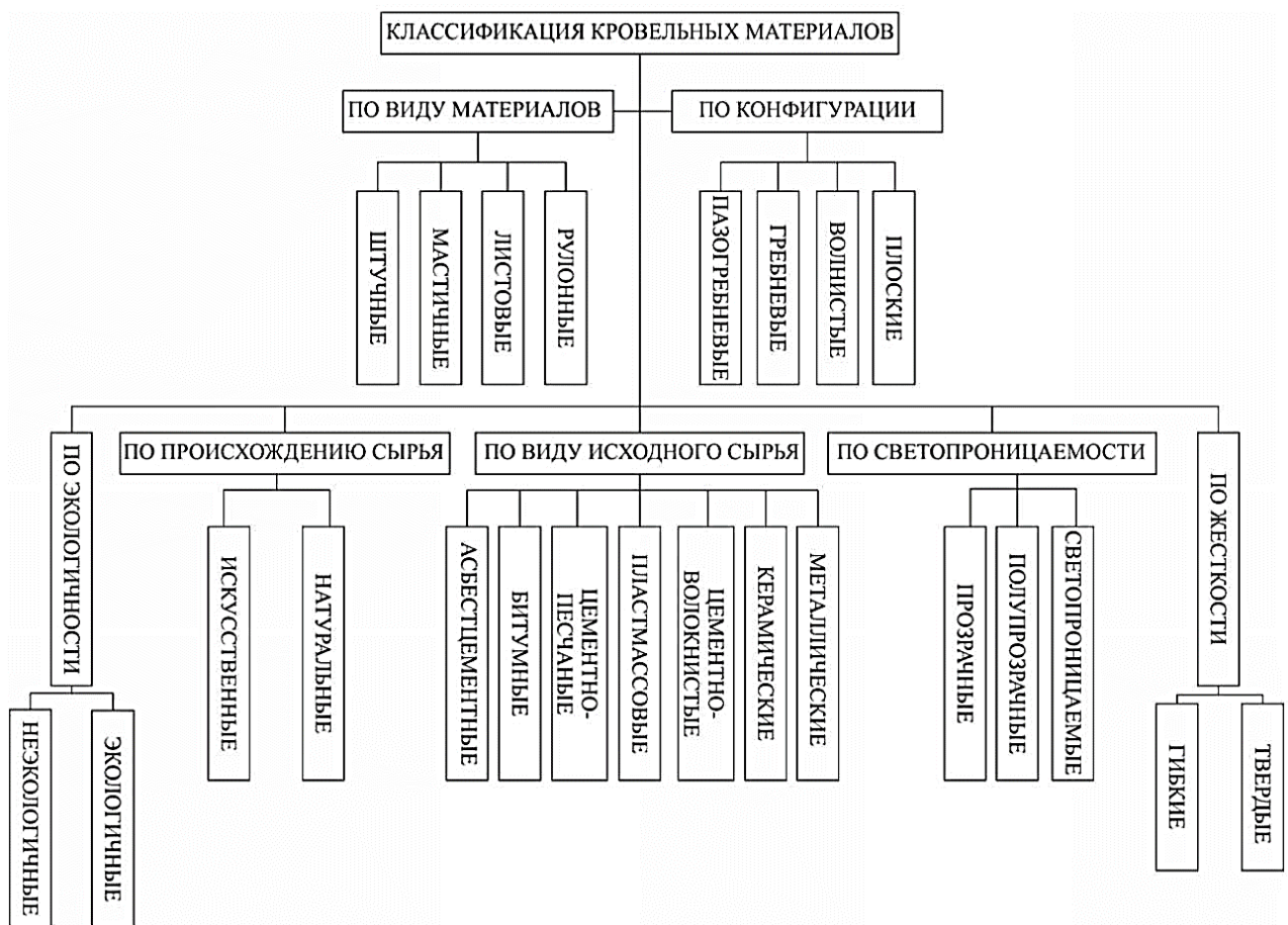
Рисунок 1 - Классификация кровельных материалов
