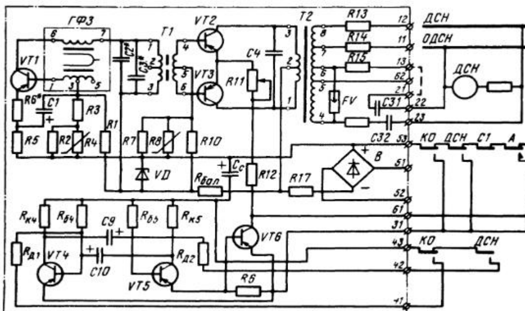
Рисунок 1. Схема генератора ГКШ
