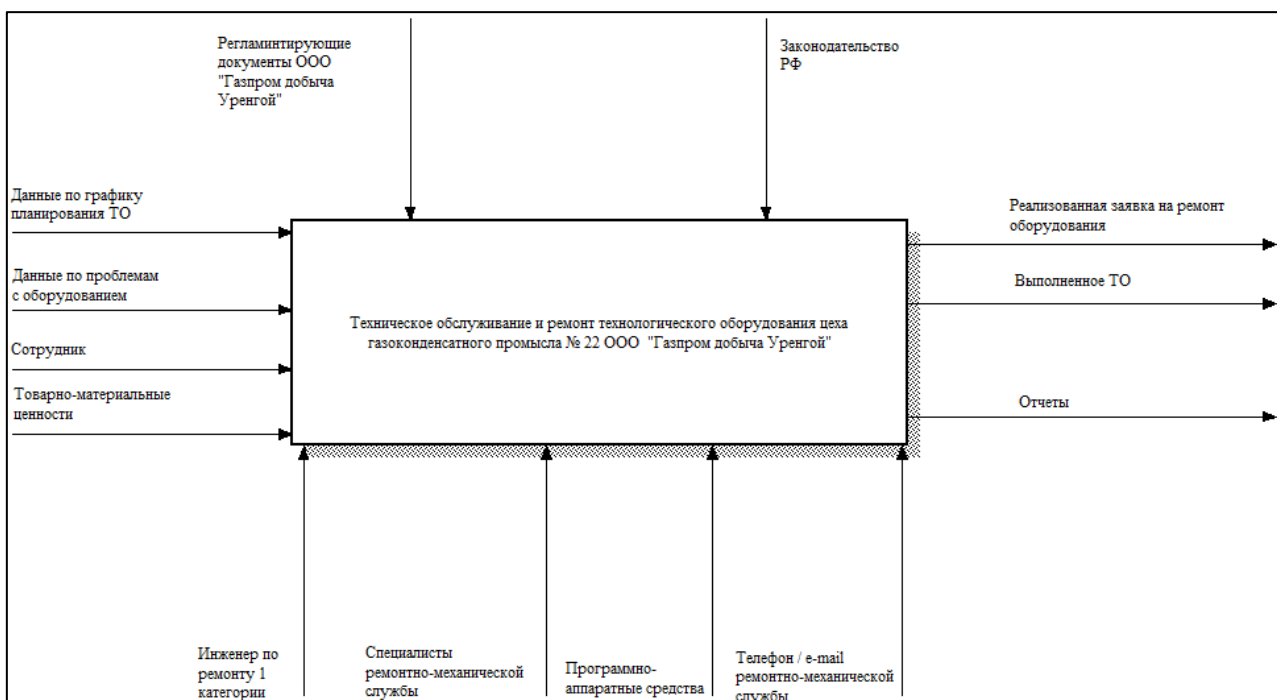
Рисунок 1.1 – Функциональная модель процесса технического обслуживания и ремонта технологического оборудования цеха газоконденсатного промысла
