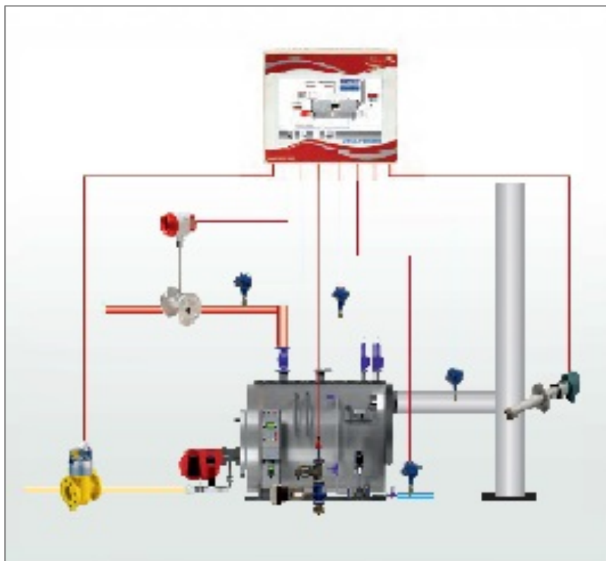
Рис.1 Система мониторинга эффективности котла.
