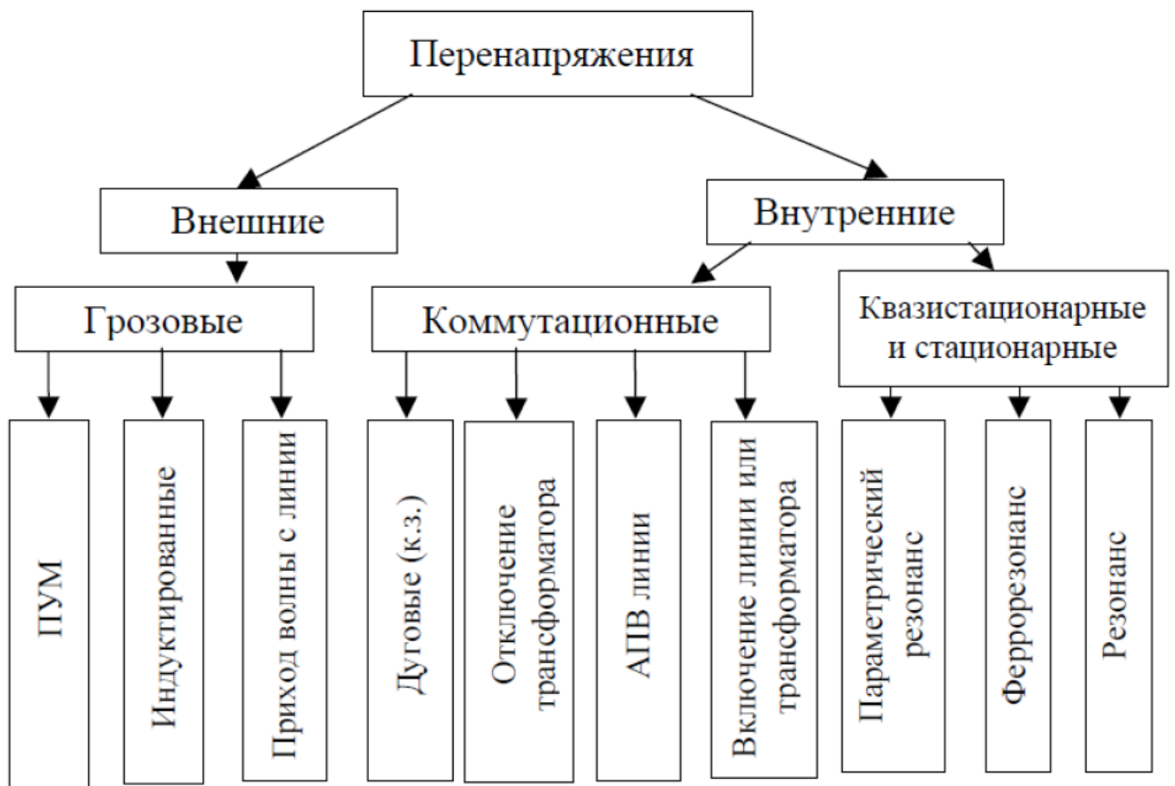
Рисунок 1 – Классификация перенапряжений
