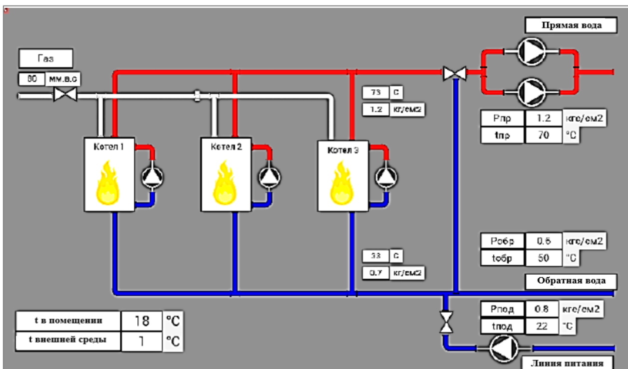
Рис. 2 Мнемосхема модульной котельной.
