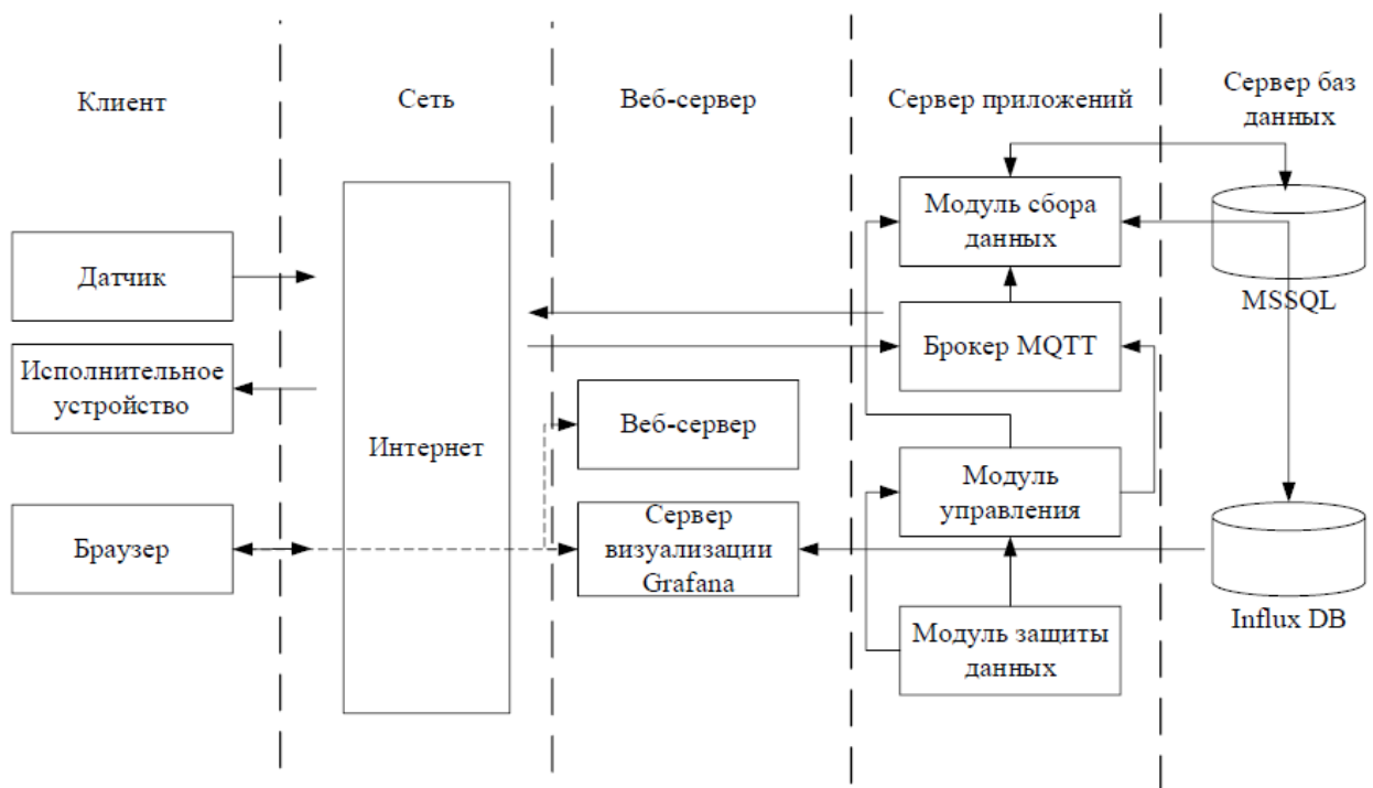
Рисунок 1. Системная архитектура «Умный дом»
