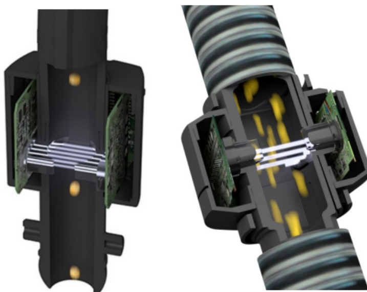
Рисунок 2 – Фотоэлектрический датчик Väderstad.
