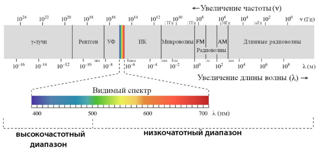
Рисунок 2. Электромагнитный спектр
