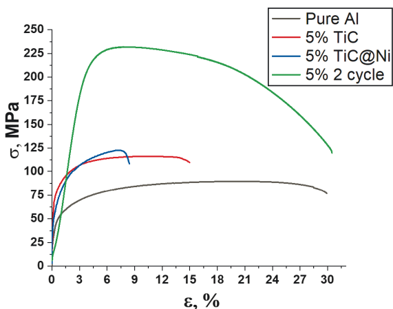
Рис. 4. Кривые деформирования образцов Al, 5% TiC, 5% TiC@Ni и 5% ALD (2 цикла)
