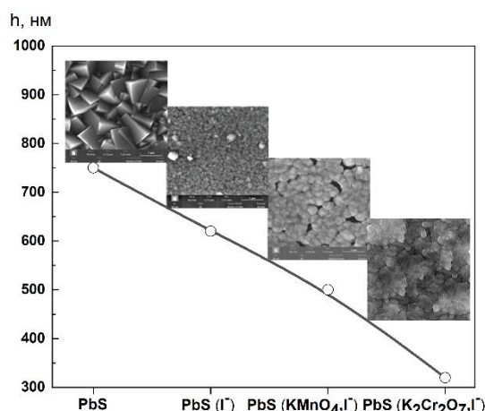
Рис. 1. Толщина пленок PbS, PbS(I), PbS(I,KmnO 4 ), PbS(I,K 2 Cr 2 O 7 ), химически осажденных при 353 К в течение 90 мин на стеклянных подложках
