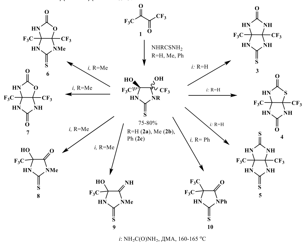
Схема 1. Реакции тиоксоимидазолидинов 2a-c с мочевиной.
