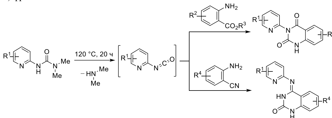
Схема 1. Взаимодействие N,N -диметил- N' -(пиридин-2-ил)мочевин с замещёнными эфирами и нитрилами антралиловых кислот.
