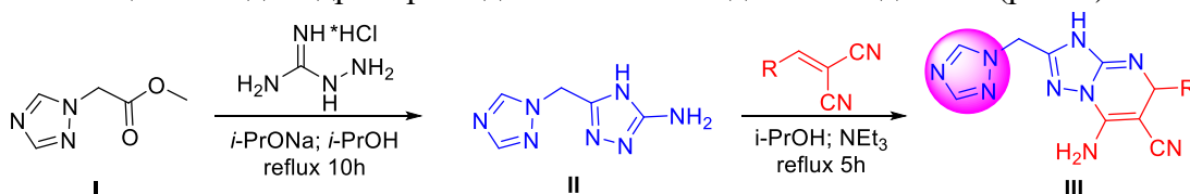
Рис. 2. Получение 2-((1,2,4-триазол-1-ил)метил)-7-амино-5-замещенных-3,5-дигидро-[1,2,4]триазоло[1,5-а]пиримидин-6-карбонитрилов
