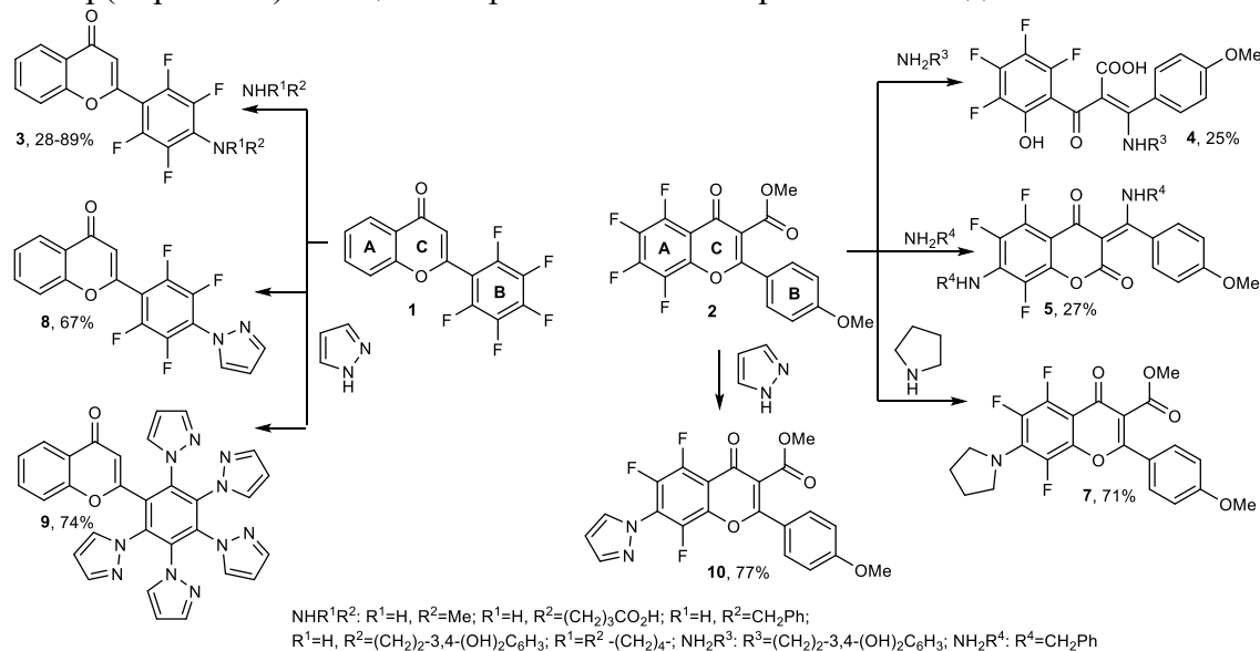
Схема 1. Реакции полифторсодержащих флавонов 1 , 2 с аминами
