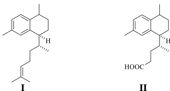
Рис. 1. Структура эргорджина (I) и DMNP (II)
