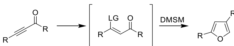
Схема 1. Предлагаемый подход
