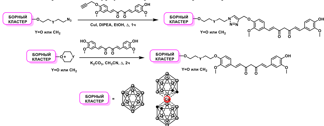
Рис. 2. Синтез конъюгатов куркумина с полиэдрическими гидридами бора.
