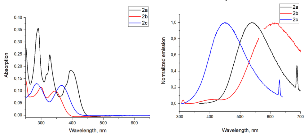
Рис. 2. Спектры поглощения (слева) и эмиссии (справа) для соединений 2a-c в MeCN
