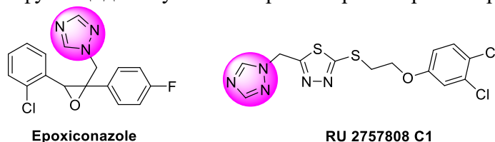
Рис. 1. Противогрибковые препараты
