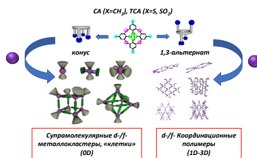
Рис. 1. Кристаллические супрамолекулярные координационные соединения на основе (тиа)каликс[4]аренов (CA, TCA).
