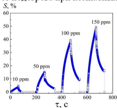
Рис. 1. Кинетическая зависимость величины отклика плёнки Cd_xPb_{1-x}S полученной при 0.02 моль/л хлорида кадмия при изменении концентрации аммиака от 10 до 150 ppm (7.08-106.19 мг/м 3 ) в воздушной среде
