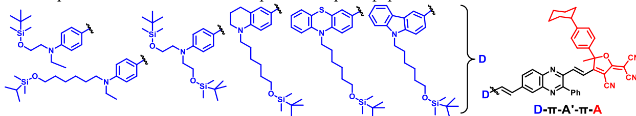
Рис. 1. Исследуемые D-π-A'-π-A хромофоры: \lambda_{\max} 536-665 нм, \beta 474-937 \times 10^{-30} ед. СГСЭ (M06-2X/aug-cc-pVDZ/B3LYP/6-31G*), термическая стабильность T_d 171-270 °C (ДСК), d_{33} = 23-52 пм/В (генерация второй гармоники, фемтосекундный лазер с \lambda 1028 нм).
