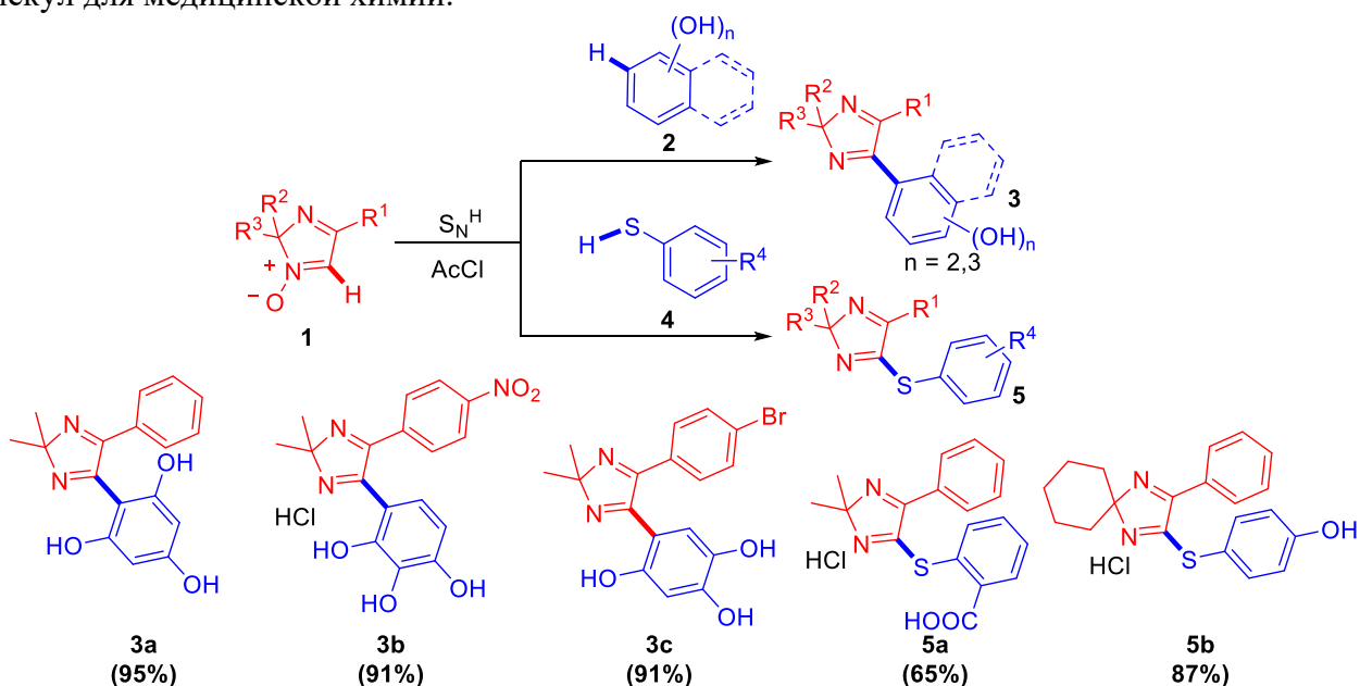
Схема 1. C-Н функционализация 2H-имидазол N-оксидов (тио)фенолами
