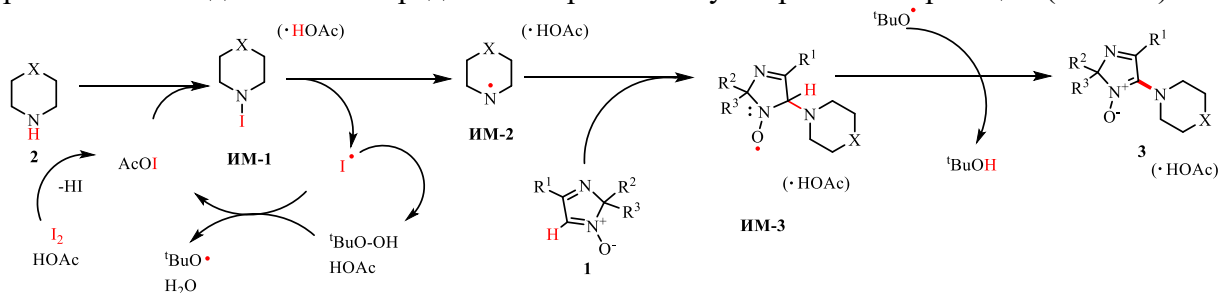
Схема 2. Предполагаемый механизм реакции.
