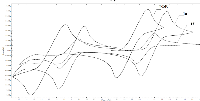
Рис. 1. Циклические вольтамперограммы вердазилов 1a,f и ТФВ .
