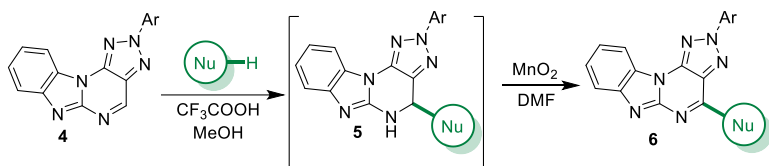
Схема 2. C8-функционализация бензимидазоазапуринов
