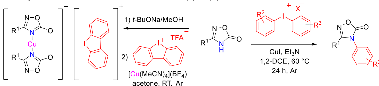
Рис. 1. Взаимодействие 1,2,4-оксадиазолонов с иодониевыми и иодолиевыми солями.
