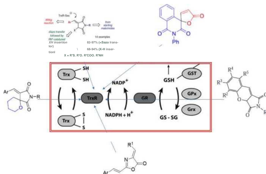
Схема 1. Ингибиторы тиоредоксин редуктазы на основе электрон-дефицитных олефинов
