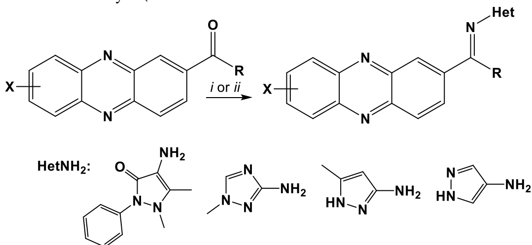
Рис. 1. Реагенты и условия: i) \text{NH}_2\text{Het} , n -ТСК, толуол; ii) \text{NH}_2\text{Het} , \text{CF}_3\text{CO}_2\text{H} , 500 об/мин, 1 час. Биологическое действие полученных конъюгатов исследуется.
