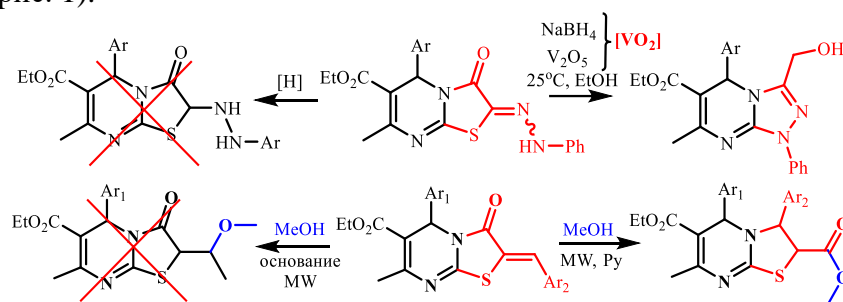
Рис. 1. Новые перегруппировки в ряду тиазоло[3,2-а]пиримидинов.
