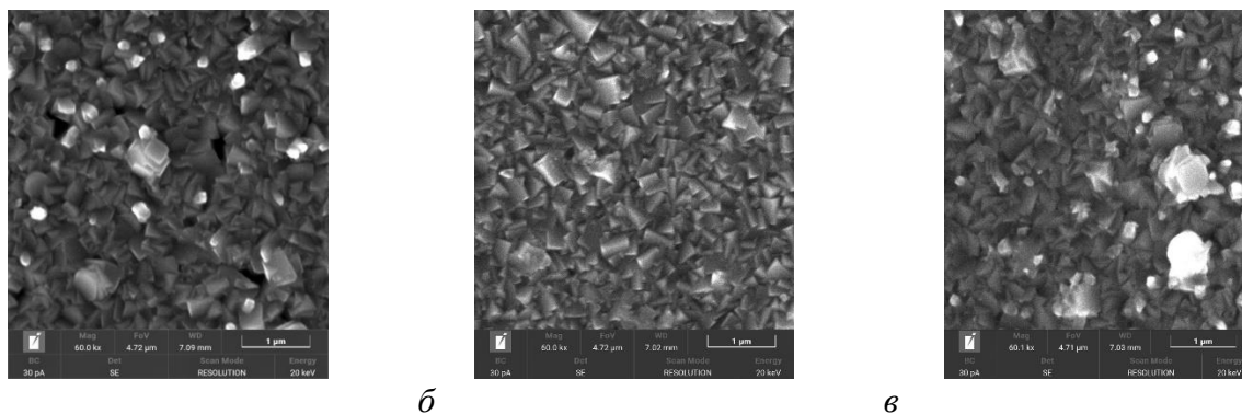
Рис. 1. Микроизображения слоев PbS(MnCl 2 ,I) в зависимости длительности активации подложки, мин: 10 (а) 20 (б), 30 (в)
