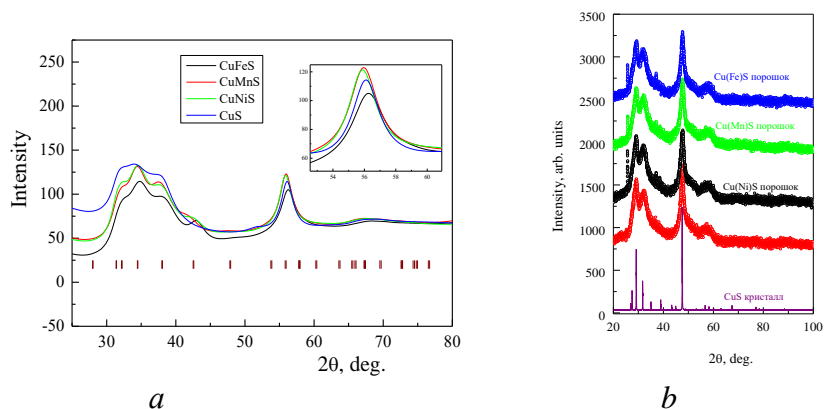
Рис. 1. Экспериментальные рентгенограммы пленок (а) и порошков (б) CuS и CuS(Mn, Ni, Fe). Во вставке показан рефлекс (110).
