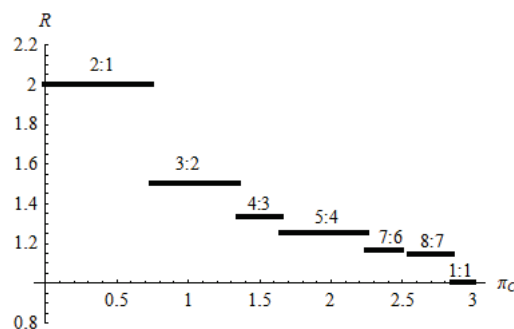
Рисунок 1. Синхронные режимы колебаний двух электрически связанных нейронов
